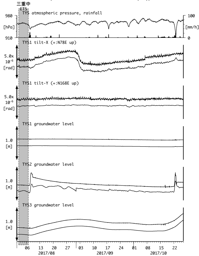
図3: Tilt and groundwater level changes at TYS 豊田神殿 (時間値) (2017/08/01 00:00 - 2017/10/27 00:00 (JST))
