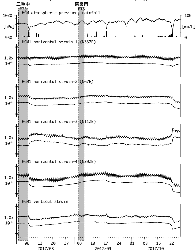
図17 : Crustal strains changes at HGM 田辺本宮 (時間値) (2017/08/01 00:00 - 2017/10/27 00:00 (JST))
