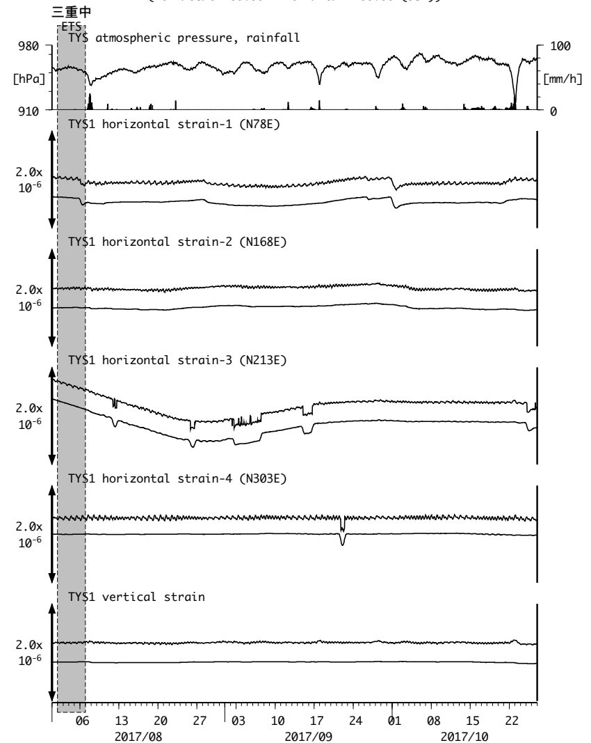
図2: Crustal strains changes at TYS 豊田神殿 (時間値) (2017/08/01 00:00 - 2017/10/27 00:00 (JST))
