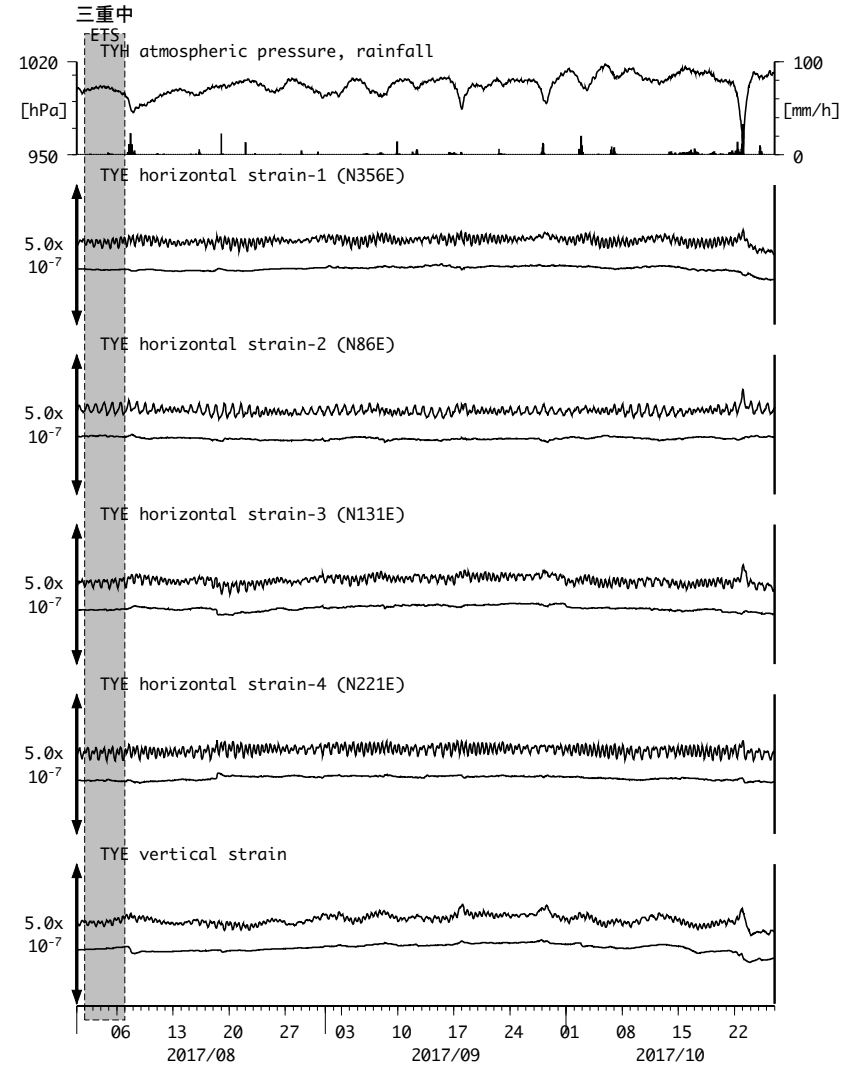
図6: Crustal strain changes at TYE 豊橋多米 (時間値) (2017/08/01 00:00 - 2017/10/27 00:00 (JST))
