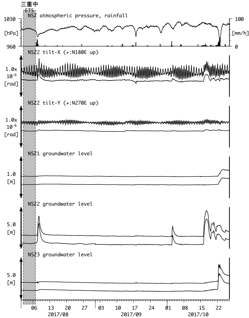
図5: Tilt and groundwater level changes at NSZ 西尾善明 (時間値) (2017/08/01 00:00 - 2017/10/27 00:00 (JST))
