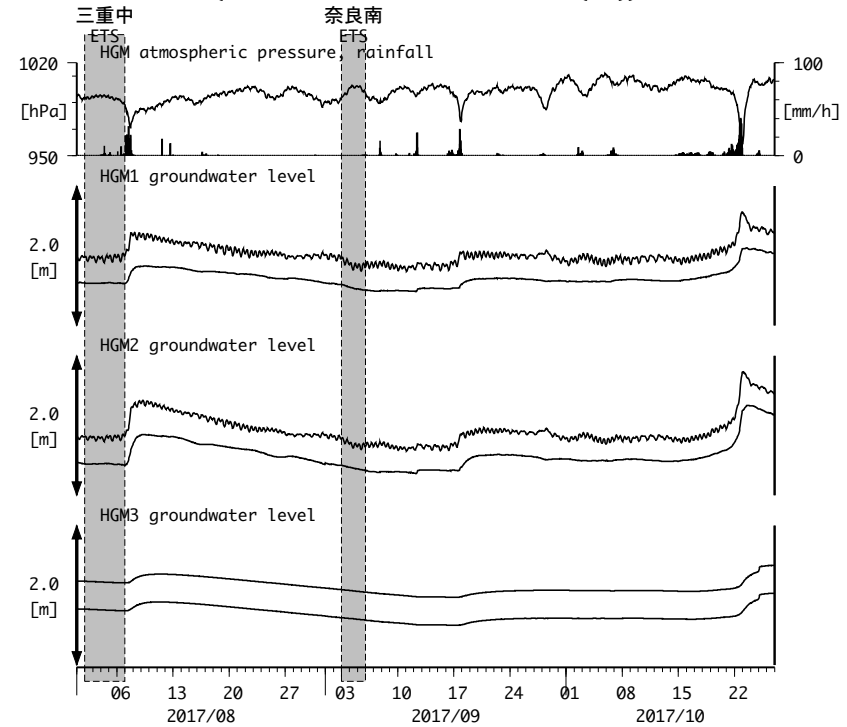
図18 : Groundwater level changes at HGM 田辺本宮 (時間値) (2017/08/01 00:00 - 2017/10/27 00:00 (JST))
