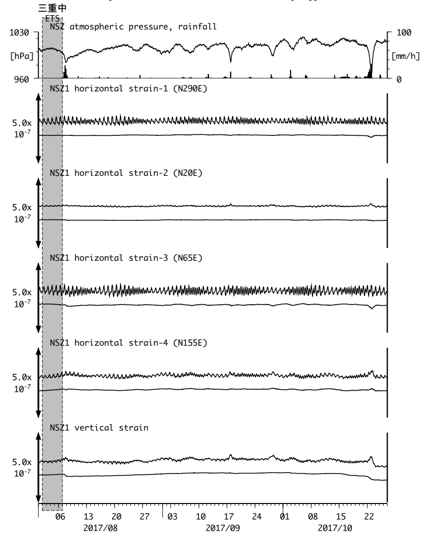
図4: Crustal strains changes at NSZ 西尾善明 (時間値) (2017/08/01 00:00 - 2017/10/27 00:00 (JST))
