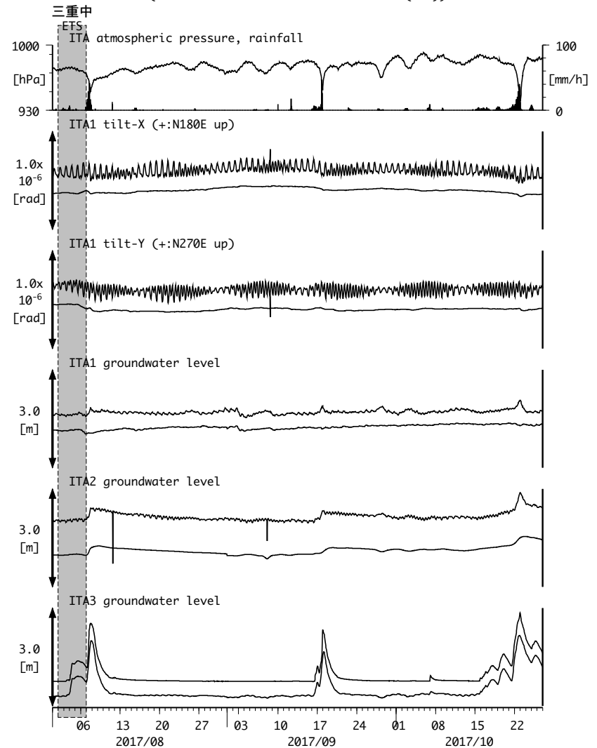
図12: Tilt and groundwater level changes at ITA 松阪飯高 (時間値) (2017/08/01 00:00 - 2017/10/27 00:00 (JST))
