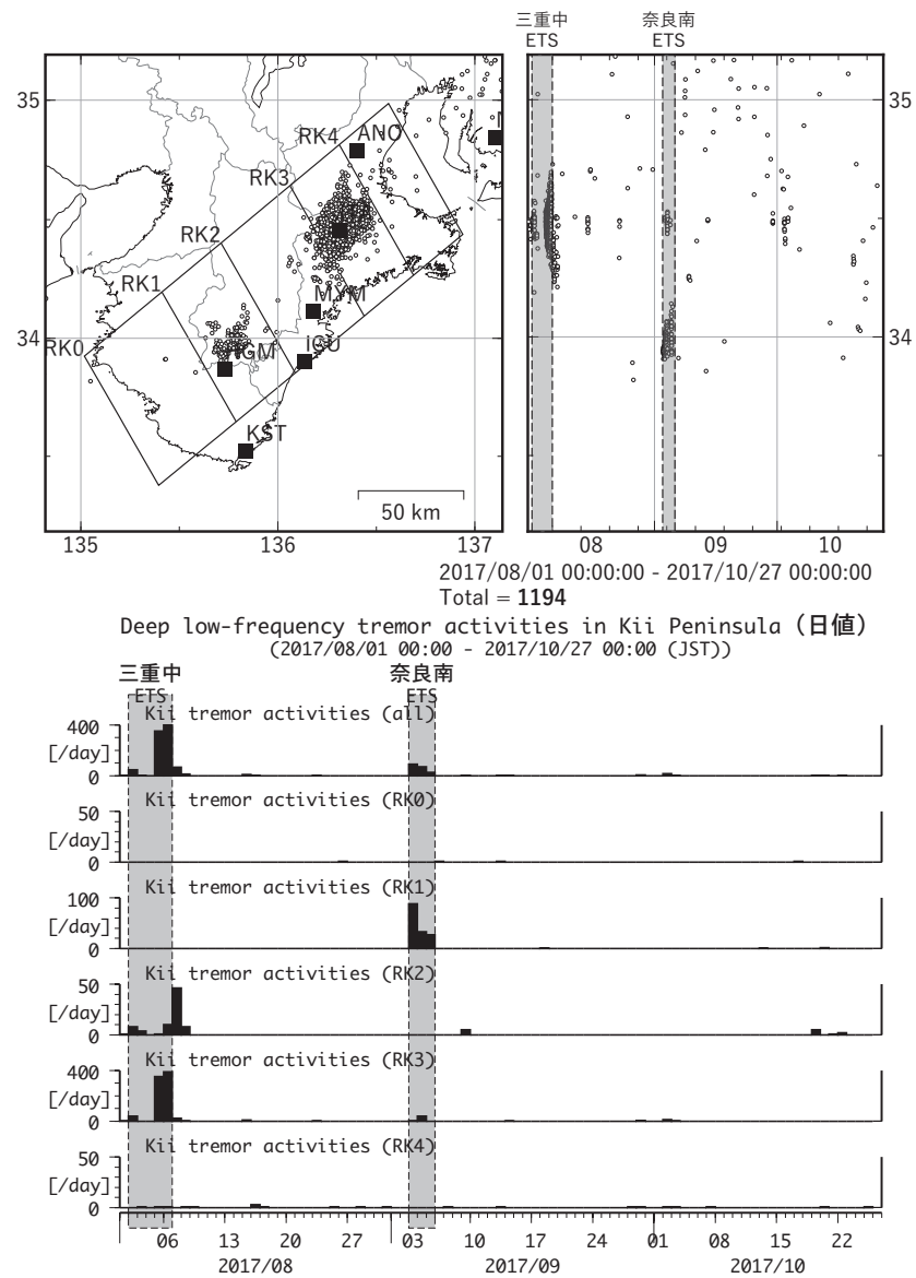
図23 (上段) 紀伊半島における深部低周波微動の時空間分布, (下段) 各領域における発生頻度 (日値)。
