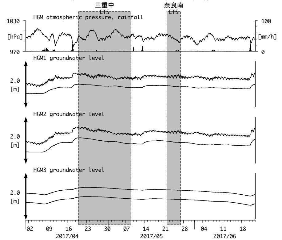
図18: Groundwater level changes at HGM 田辺本宮 (時間値) (2017/04/01 00:00 - 2017/06/23 00:00 (JST))
