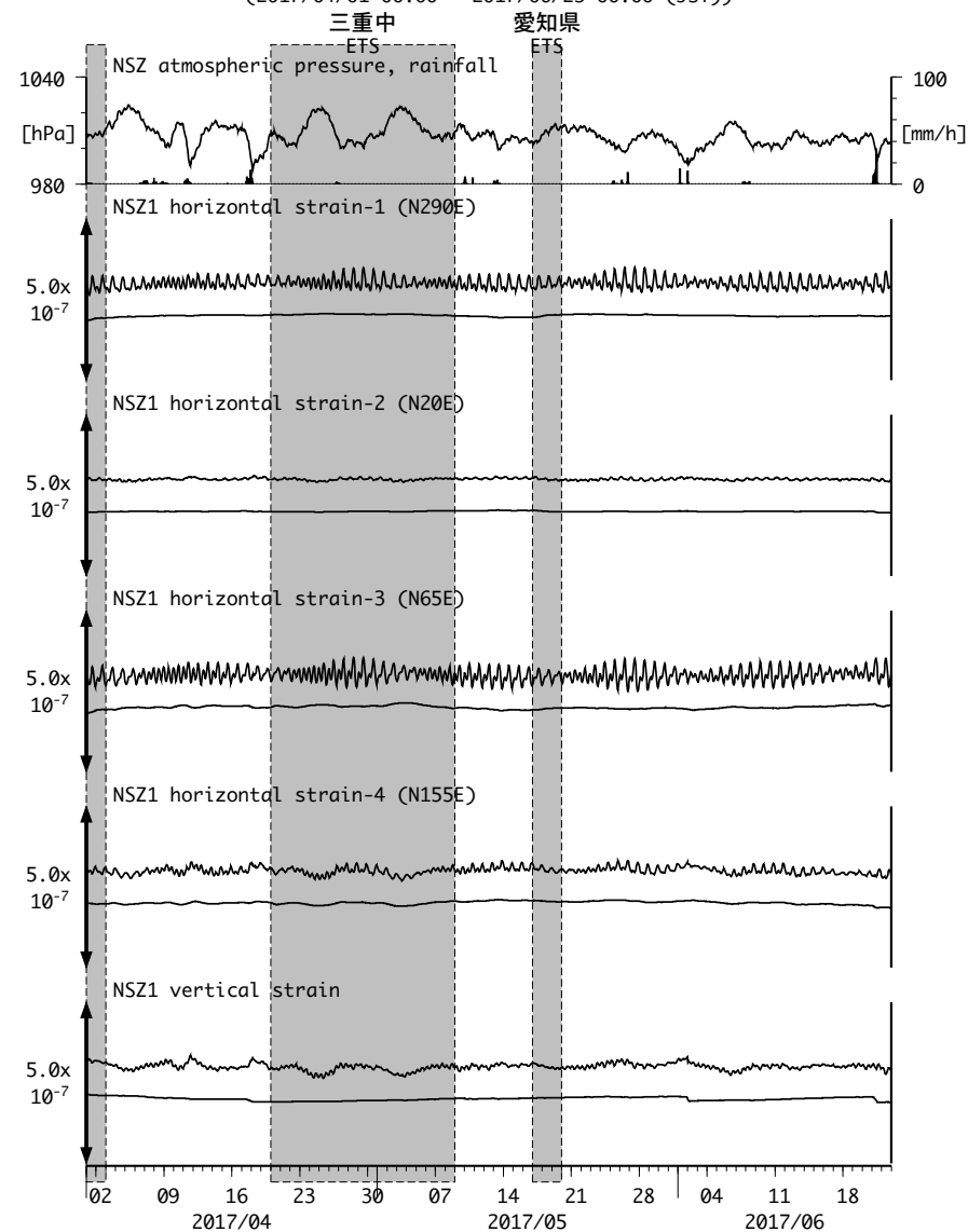
図4: Crustal strains changes at NSZ 西尾善明 (時間値) (2017/04/01 00:00 - 2017/06/23 00:00 (JST))
