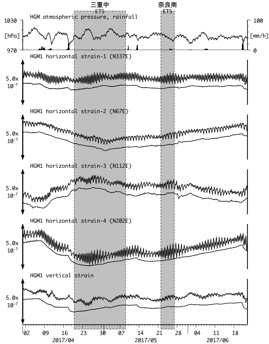
図17: Crustal strains changes at HGM 田辺本宮 (時間値) (2017/04/01 00:00 - 2017/06/23 00:00 (JST))
