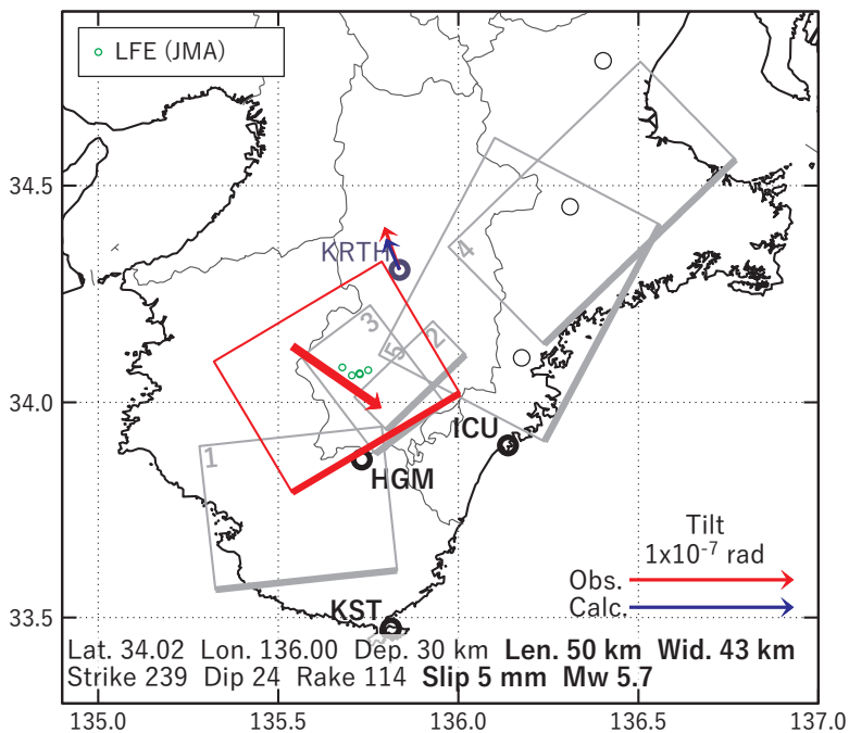
図26 2017/5/22-26の歪・傾斜変化（図25[A]）を説明する断層モデル。
