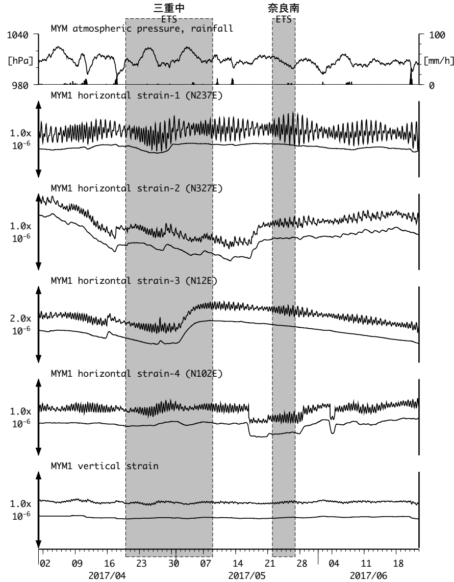
図13: Crustal strain changes at MYM 紀北海山 (時間値) (2017/04/01 00:00 - 2017/06/23 00:00 (JST))
