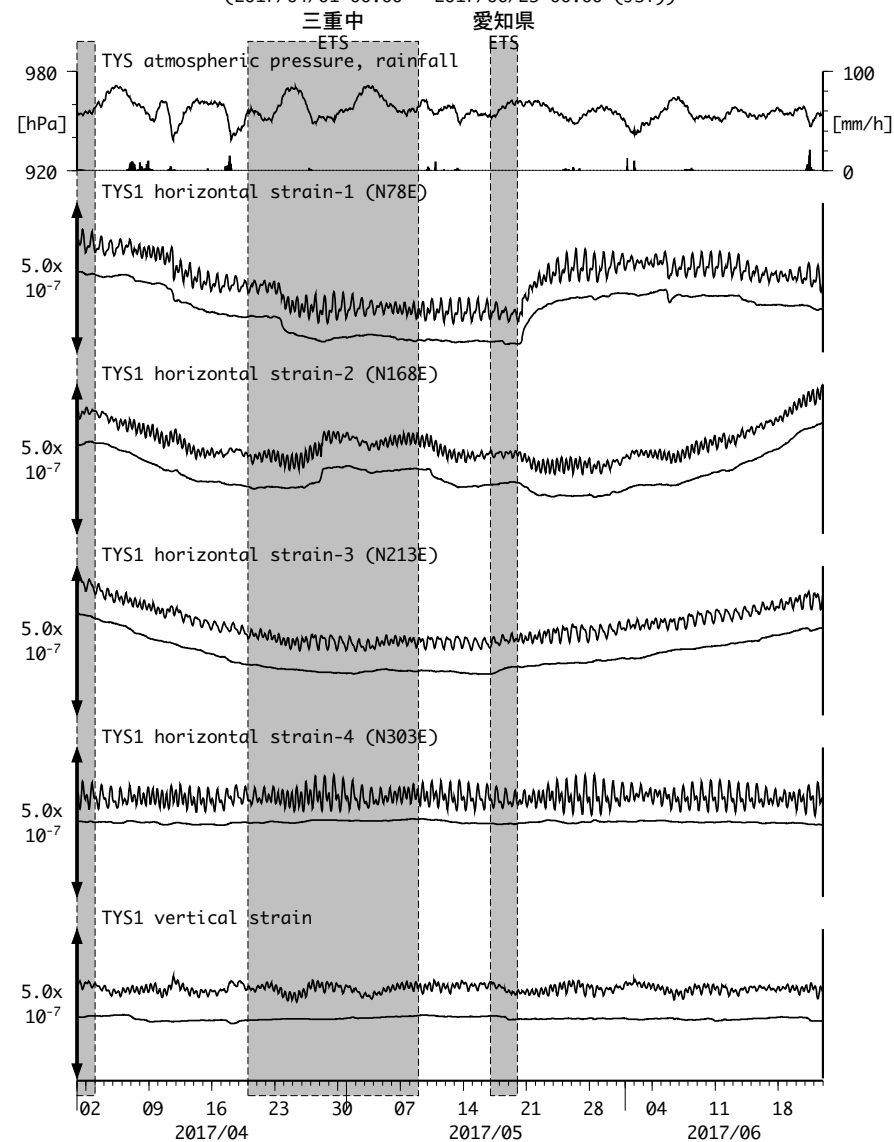
図2: Crustal strains changes at TYS 豊田神殿 (時間値) (2017/04/01 00:00 - 2017/06/23 00:00 (JST))
