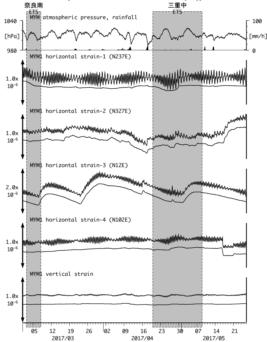
図13: Crustal strain changes at MYM 紀北海山 (時間値) (2017/03/01 00:00 - 2017/05/26 00:00 (JST))
