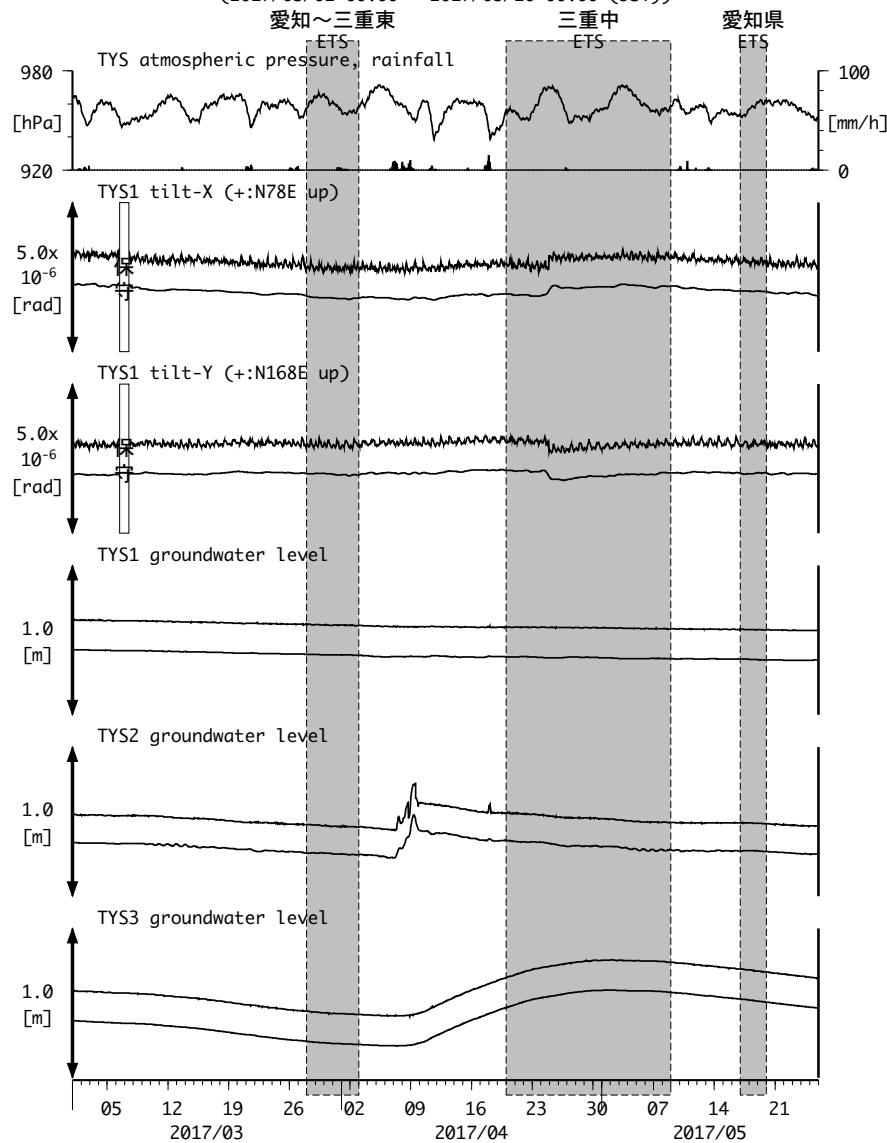
図3: Tilt and groundwater level changes at TYS 豊田神殿 (時間値) (2017/03/01 00:00 - 2017/05/26 00:00 (JST))
