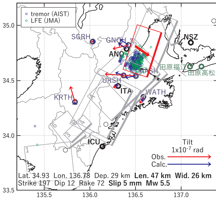
図28 2017/5/4-8の歪・傾斜・地下水変化（図25[C]）を説明する断層モデル。
