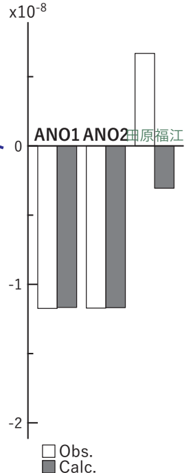
図28 2017/5/4-8の歪・傾斜・地下水変化（図25[C]）を説明する断層モデル。
