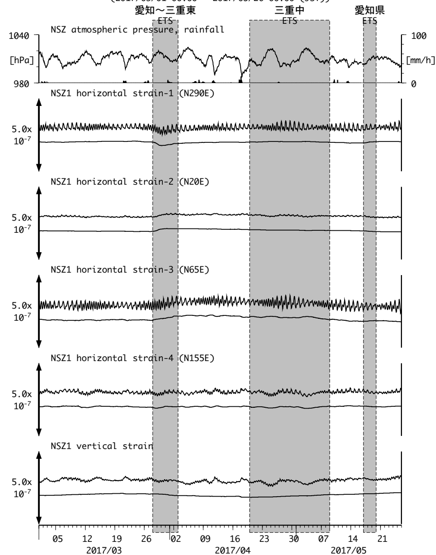
図4: Crustal strains changes at NSZ 西尾善明 (時間値) (2017/03/01 00:00 - 2017/05/26 00:00 (JST))
