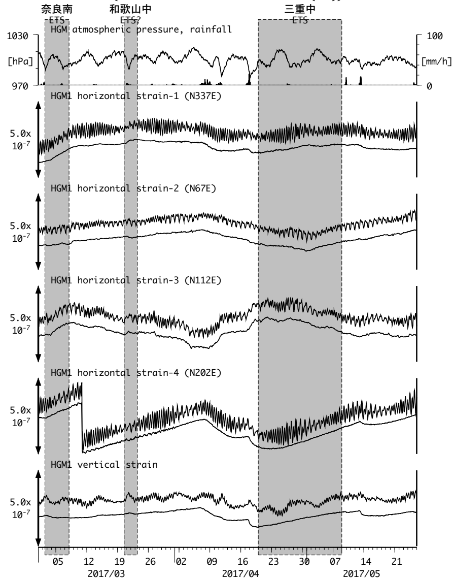
図17: Crustal strains changes at HGM 田辺本宮 (時間値) (2017/03/01 00:00 - 2017/05/26 00:00 (JST))
