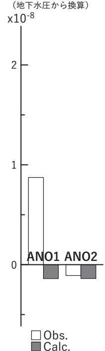
図27 2017/4/25PM-30の歪・傾斜・地下水変化（図25[B]）を説明する断層モデル。
