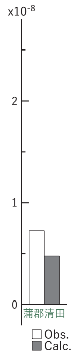
(b3) 体積歪
