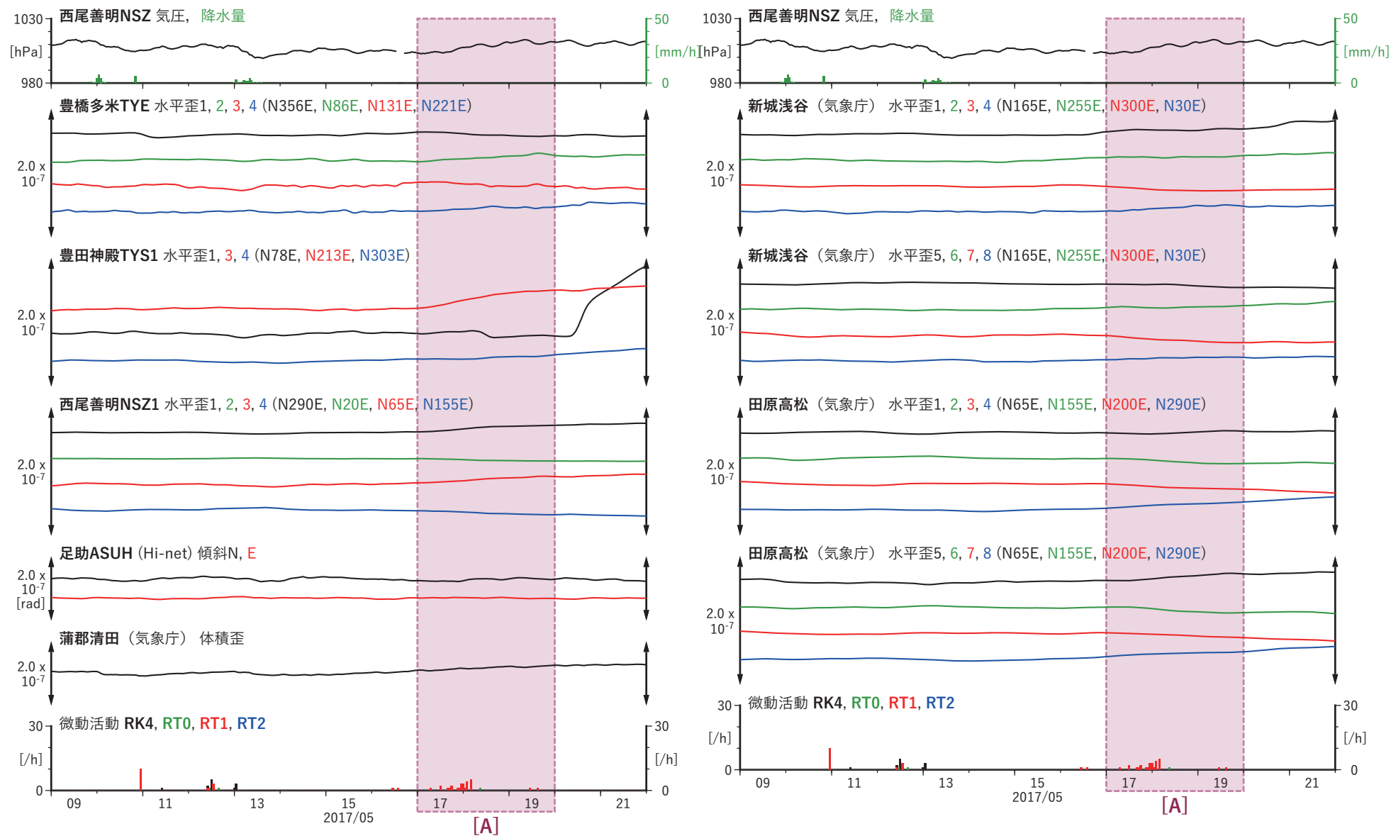
図30 東海地方における歪・傾斜観測結果 (2017/5/9 0:00 - 2017/5/22 0:00 (JST))
