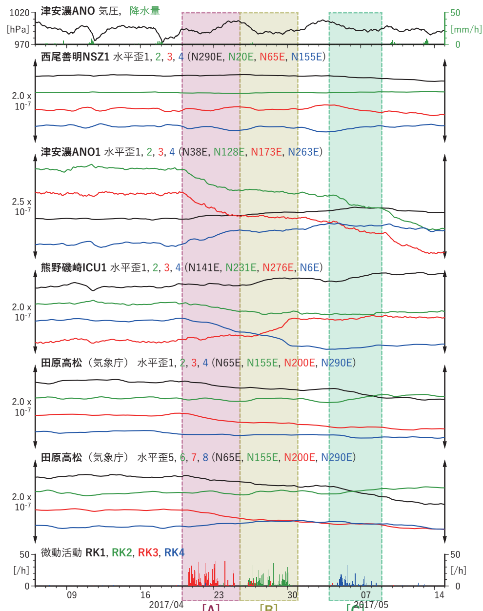
図25 東海地方・紀伊半島における歪・傾斜・地下水観測結果 (2017/4/6 0:00 - 2017/5/15 0:00 (JST))
