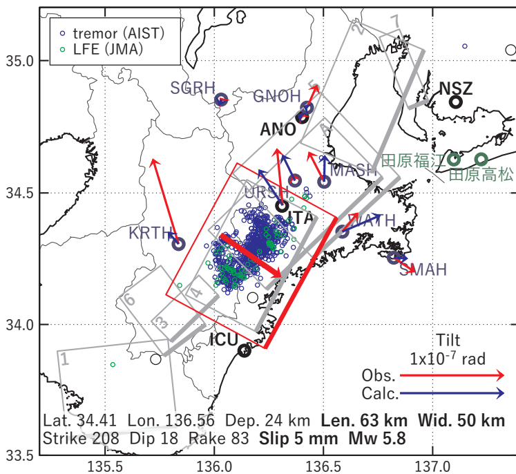
図27 2017/4/25PM-30の歪・傾斜・地下水変化（図25[B]）を説明する断層モデル。
