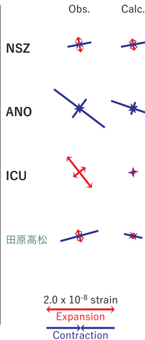
図28 2017/5/4-8の歪・傾斜・地下水変化（図25[C]）を説明する断層モデル。
