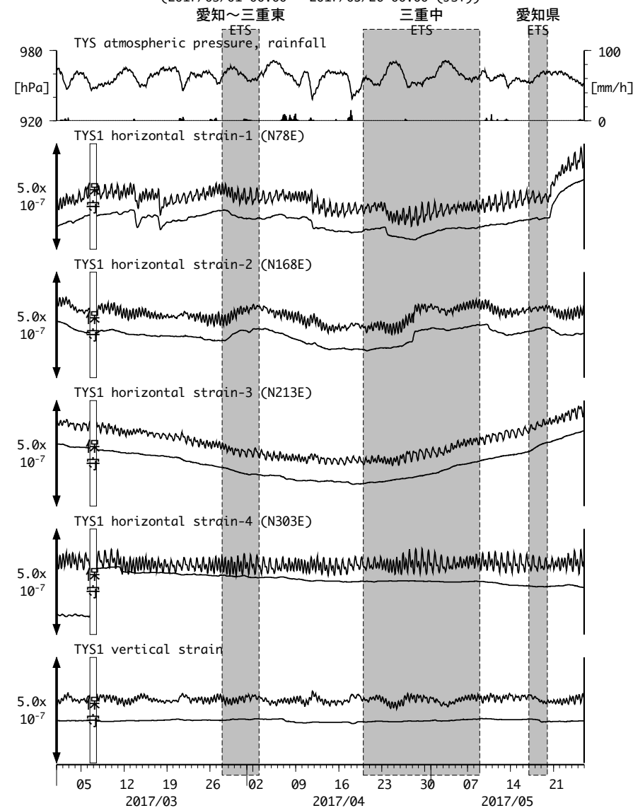
図2: Crustal strains changes at TYS 豊田神殿 (時間値) (2017/03/01 00:00 - 2017/05/26 00:00 (JST))
