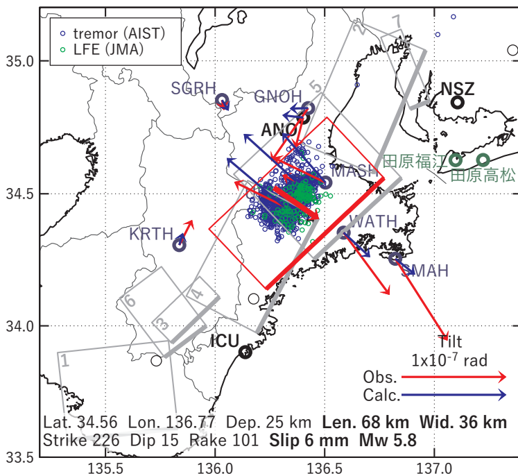
図26 2017/4/20-25AMの歪・傾斜・地下水変化（図25[A]）を説明する断層モデル。
