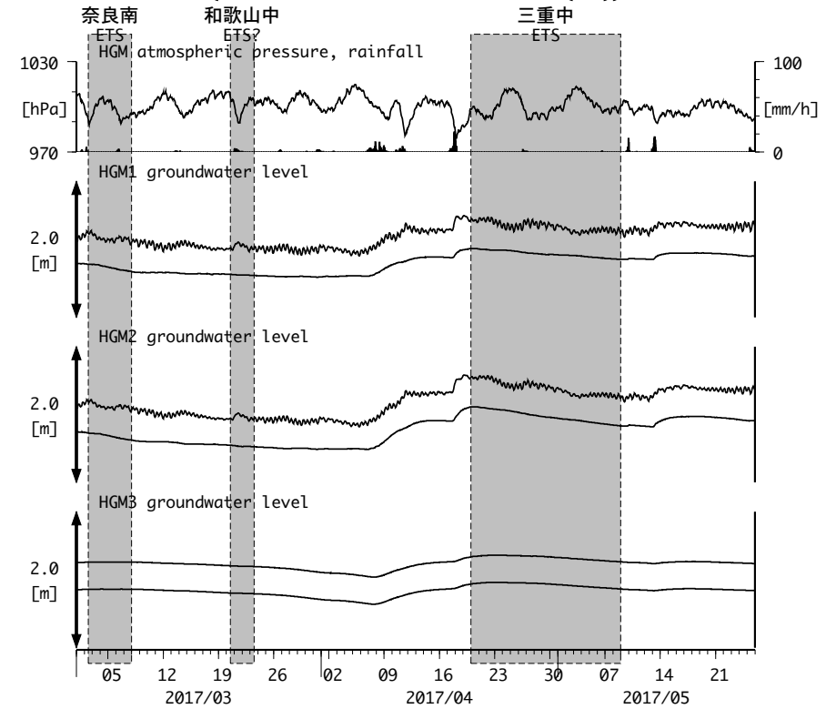
図18: Groundwater level changes at HGM 田辺本宮 (時間値) (2017/03/01 00:00 - 2017/05/26 00:00 (JST))
