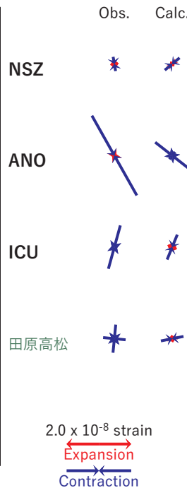
図26 2017/4/20-25AMの歪・傾斜・地下水変化（図25[A]）を説明する断層モデル。
