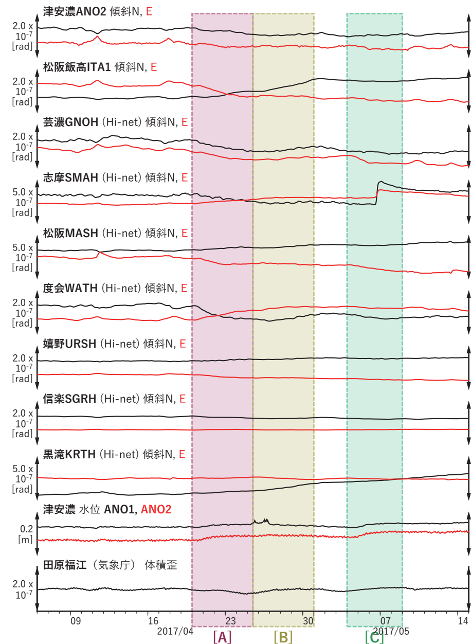
図25 東海地方・紀伊半島における歪・傾斜・地下水観測結果 (2017/4/6 0:00 - 2017/5/15 0:00 (JST))
