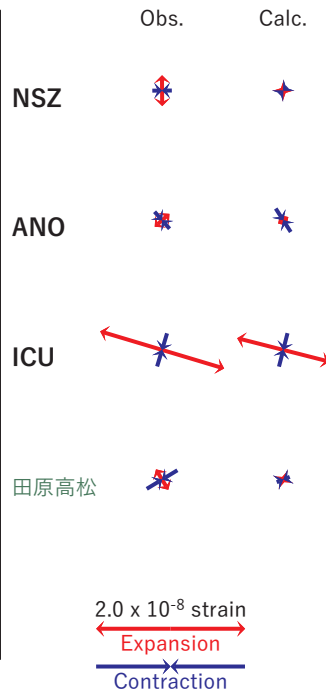
図27 2017/4/25PM-30の歪・傾斜・地下水変化（図25[B]）を説明する断層モデル。
