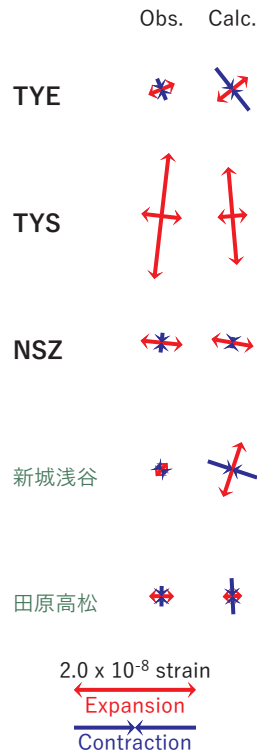
図31 2017/5/17-19の歪・傾斜変化（図30[A]）を説明する断層モデル。
