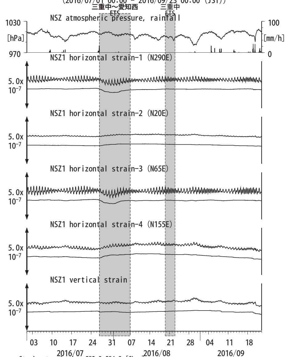
図4: Crustal strains changes at NSZ 西尾善明 (時間値) (2016/07/01 00:00 - 2016/09/23 00:00 (JST))
