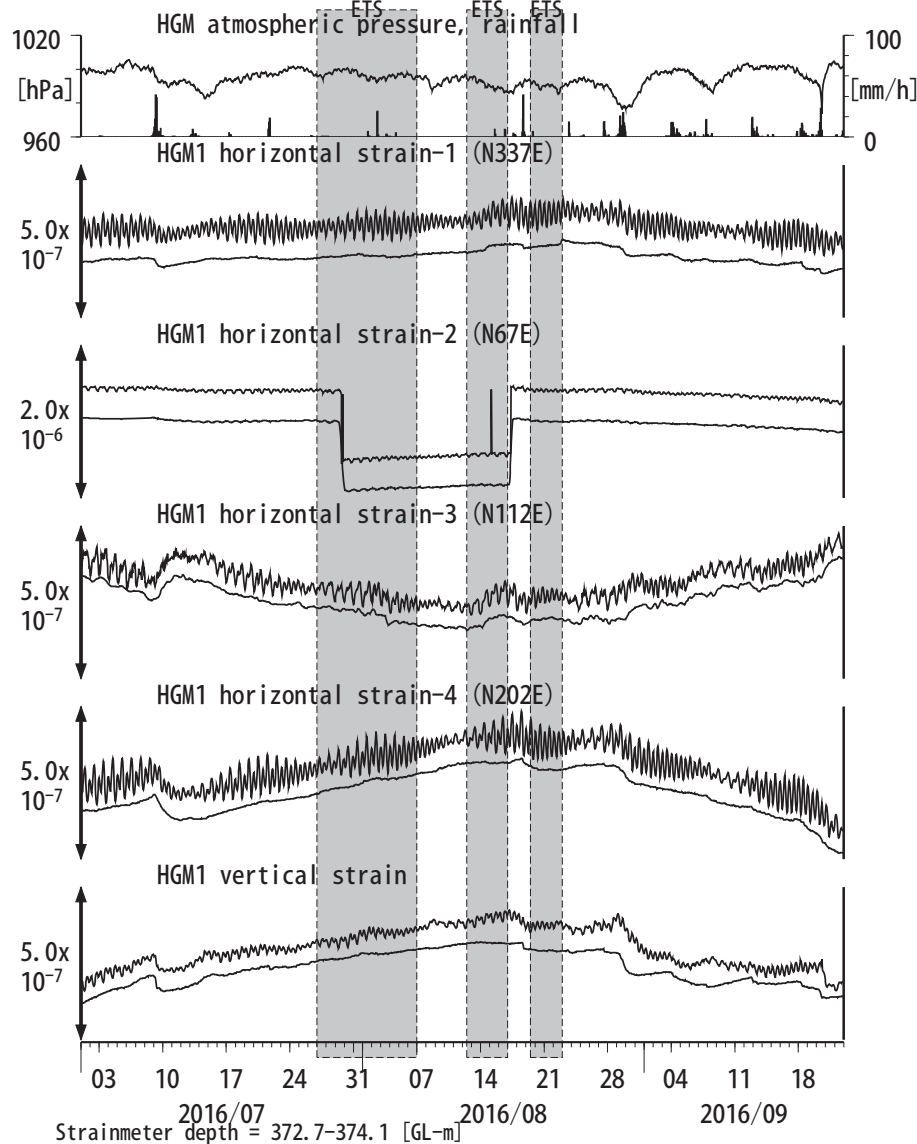
図17: Crustal strains changes at HGM 田辺本宮 (時間値) (2016/07/01 00:00 - 2016/09/23 00:00 (JST))
