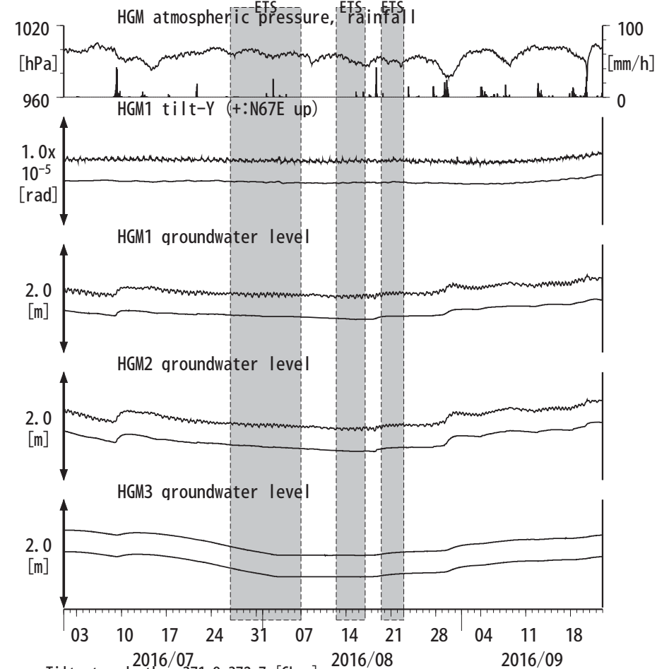
図18: Tilt and groundwater level changes at HGM 田辺本宮 (時間値) (2016/07/01 00:00 - 2016/09/23 00:00 (JST))
