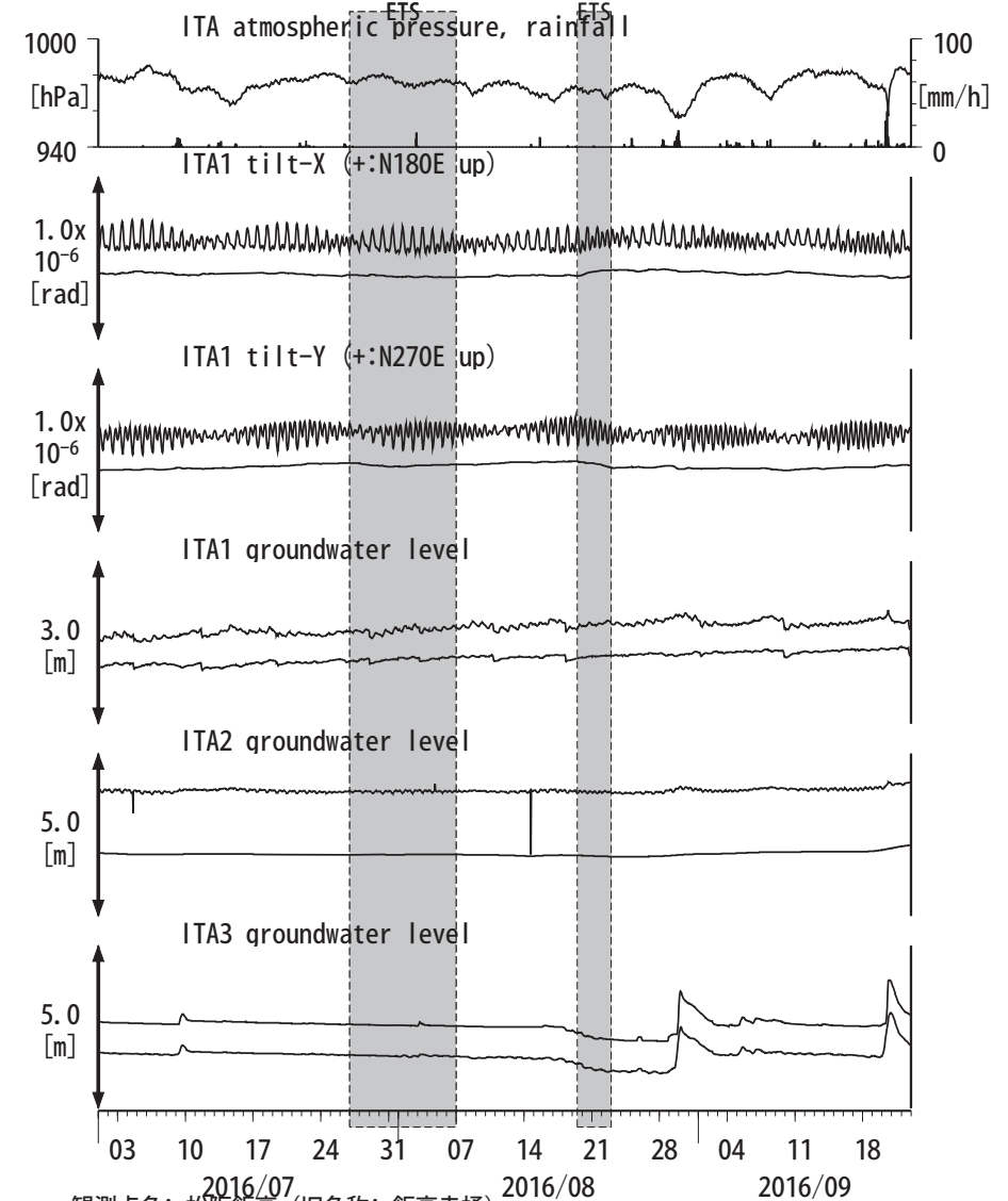
図12: Tilt and groundwater level changes at ITA 松阪飯高 (時間値) (2016/07/01 00:00 - 2016/09/23 00:00 (JST)) 三重中～愛知西 三重中
