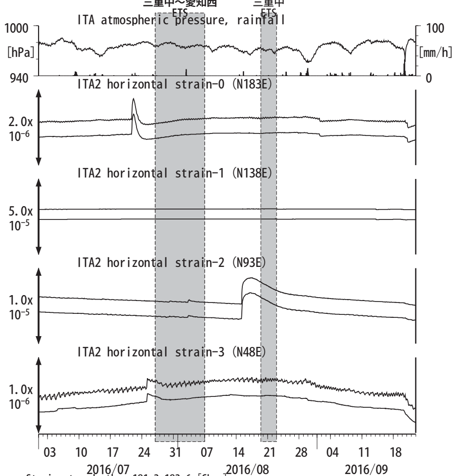
図11: Crustal strain changes at ITA 松阪飯高 (時間値) (2016/07/01 00:00 - 2016/09/23 00:00 (JST)) 三重中～愛知西 三重中
