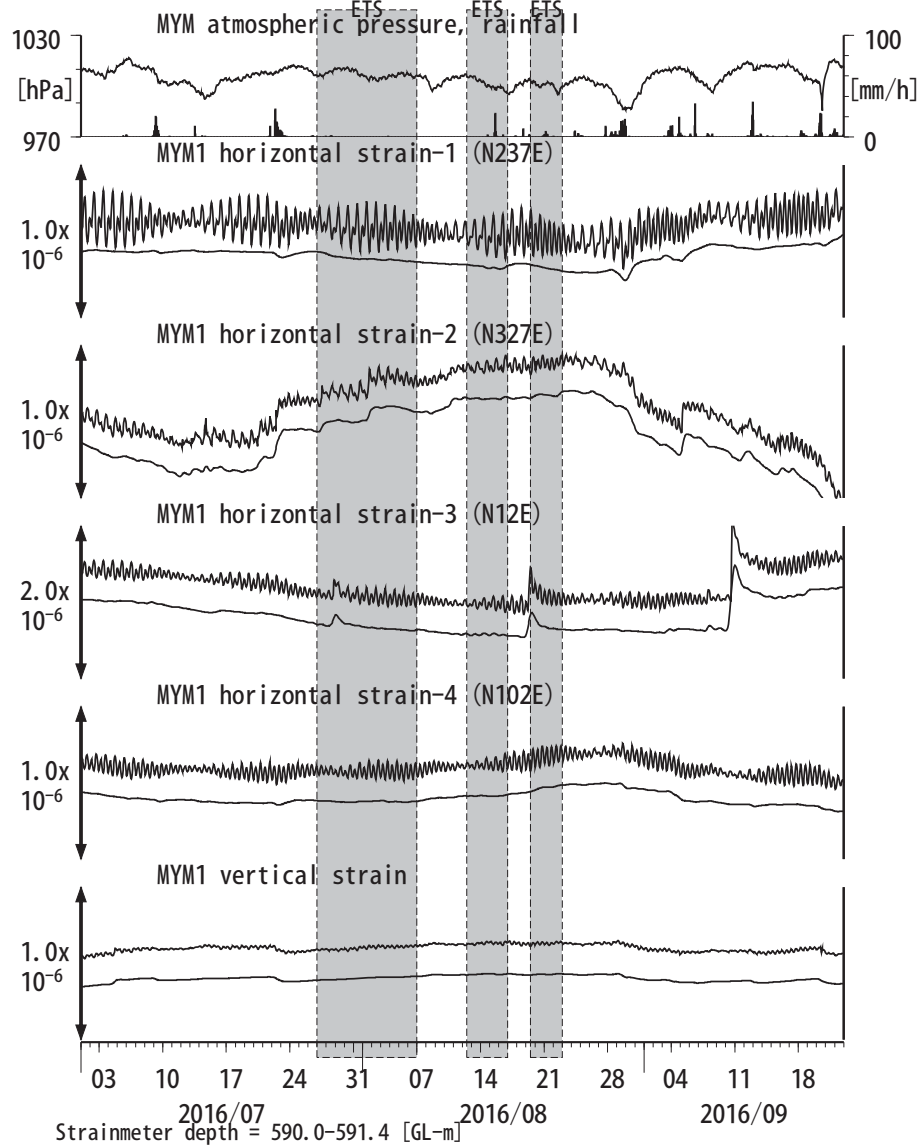
図13: Crustal strain changes at MYM 紀北海山 (時間値) (2016/07/01 00:00 - 2016/09/23 00:00 (JST))
