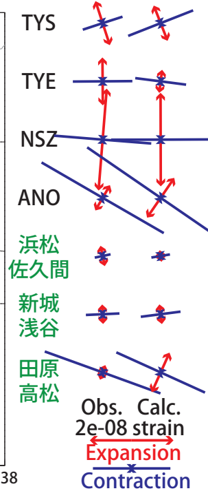
(b2) 主歪の比較
