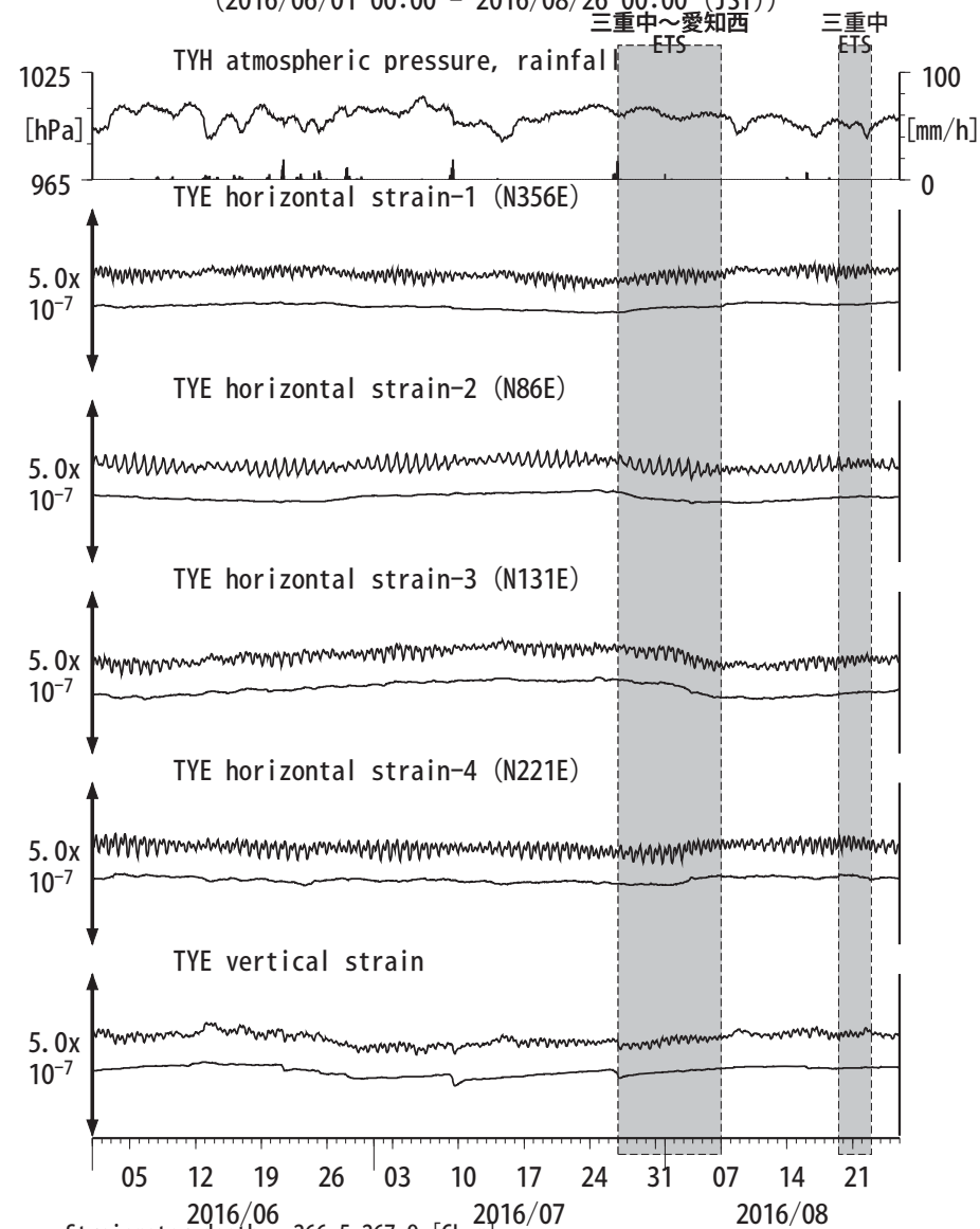
図6: Crustal strain changes at TYE 豊橋多米 (時間値) (2016/06/01 00:00 - 2016/08/26 00:00 (JST))
