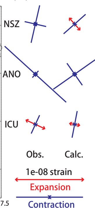
(b2) 主歪の比較
