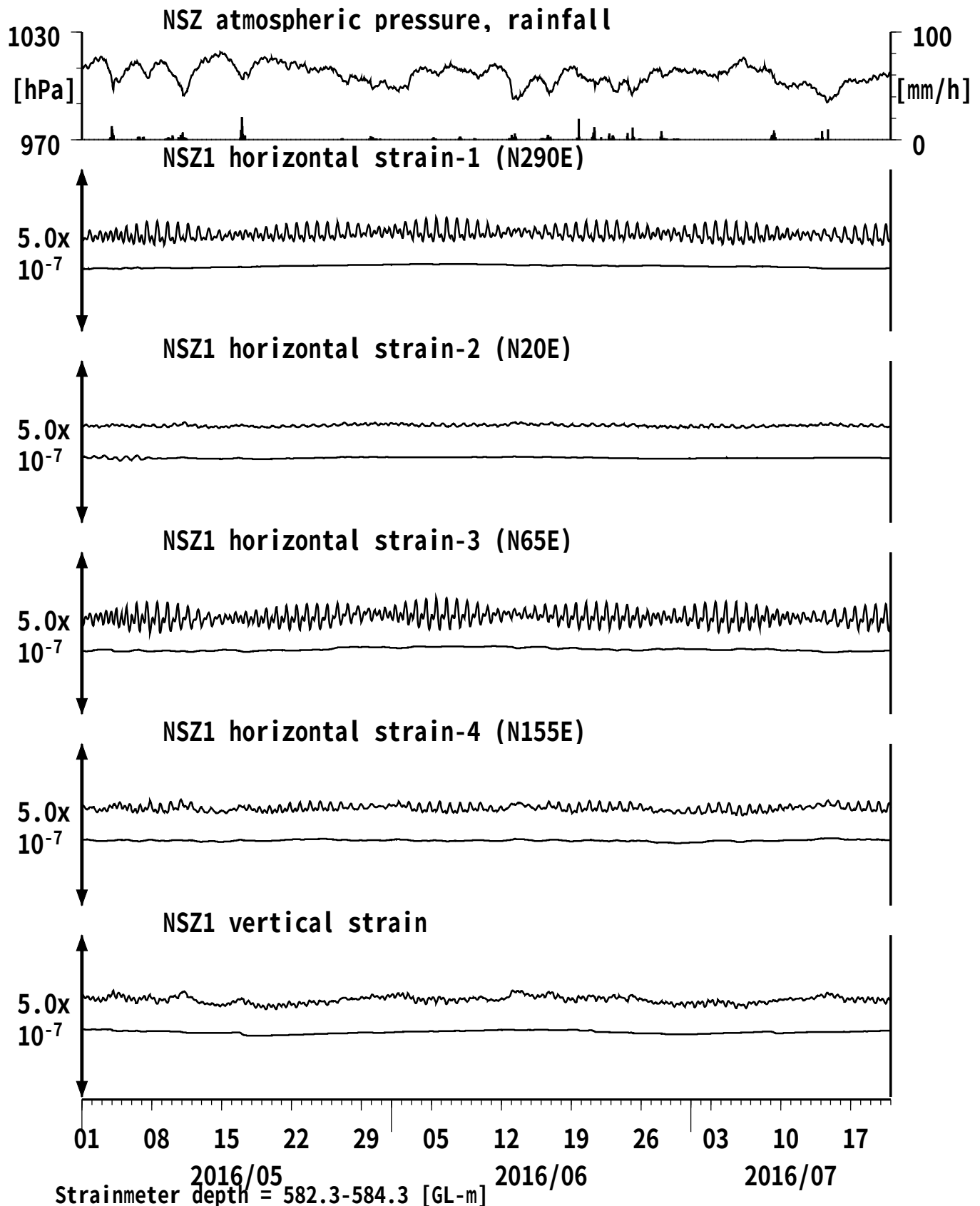
図4: Crustal strains changes at NSZ 西尾善明 (時間値) (2016/05/01 00:00 - 2016/07/21 00:00 (JST))
