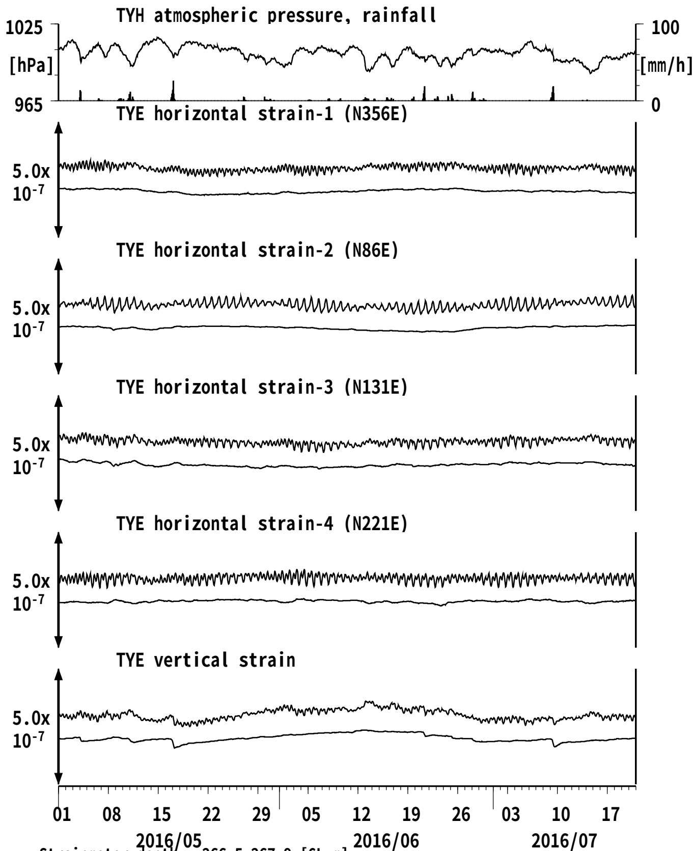
図6: Crustal strain changes at TYE 豊橋多米 (時間値) (2016/05/01 00:00 - 2016/07/21 00:00 (JST))
