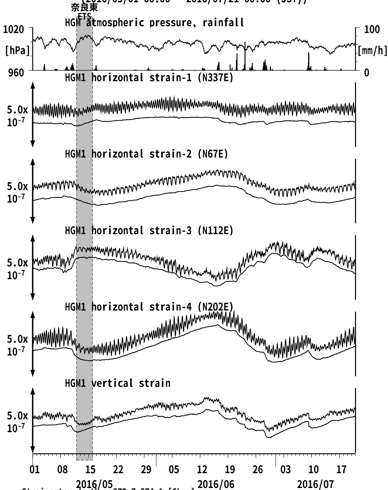
図17: Crustal strains changes at HGM 田辺本宮 (時間値) (2016/05/01 00:00 - 2016/07/21 00:00 (JST))
