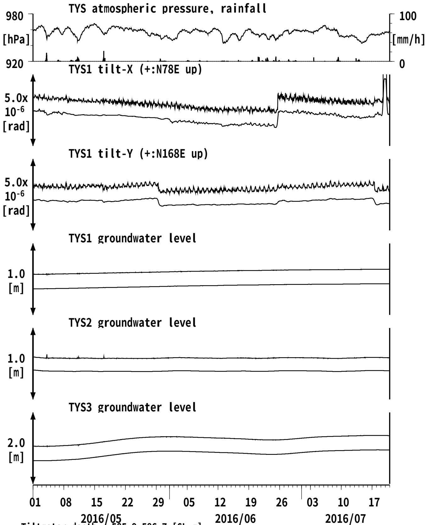
図3: Tilt and groundwater level changes at TYS 豊田神殿 (時間値) (2016/05/01 00:00 - 2016/07/21 00:00 (JST))
