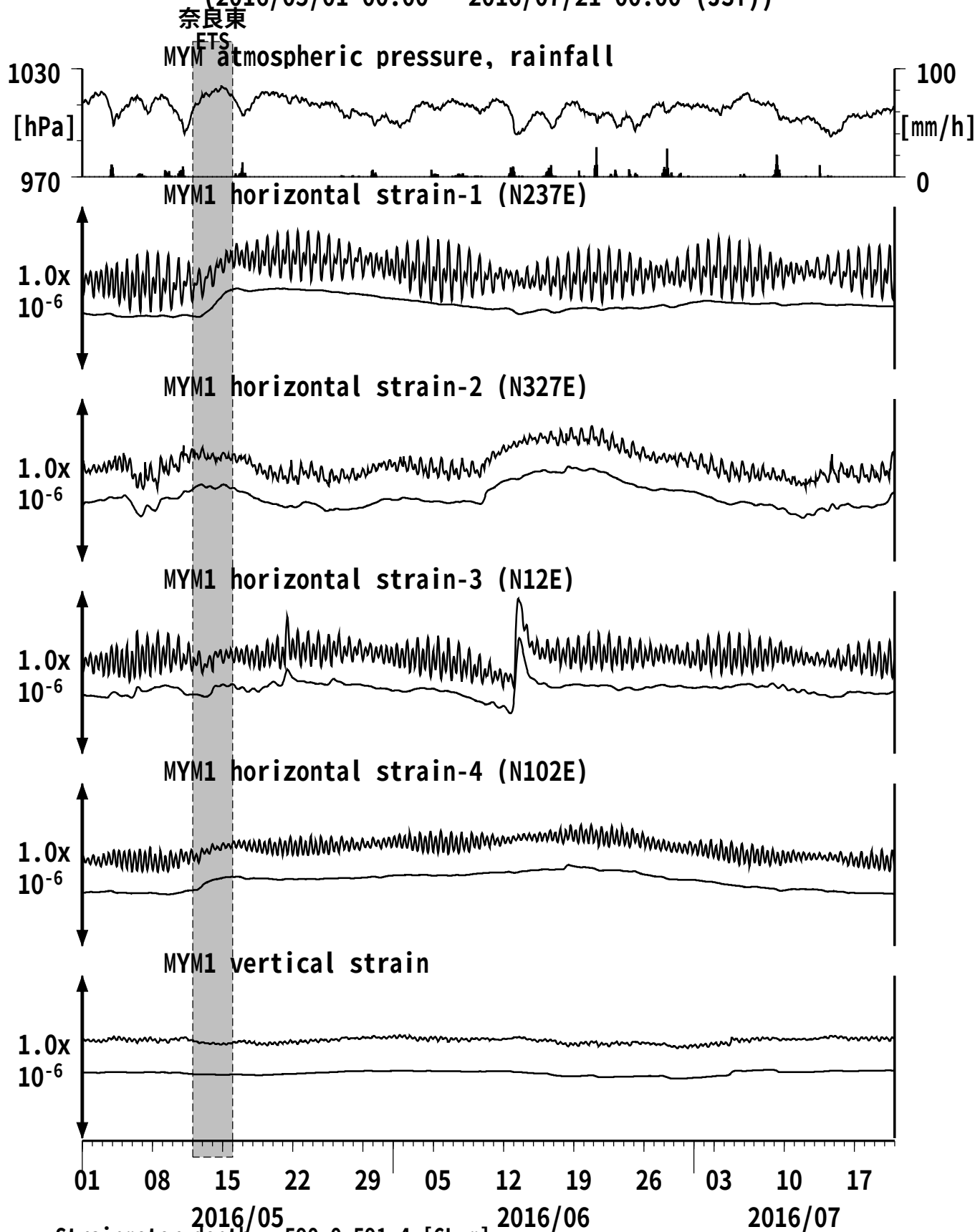
図13: Crustal strain changes at MYM 紀北海山 (時間値) (2016/05/01 00:00 - 2016/07/21 00:00 (JST))
