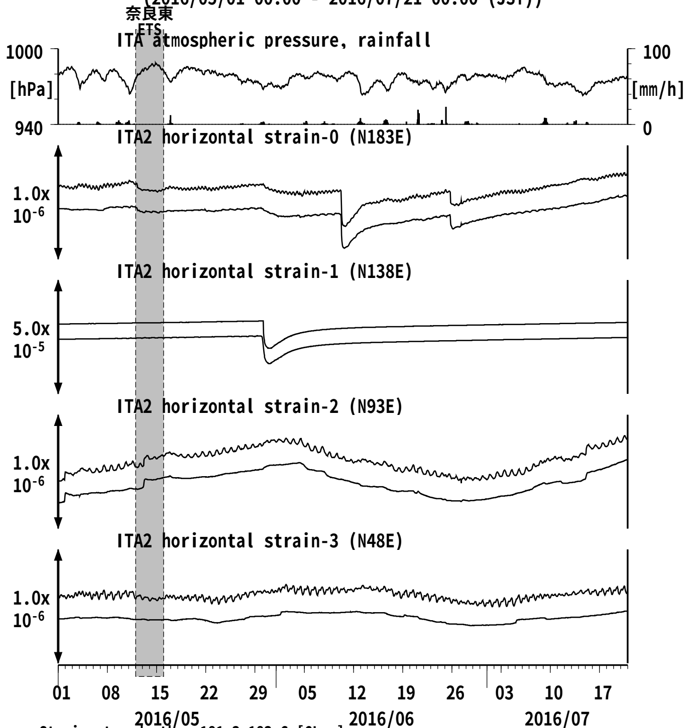
図11: Crustal strain changes at ITA 松阪飯高 (時間値) (2016/05/01 00:00 - 2016/07/21 00:00 (JST))
