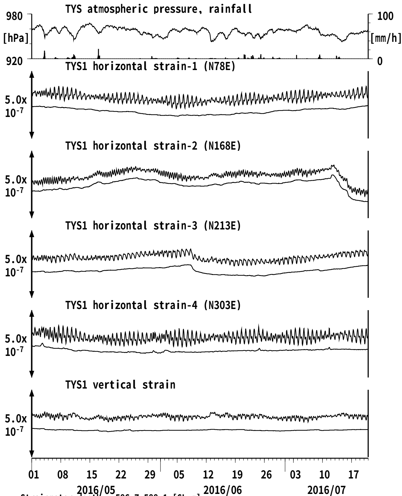
図2: Crustal strains changes at TYS 豊田神殿 (時間値) (2016/05/01 00:00 - 2016/07/21 00:00 (JST))
