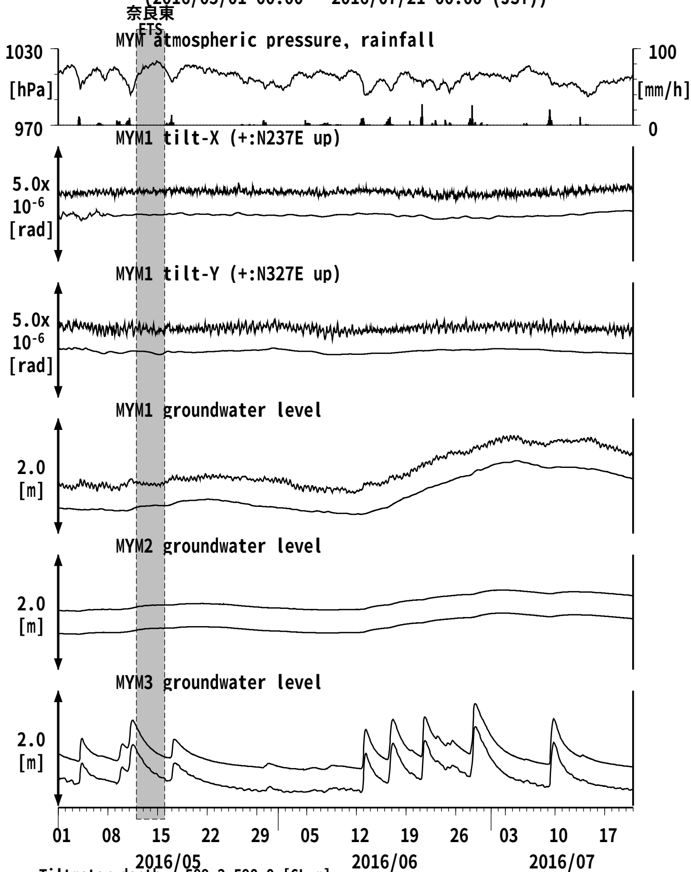
図14: Tilt and groundwater level changes at MYM 紀北海山 (時間値) (2016/05/01 00:00 - 2016/07/21 00:00 (JST))
