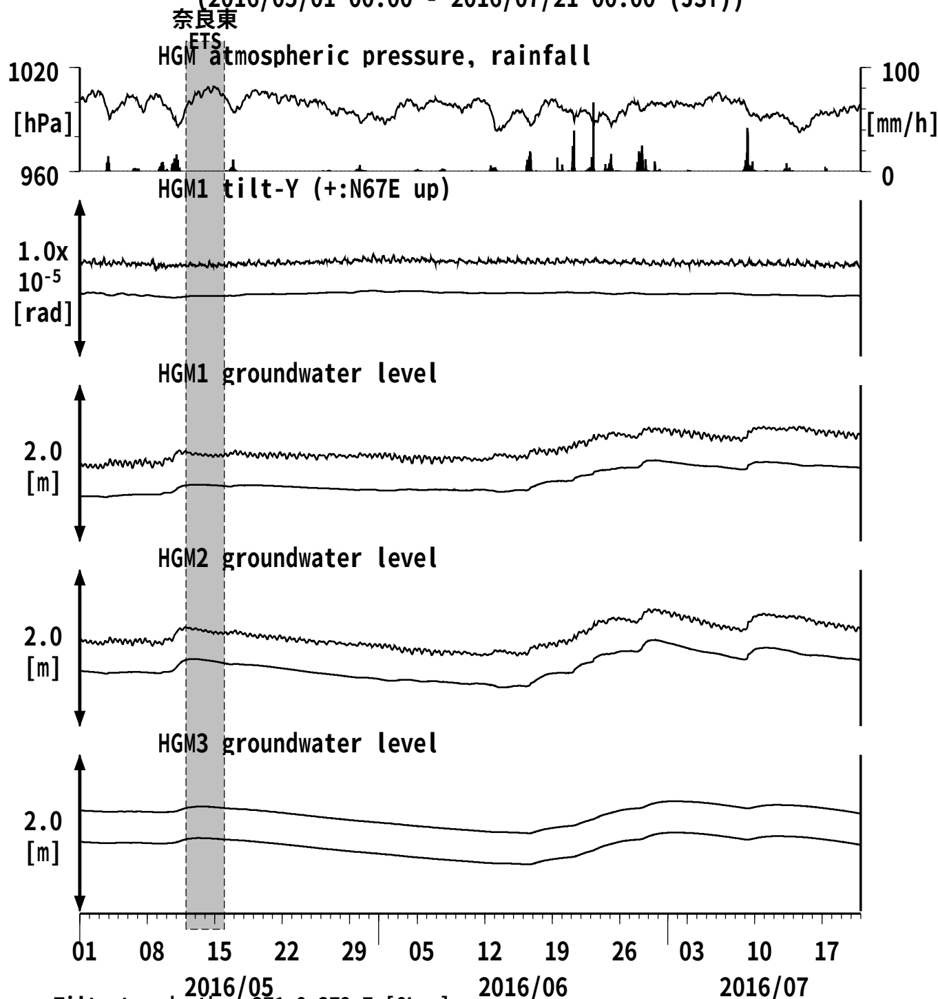
図18: Tilt and groundwater level changes at HGM 田辺本宮 (時間値) (2016/05/01 00:00 - 2016/07/21 00:00 (JST))
