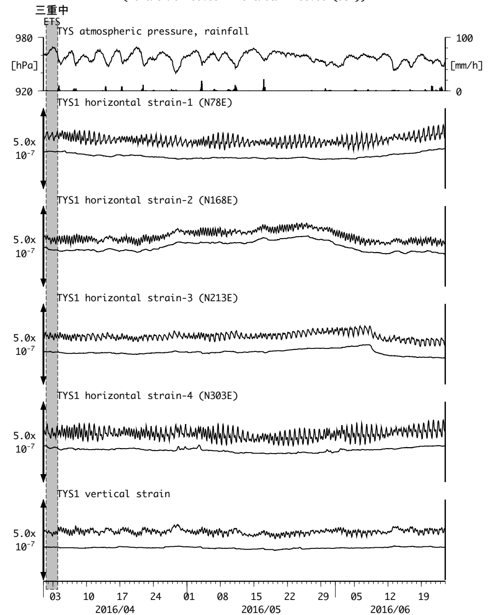
図2 : Crustal strains changes at TYS 豊田神殿 (時間値) (2016/04/01 00:00 - 2016/06/24 00:00 (JST))
