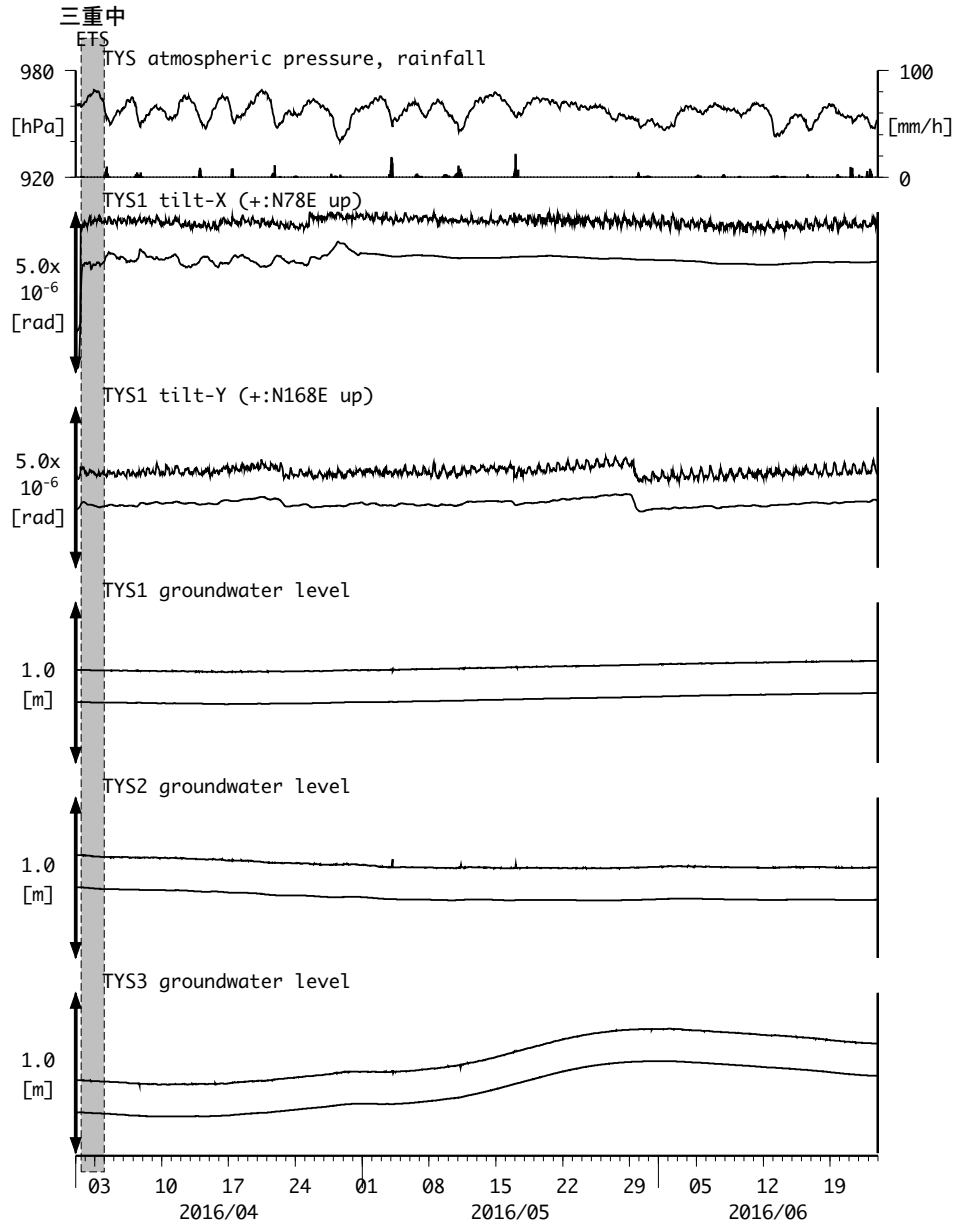
図3: Tilt and groundwater level changes at TYS 豊田神殿 (時間値) (2016/04/01 00:00 - 2016/06/24 00:00 (JST))
