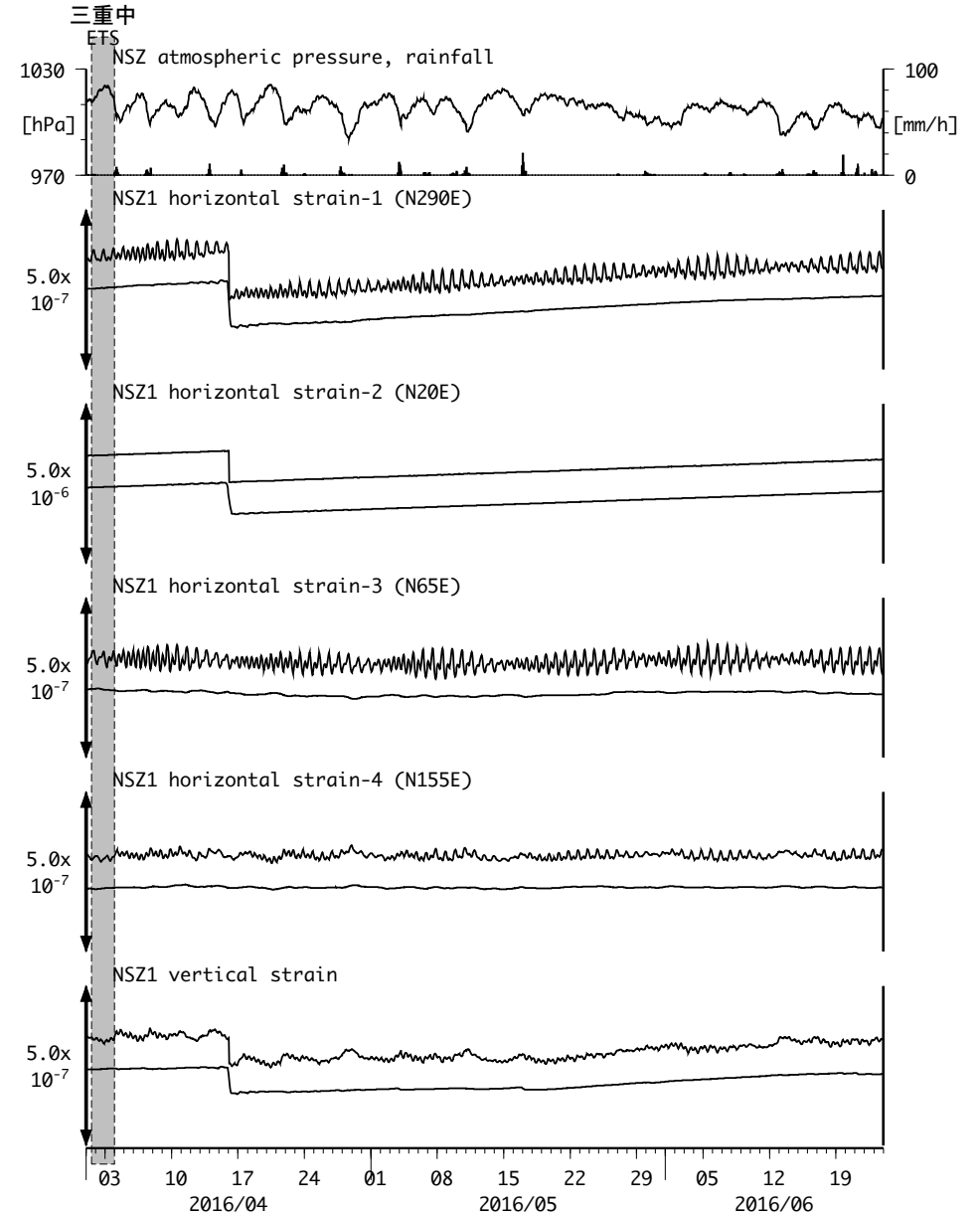
図4: Crustal strains changes at NSZ 西尾善明 (時間値) (2016/04/01 00:00 - 2016/06/24 00:00 (JST))
