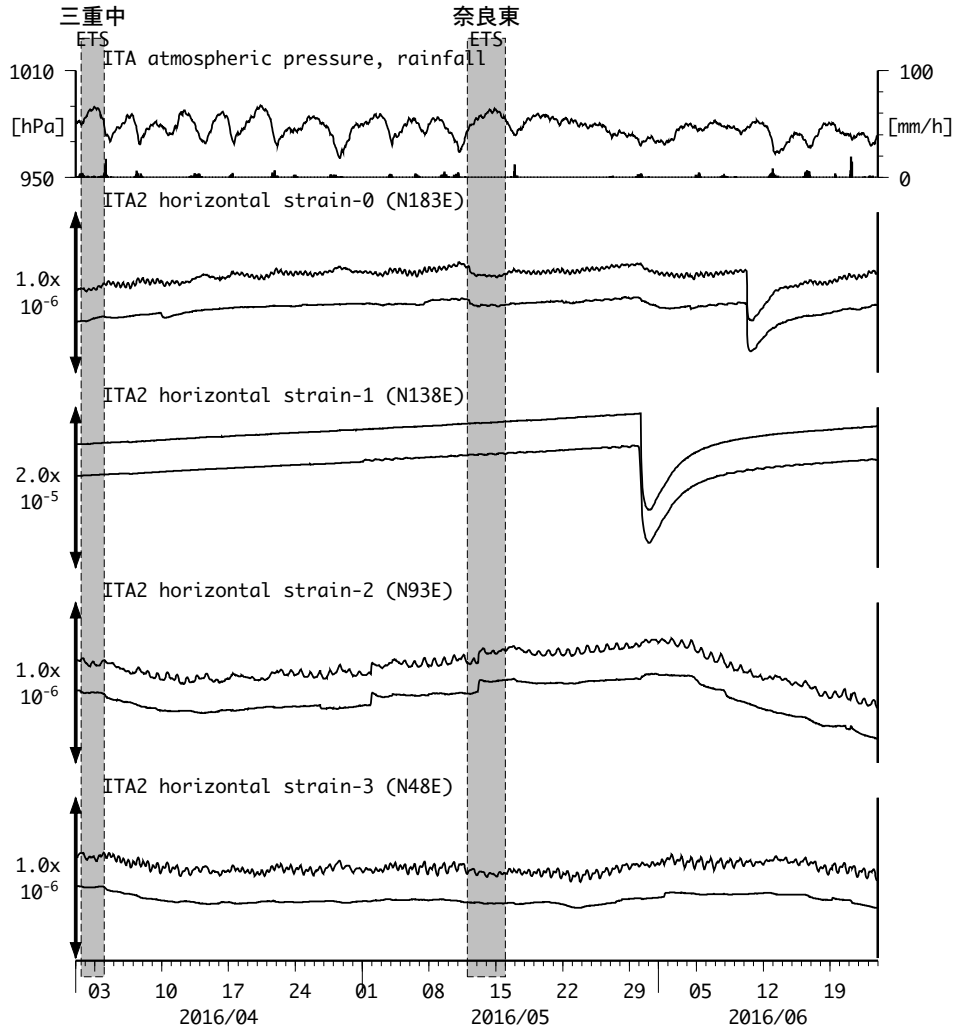
図11: Crustal strain changes at ITA 松阪飯高 (時間値) (2016/04/01 00:00 - 2016/06/24 00:00 (JST))
