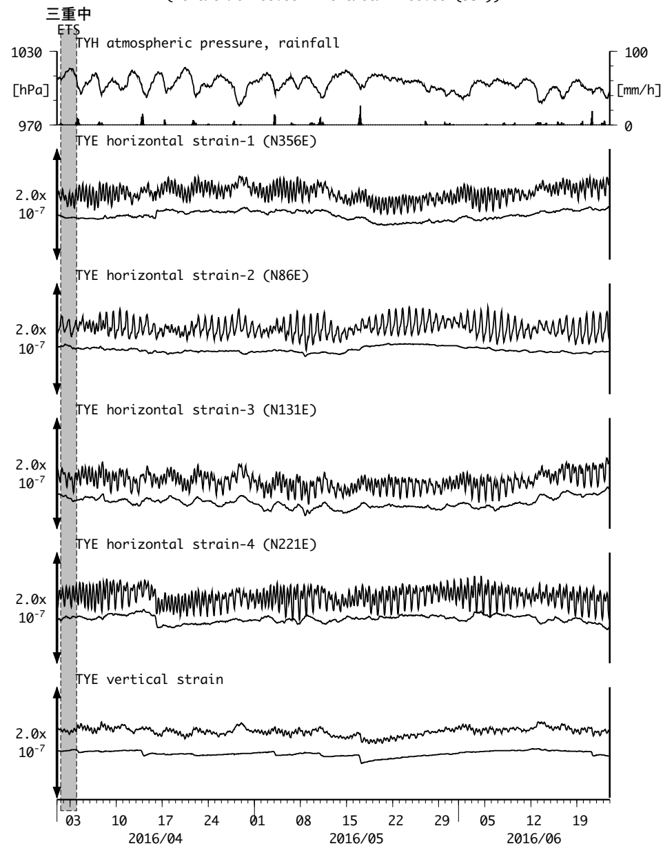
図6: Crustal strain changes at TYE 豊橋多米 (時間値) (2016/04/01 00:00 - 2016/06/24 00:00 (JST))
