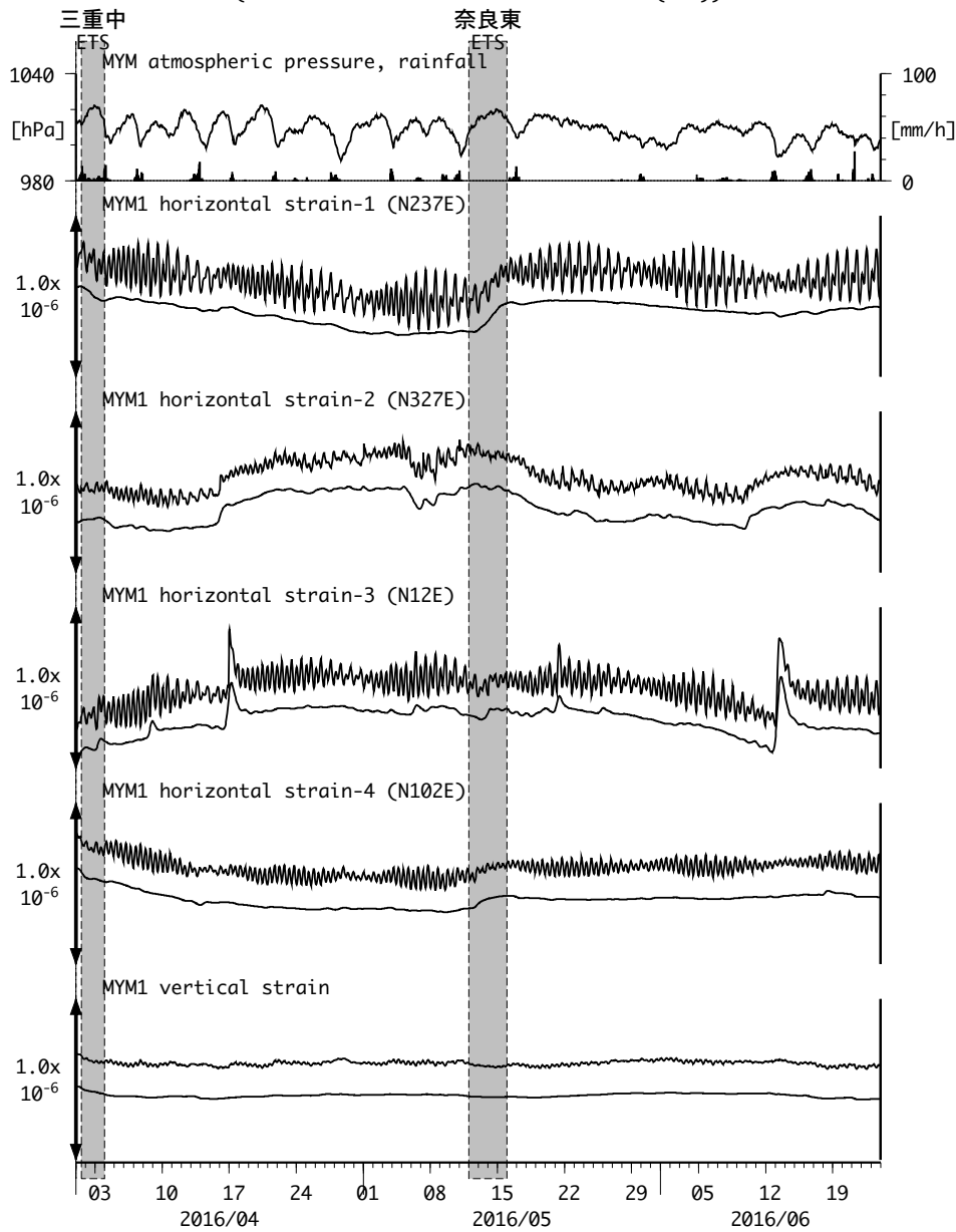
図13 : Crustal strain changes at MYM 紀北海山 (時間値) (2016/04/01 00:00 - 2016/06/24 00:00 (JST))
