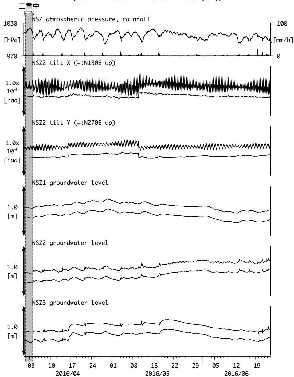
図5: Tilt and groundwater level changes at NSZ 西尾善明 (時間値) (2016/04/01 00:00 - 2016/06/24 00:00 (JST))
