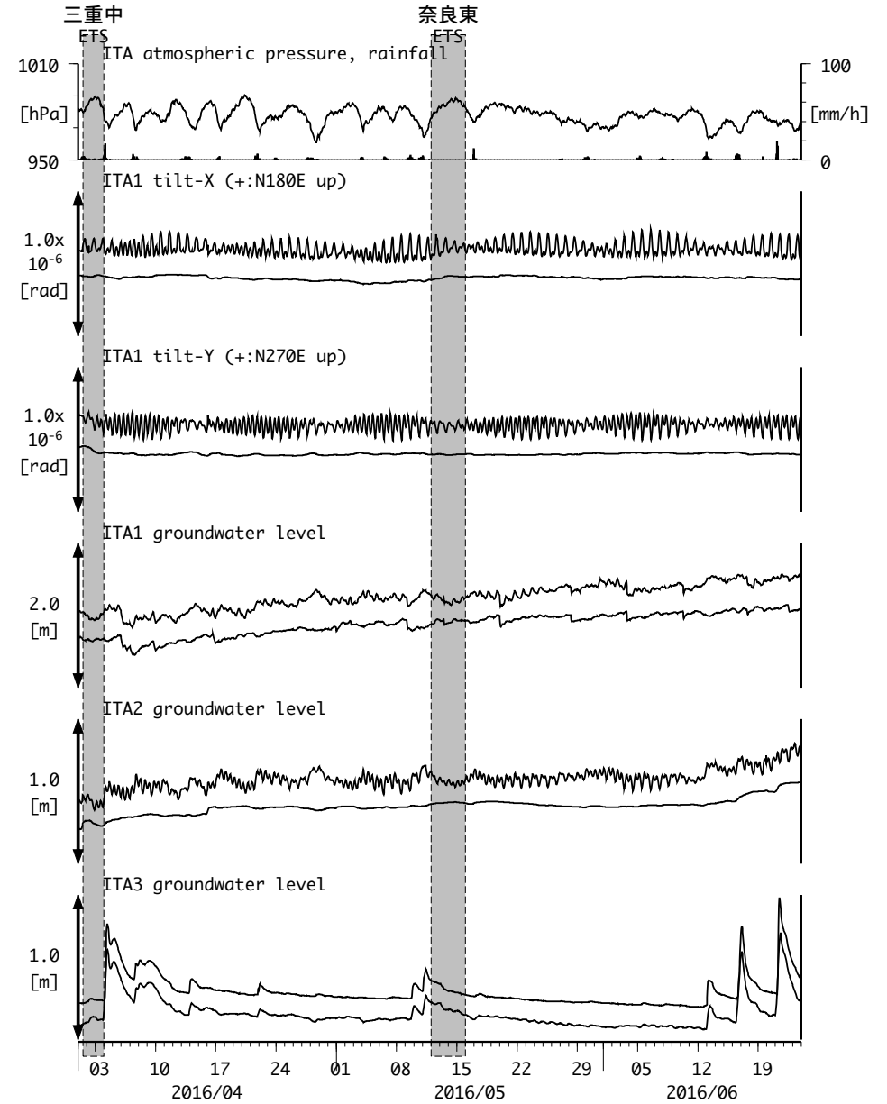
図12: Tilt and groundwater level changes at ITA 松阪飯高 (時間値) (2016/04/01 00:00 - 2016/06/24 00:00 (JST))
