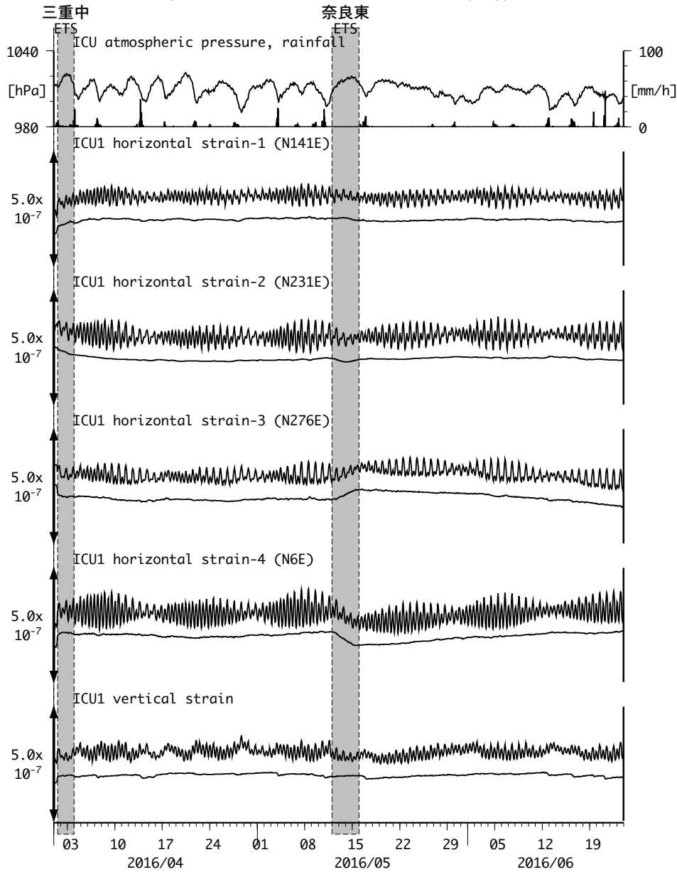
図15 : Crustal strain changes at ICU 熊野磯崎 (時間値) (2016/04/01 00:00 - 2016/06/24 00:00 (JST))
