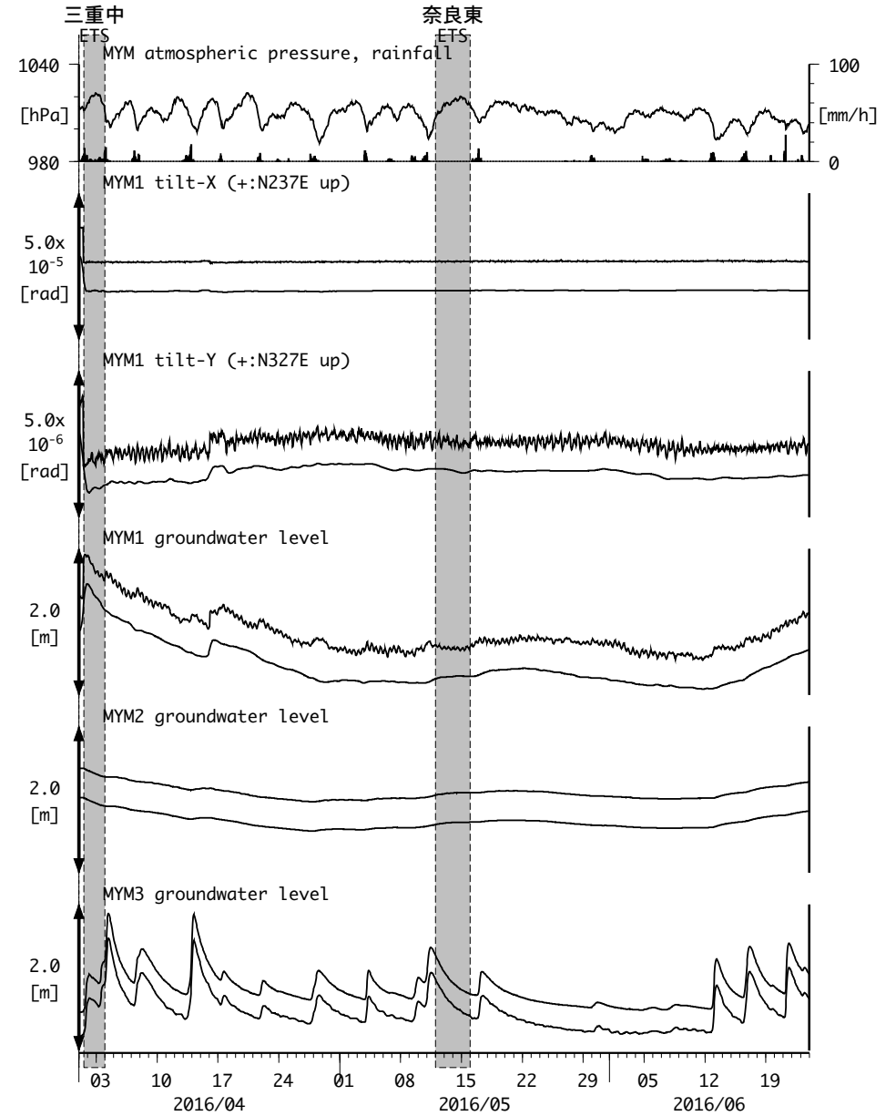
図14 : Tilt and groundwater level changes at MYM 紀北海山 (時間値) (2016/04/01 00:00 - 2016/06/24 00:00 (JST))
