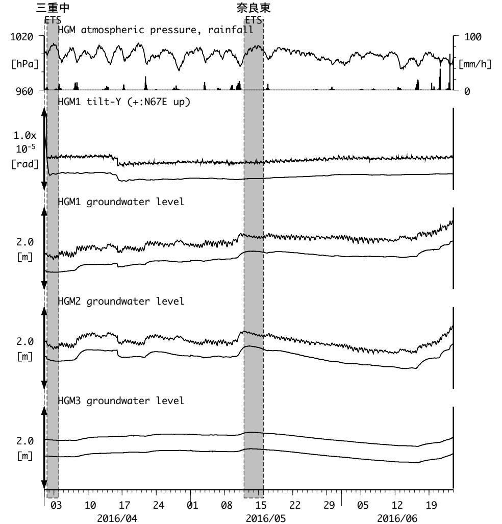
図18 : Tilt and groundwater level changes at HGM 田辺本宮 (時間値) (2016/04/01 00:00 - 2016/06/24 00:00 (JST))
