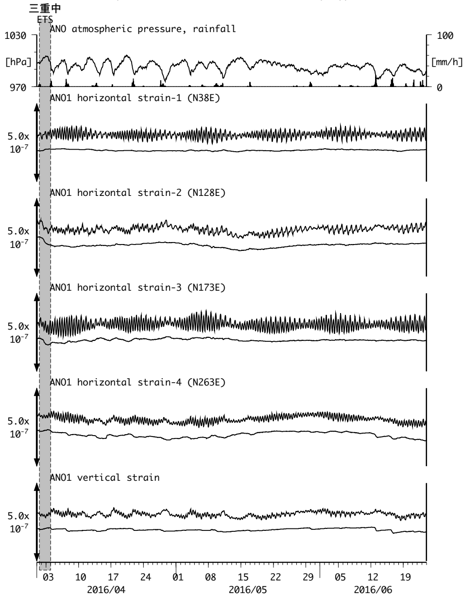
図9 : Crustal strains changes at ANO 津安濃 (時間値) (2016/04/01 00:00 - 2016/06/24 00:00 (JST))
