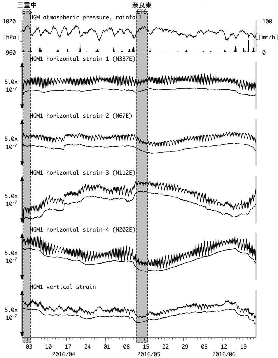
図17 : Crustal strains changes at HGM 田辺本宮 (時間値) (2016/04/01 00:00 - 2016/06/24 00:00 (JST))
