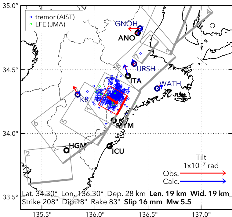
図26 2016/5/12-13の歪・傾斜変化 (図25[A]) を説明する断層モデル。
