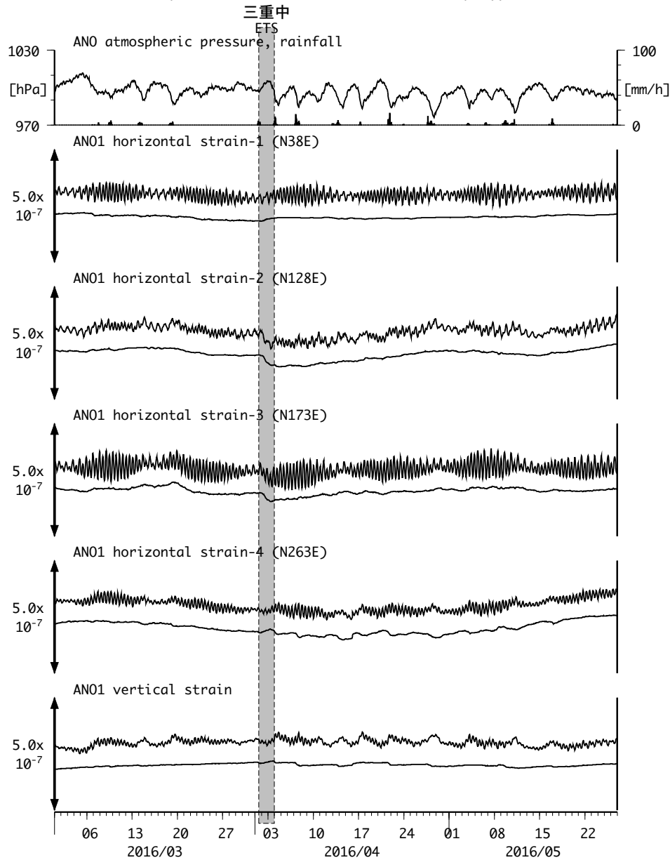
図9 : Crustal strains changes at ANO 津安濃 (時間値) (2016/03/01 00:00 - 2016/05/27 00:00 (JST))
