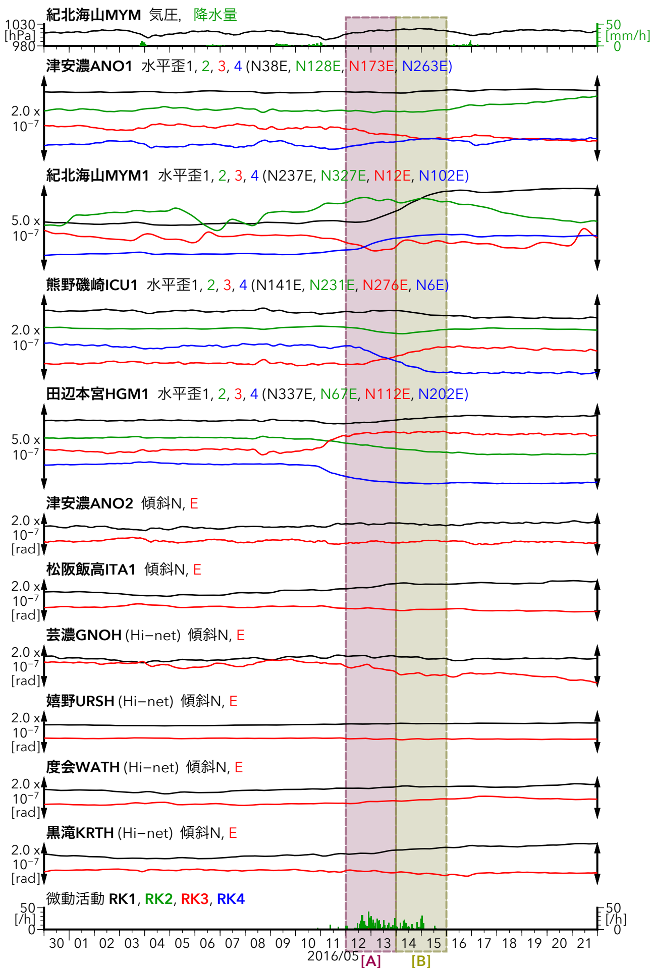
図25 紀伊半島における歪・傾斜観測結果 (2016/4/30 0:00 - 2016/5/22 0:00 (JST))
