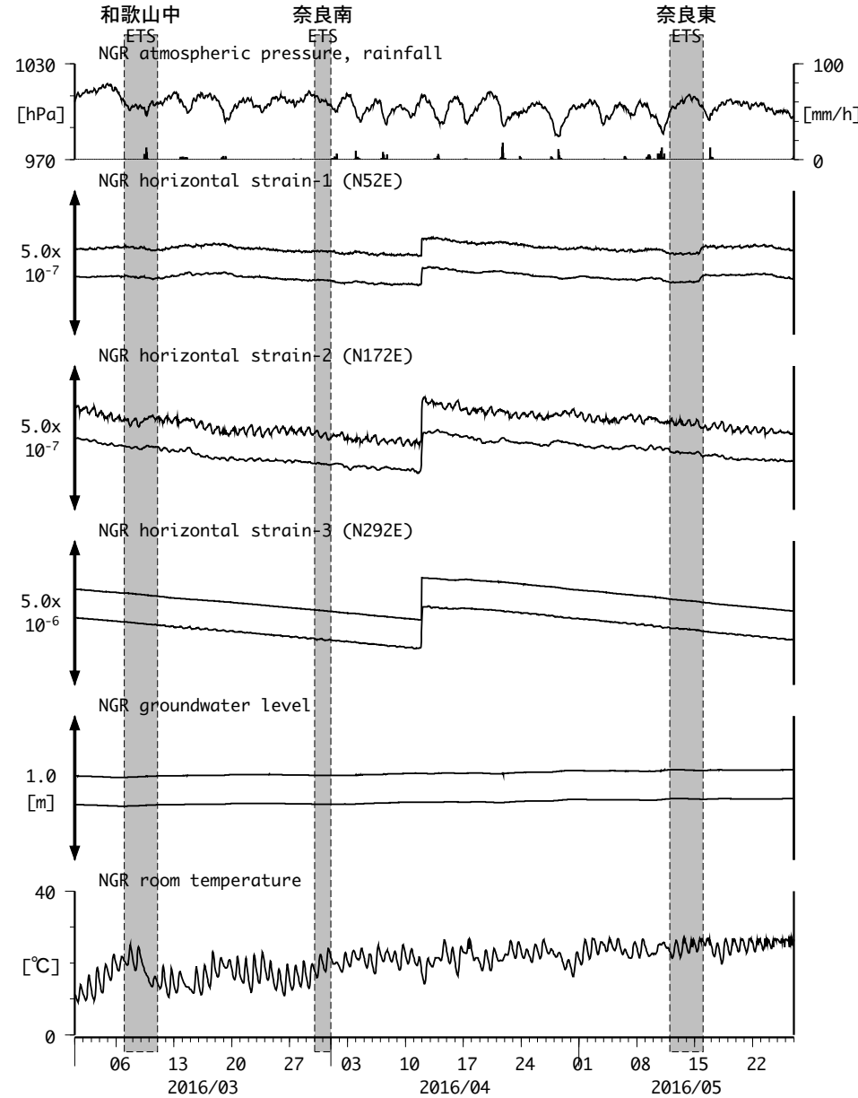
図21: Crustal strain and groundwater level changes at 岩出東坂本（時間値） (2016/03/01 00:00 - 2016/05/27 00:00 (JST))
