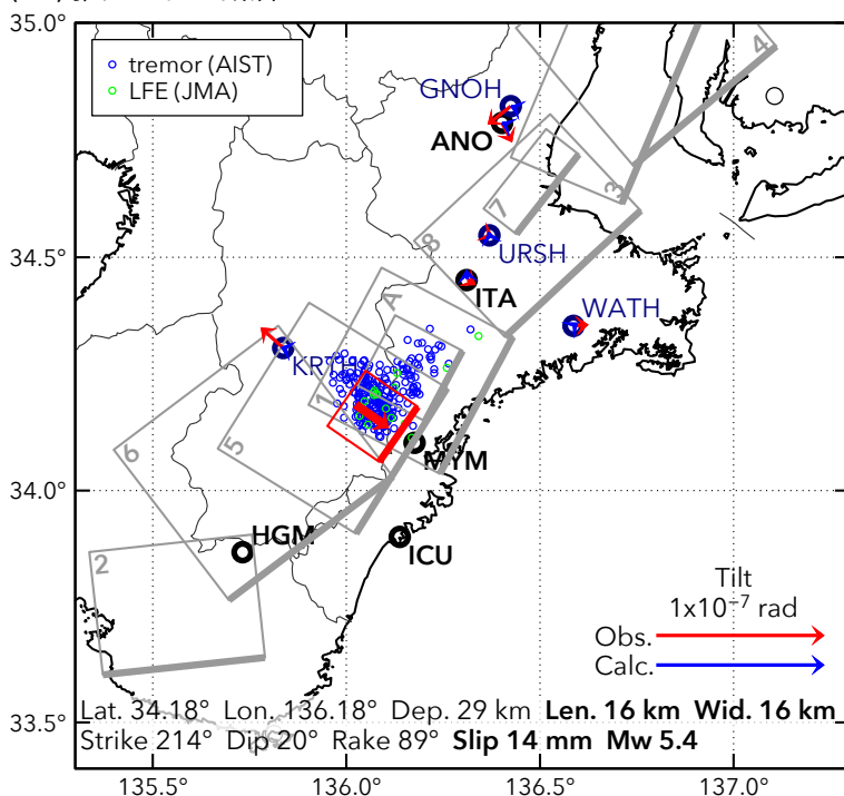
図27 2016/5/13-14の歪・傾斜変化（図25[B]）を説明する断層モデル。
