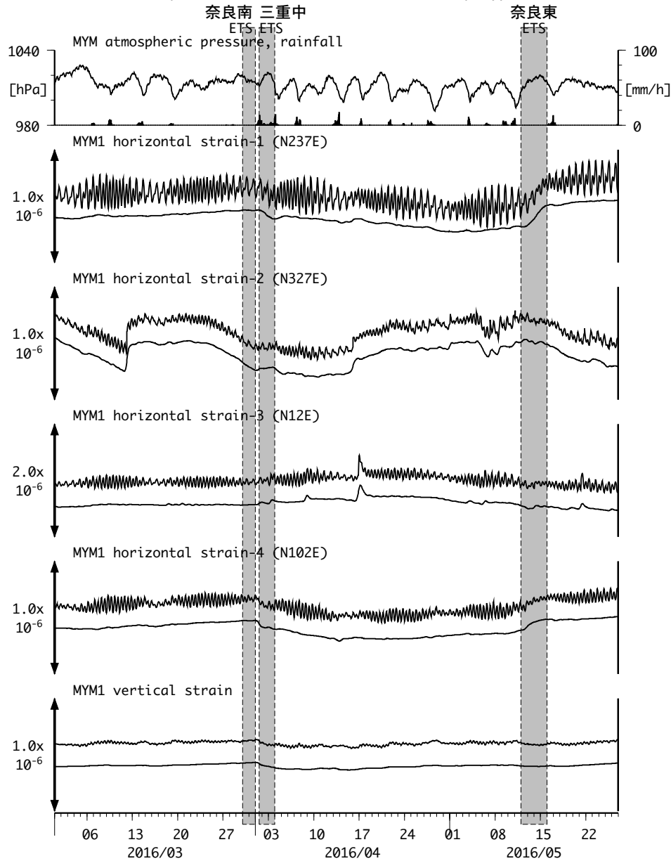
図13 : Crustal strain changes at MYM 紀北海山 (時間値) (2016/03/01 00:00 - 2016/05/27 00:00 (JST))
