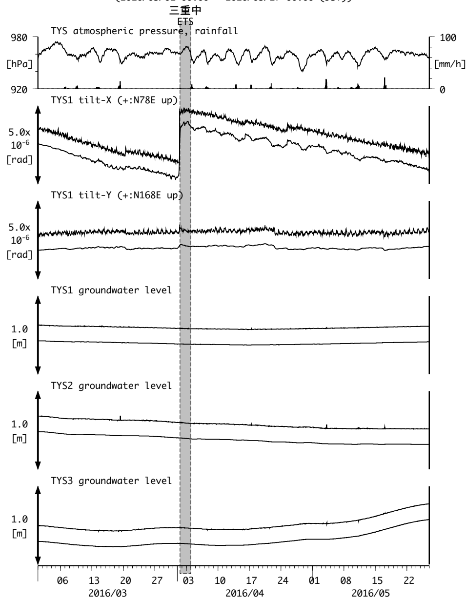
図3: Tilt and groundwater level changes at TYS 豊田神殿 (時間値) (2016/03/01 00:00 - 2016/05/27 00:00 (JST))
