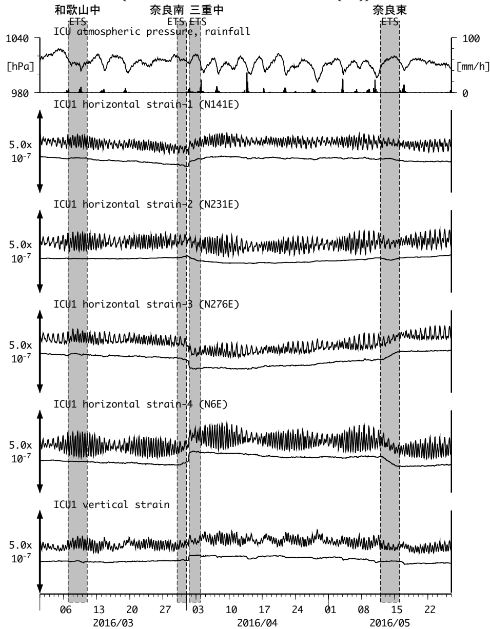
図15 : Crustal strain changes at ICU 熊野磯崎 (時間値) (2016/03/01 00:00 - 2016/05/27 00:00 (JST))
