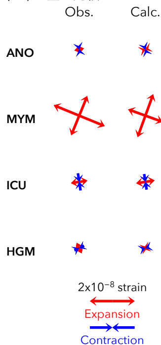
図27 2016/5/13-14の歪・傾斜変化（図25[B]）を説明する断層モデル。
