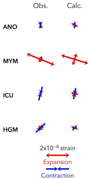
図26 2016/5/12-13の歪・傾斜変化 (図25[A]) を説明する断層モデル。
