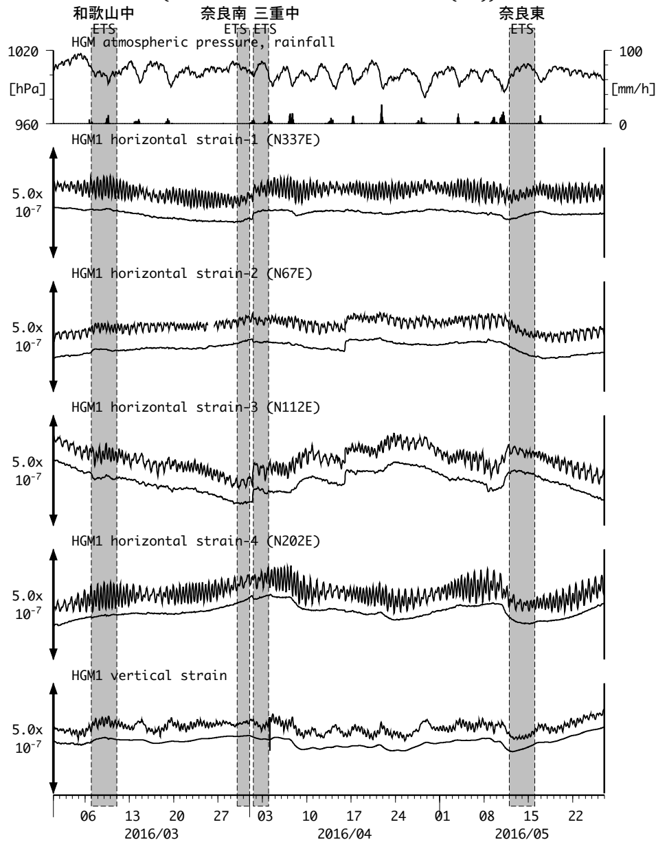
図17: Crustal strains changes at HGM 田辺本宮 (時間値) (2016/03/01 00:00 - 2016/05/27 00:00 (JST))
