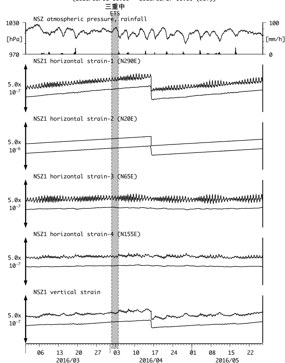
図4: Crustal strains changes at NSZ 西尾善明 (時間値) (2016/03/01 00:00 - 2016/05/27 00:00 (JST))
