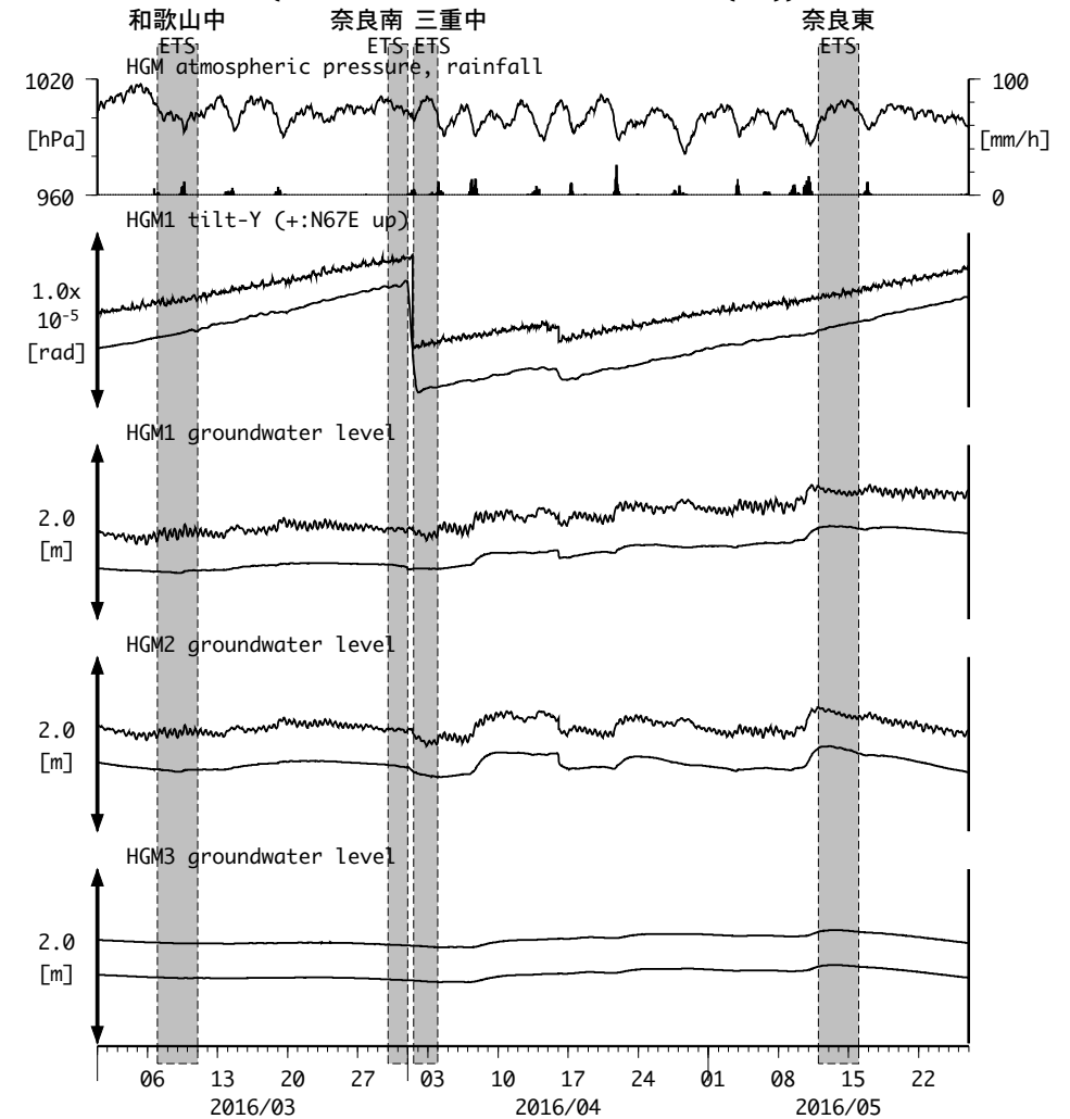
図18: Tilt and groundwater level changes at HGM 田辺本宮 (時間値) (2016/03/01 00:00 - 2016/05/27 00:00 (JST))
