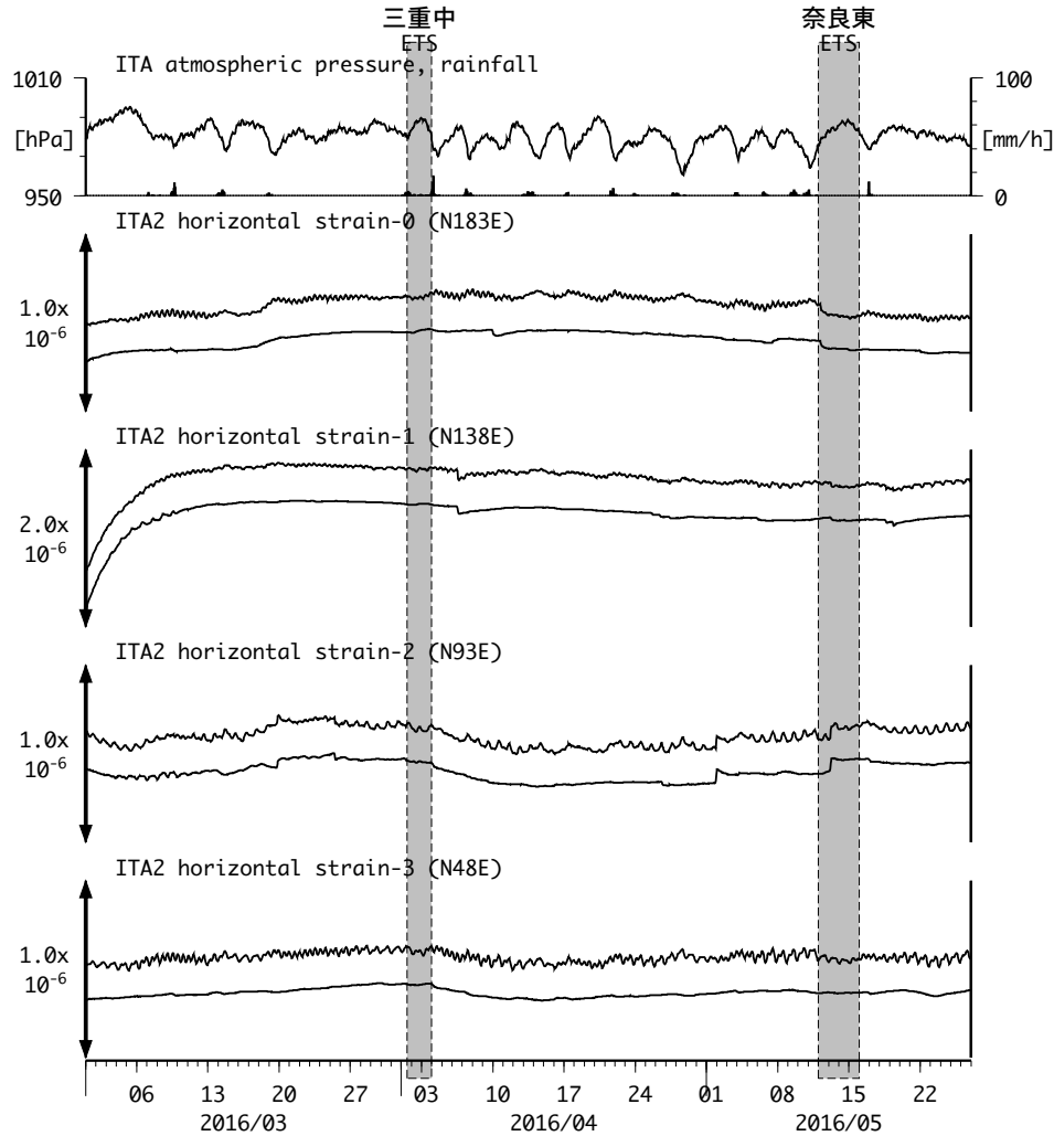
図11: Crustal strain changes at ITA 松阪飯高 (時間値) (2016/03/01 00:00 - 2016/05/27 00:00 (JST))
