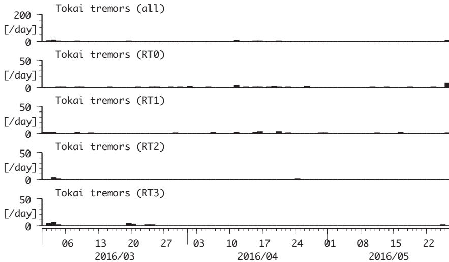
図22 (上段) 愛知県およびその周辺における深部低周波微動の時空間分布, (下段) 各領域における発生頻度 (日値)。
