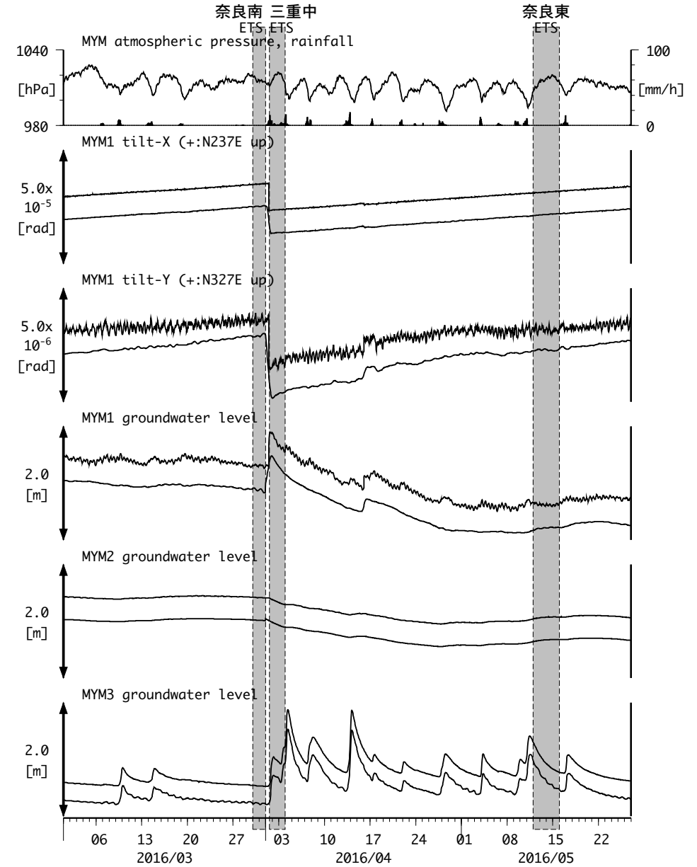
図14 : Tilt and groundwater level changes at MYM 紀北海山 (時間値) (2016/03/01 00:00 - 2016/05/27 00:00 (JST))
