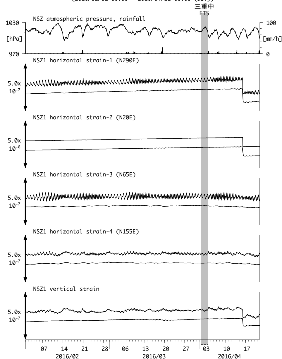
図4: Crustal strains changes at NSZ 西尾善明 (時間値)
