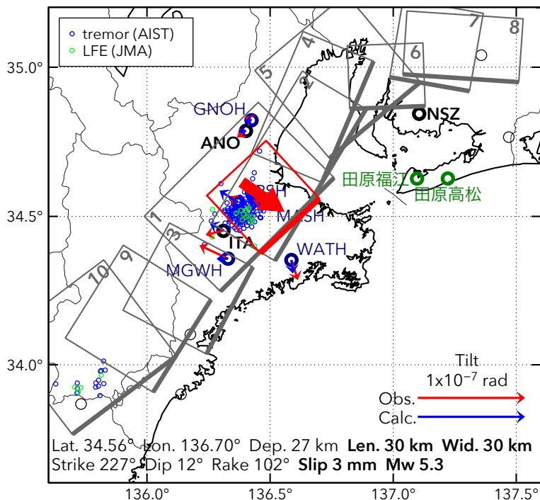
図29 2016/4/1PM-2AMの歪・傾斜変化 (図28[A]) を説明する断層モデル。
