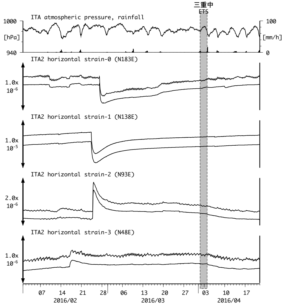
図11 : Crustal strain changes at ITA 松阪飯高 (時間値) (2016/02/01 00:00 - 2016/04/22 00:00 (JST))
