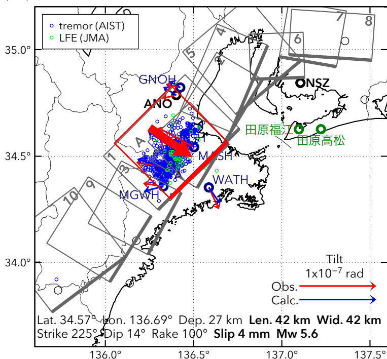
図30 2016/4/2PM-3の歪・傾斜変化(図28[B])を説明する断層モデル。
