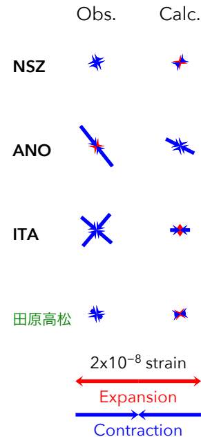
図29 2016/4/1PM-2AMの歪・傾斜変化 (図28[A]) を説明する断層モデル。
