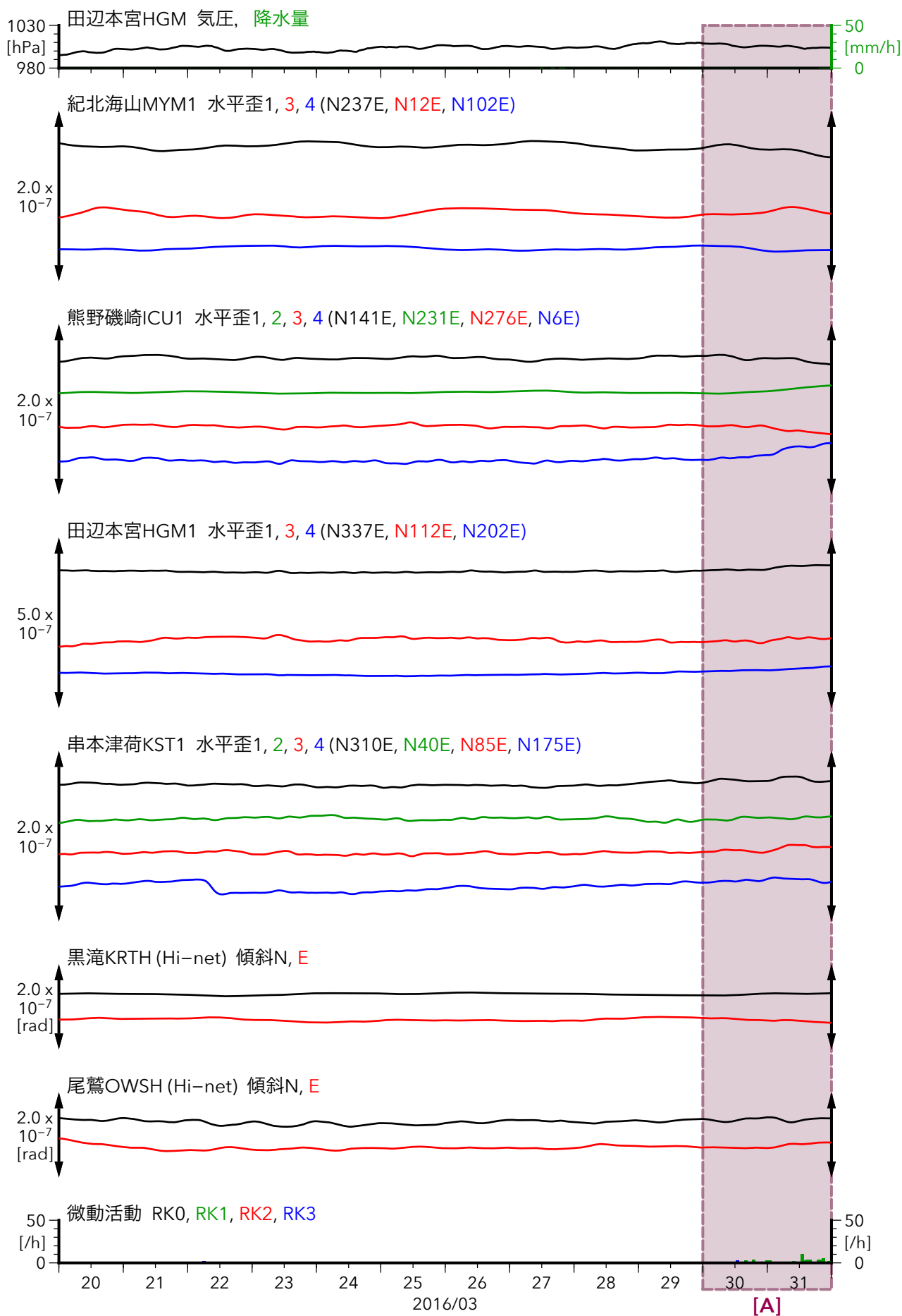
図25 紀伊半島における歪・傾斜観測結果 (2016/3/20 0:00 - 2016/4/1 0:00 (JST))
