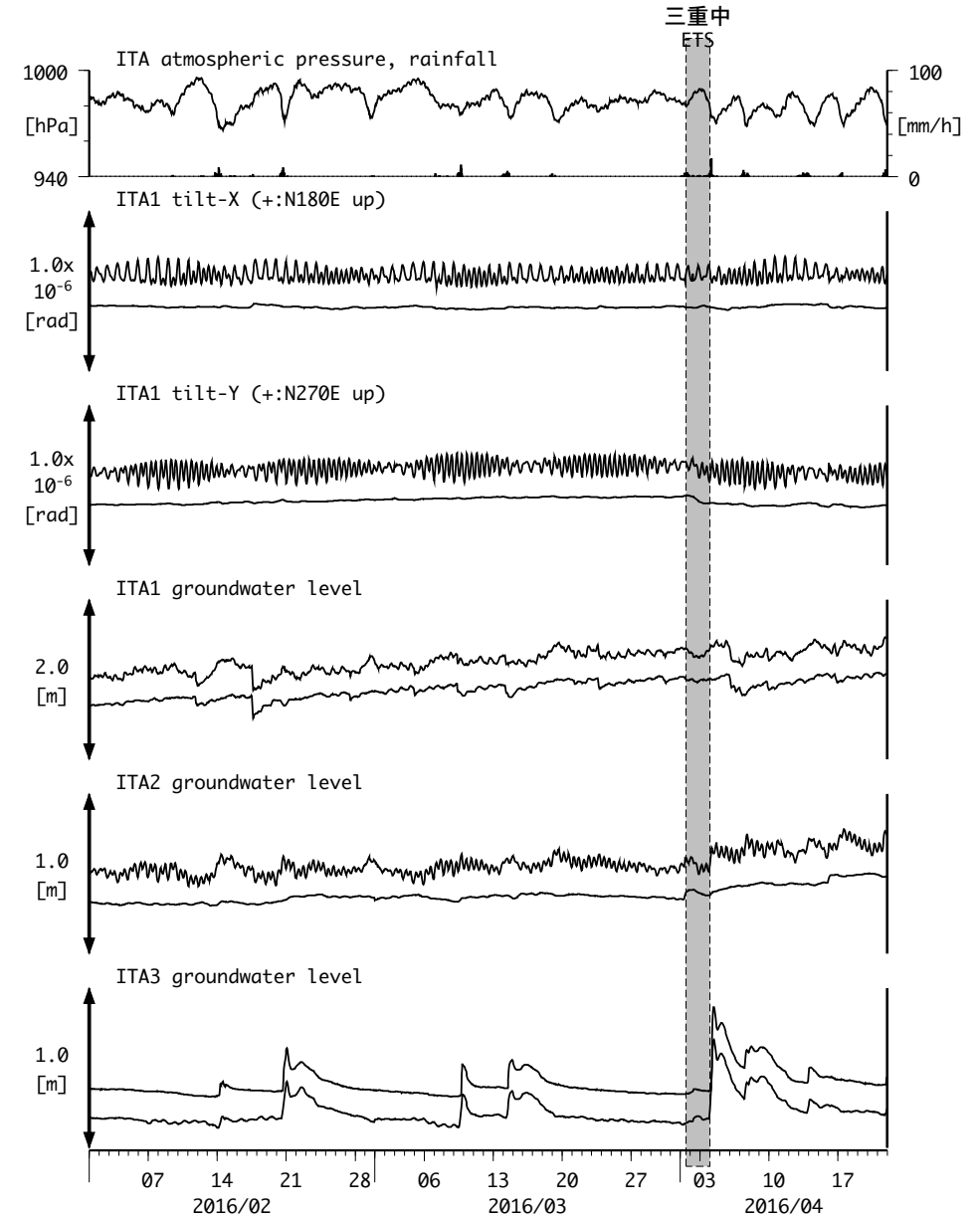
図12 : Tilt and groundwater level changes at ITA 松阪飯高 (時間値) (2016/02/01 00:00 - 2016/04/22 00:00 (JST))
