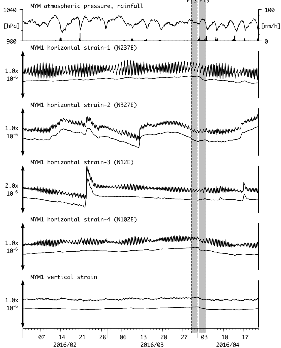
図13 : Crustal strain changes at MYM 紀北海山 (時間値)
