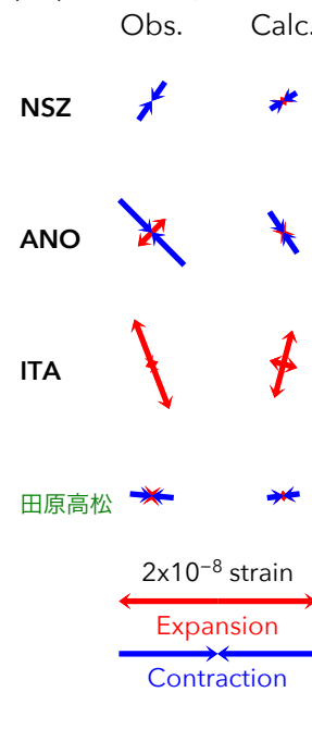
図30 2016/4/2PM-3の歪・傾斜変化(図28[B])を説明する断層モデル。
