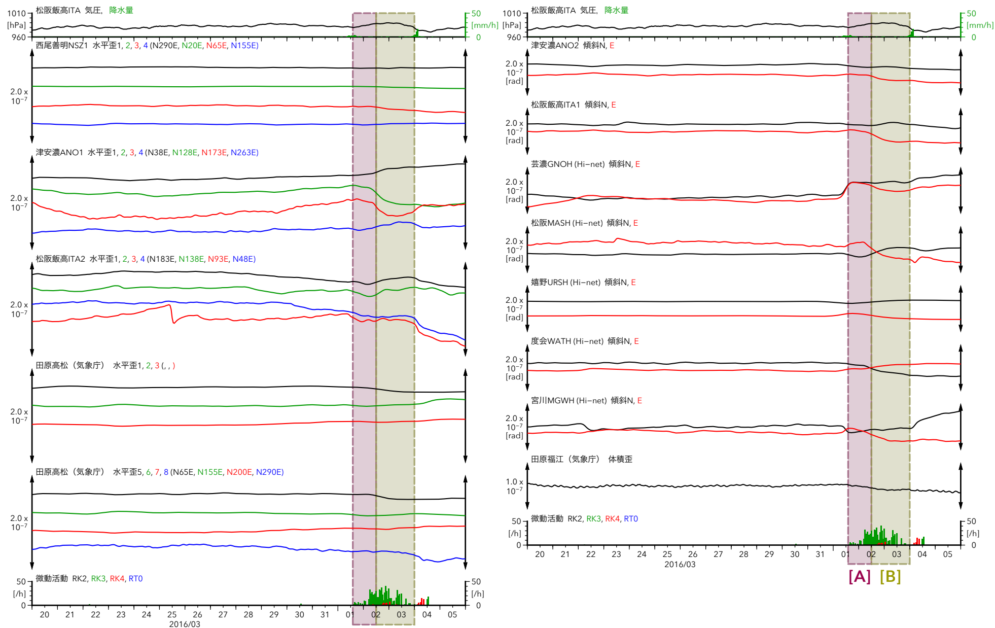
図28 東海地方・紀伊半島における歪・傾斜観測結果 (2016/3/20 0:00 - 4/6 0:00 (JST))
