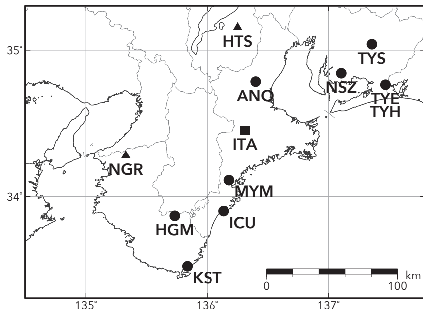
図1 紀伊半島～愛知県における地下水等総合観測施設の分布図（●・■・▲）。●はデジタル方式の石井式歪計・傾斜計を併設している観測点，■はGladwin式歪計・ミツトヨ式傾斜計を併設している観測点，▲はアナログ方式の石井式歪計を併設している観測点を示す。
