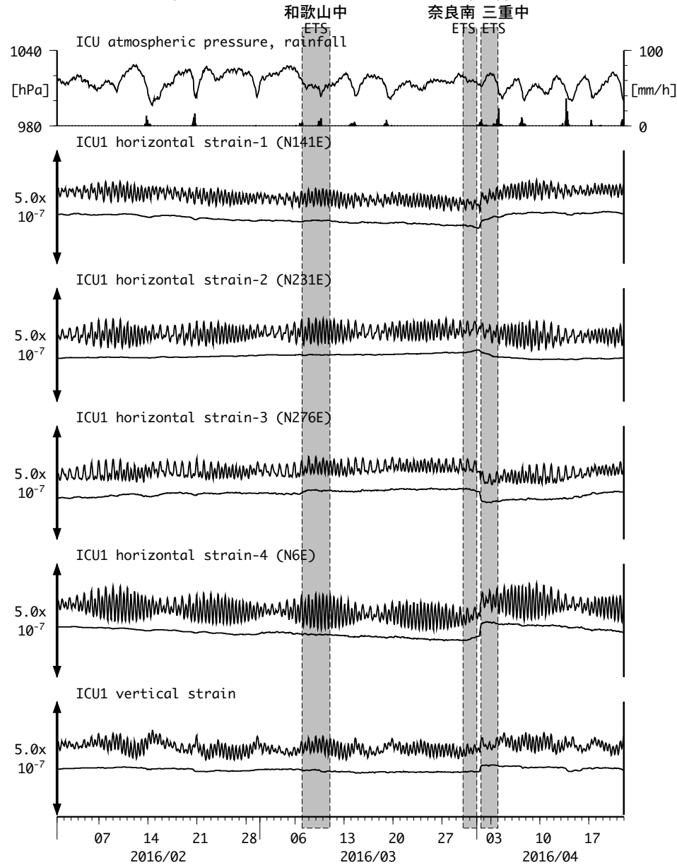
図15 : Crustal strain changes at ICU 熊野磯崎 (時間値) (2016/02/01 00:00 - 2016/04/22 00:00 (JST))
