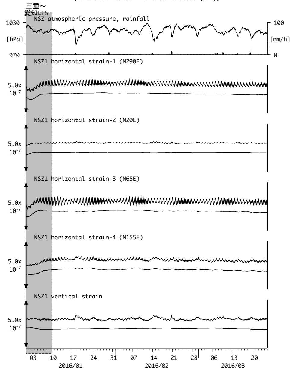
図4: Crustal strains changes at NSZ 西尾善明 (時間値) (2016/01/01 00:00 - 2016/03/25 00:00 (JST))
