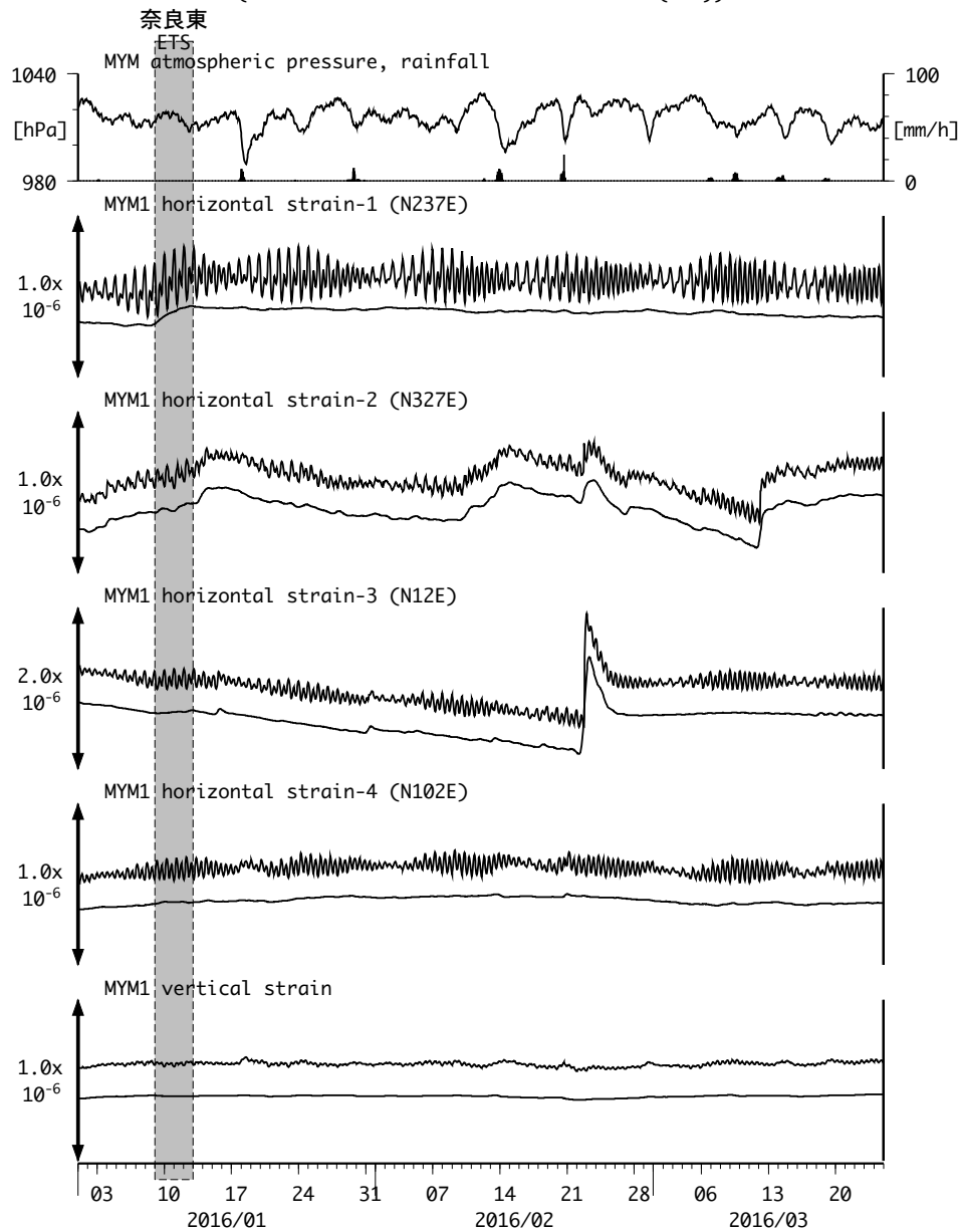
図13 : Crustal strain changes at MYM 紀北海山 (時間値) (2016/01/01 00:00 - 2016/03/25 00:00 (JST))
