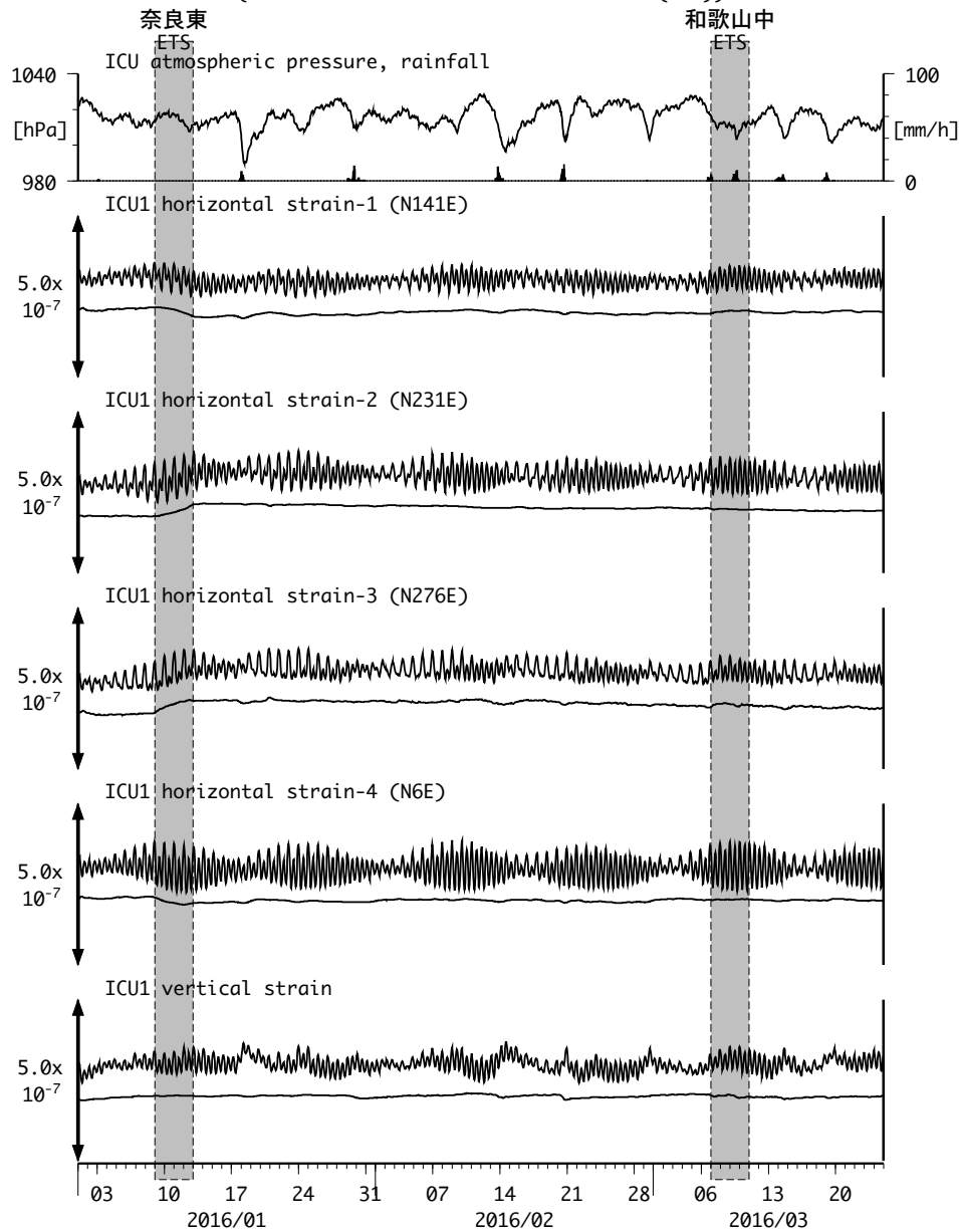
図15 : Crustal strain changes at ICU 熊野磯崎 (時間値) (2016/01/01 00:00 - 2016/03/25 00:00 (JST))
