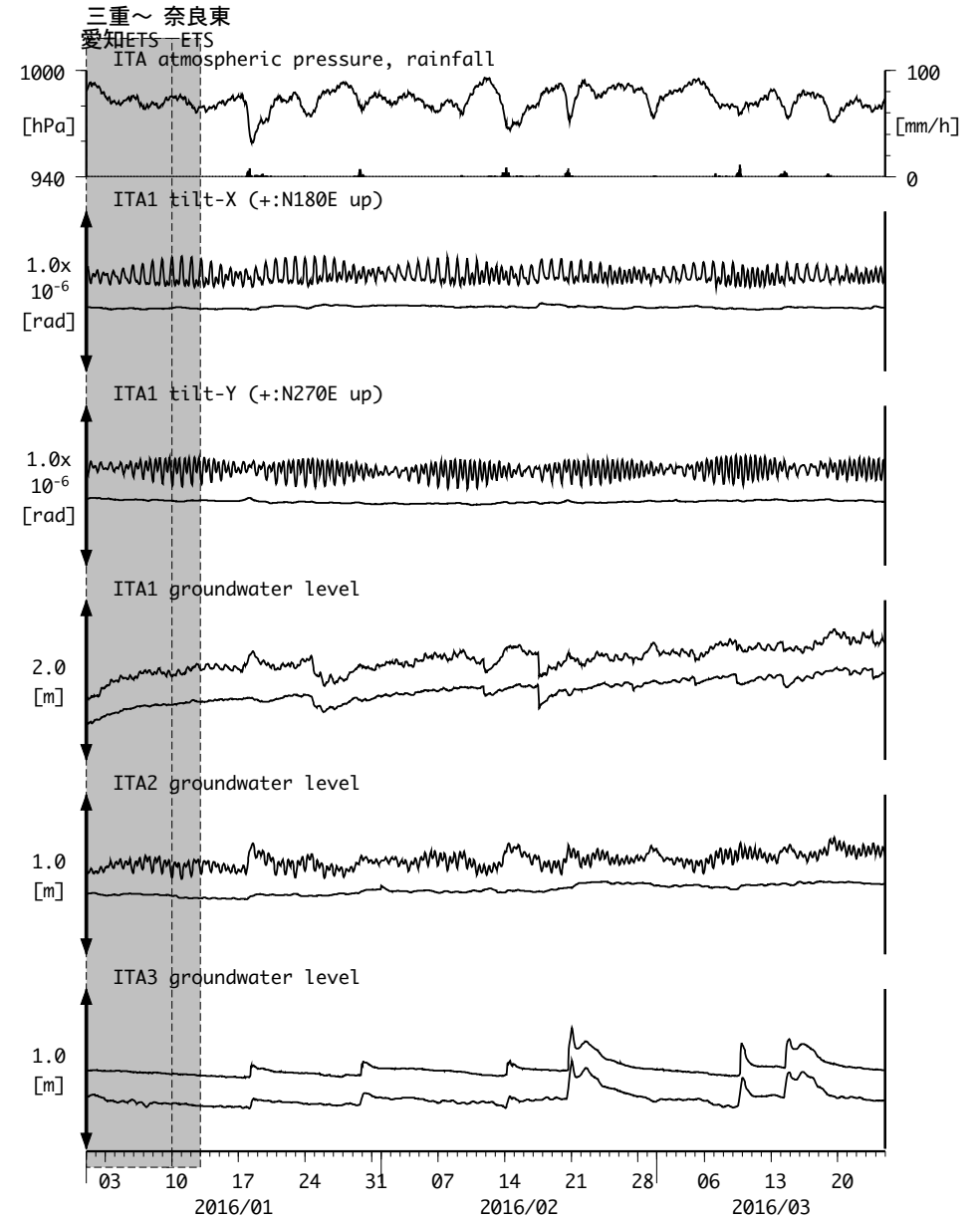
図12: Tilt and groundwater level changes at ITA 松阪飯高 (時間値) (2016/01/01 00:00 - 2016/03/25 00:00 (JST))
