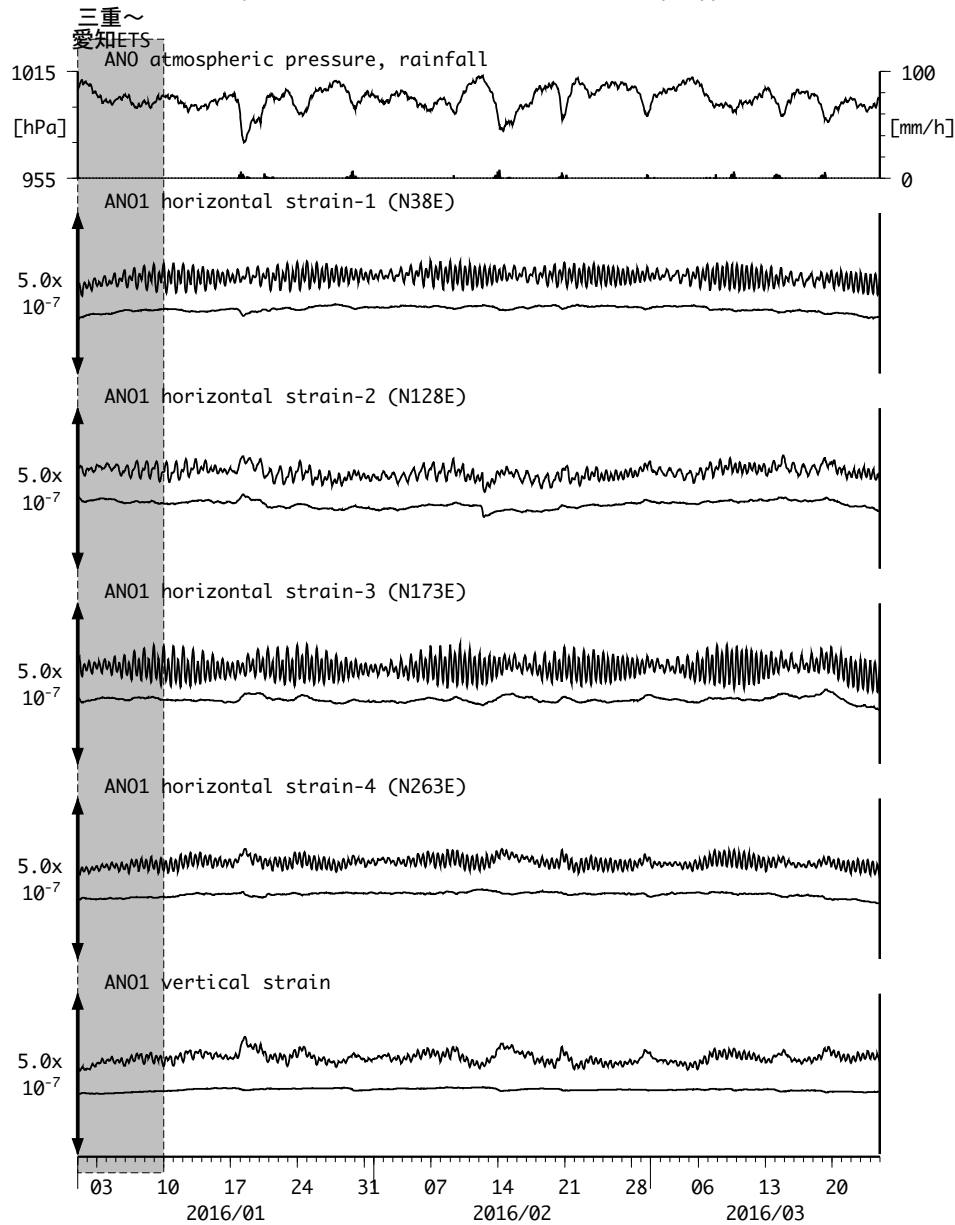
図9 : Crustal strains changes at ANO 津安濃 (時間値) (2016/01/01 00:00 - 2016/03/25 00:00 (JST))
