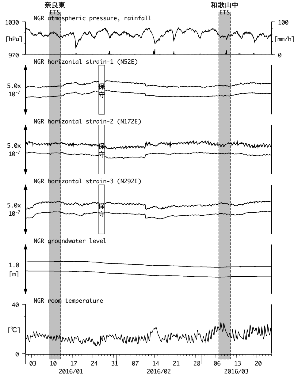
図21: Crustal strain and groundwater level changes at 岩出東坂本（時間値） (2016/01/01 00:00 - 2016/03/25 00:00 (JST))
