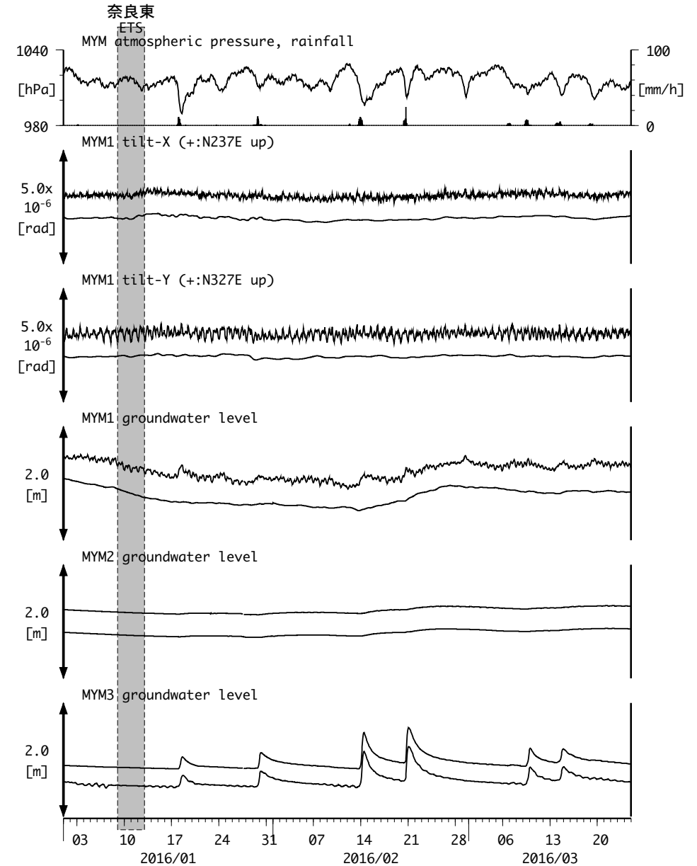
図14 : Tilt and groundwater level changes at MYM 紀北海山 (時間値) (2016/01/01 00:00 - 2016/03/25 00:00 (JST))
