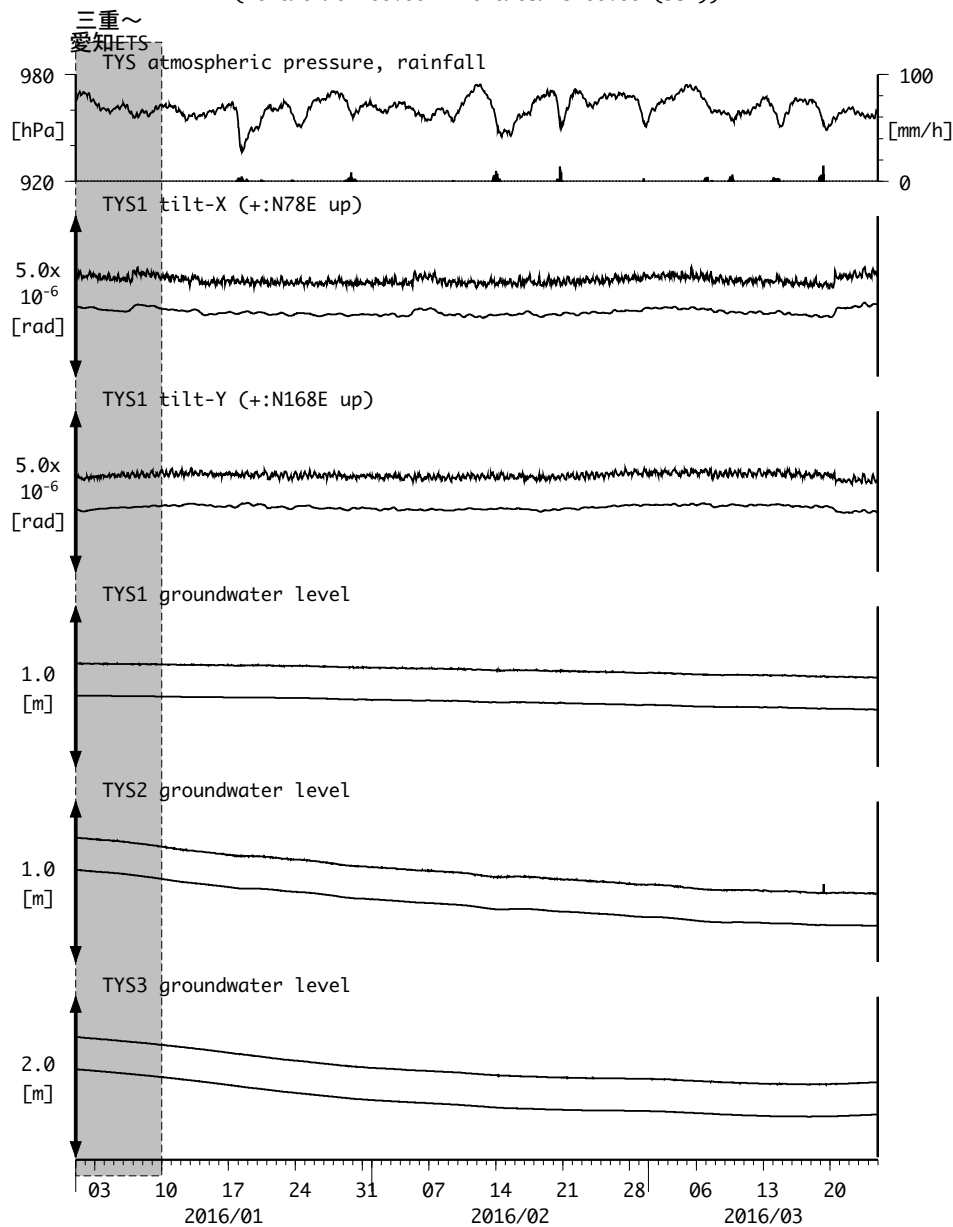
図3: Tilt and groundwater level changes at TYS 豊田神殿 (時間値) (2016/01/01 00:00 - 2016/03/25 00:00 (JST))
