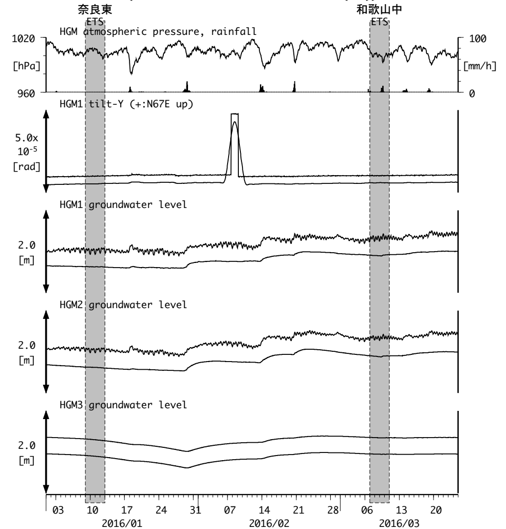
図18: Tilt and groundwater level changes at HGM 田辺本宮 (時間値) (2016/01/01 00:00 - 2016/03/25 00:00 (JST))
