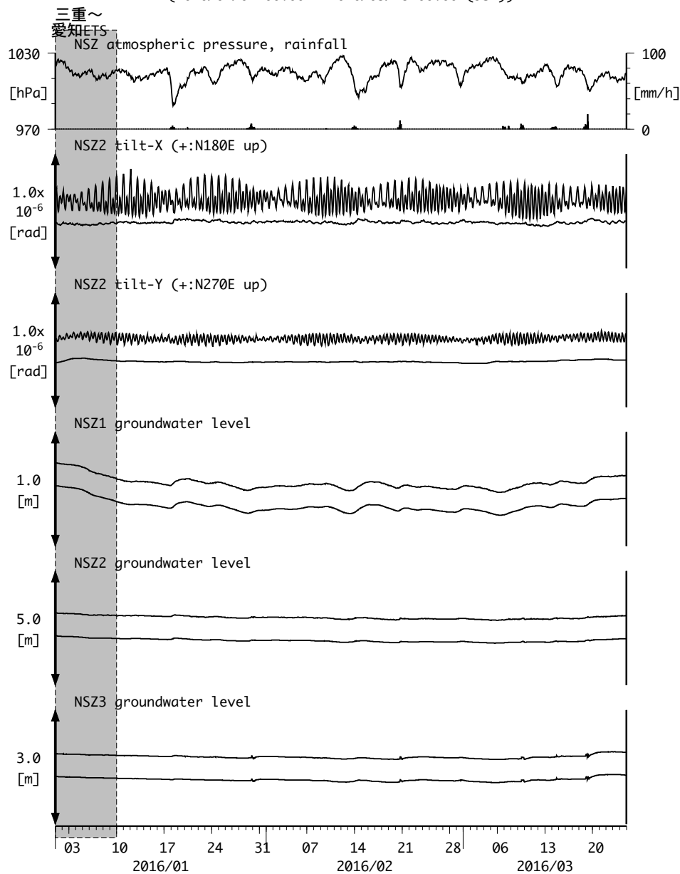
図5: Tilt and groundwater level changes at NSZ 西尾善明 (時間値) (2016/01/01 00:00 - 2016/03/25 00:00 (JST))
