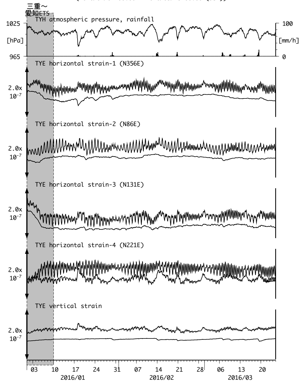
図6: Crustal strain changes at TYE 豊橋多米 (時間値) (2016/01/01 00:00 - 2016/03/25 00:00 (JST))
