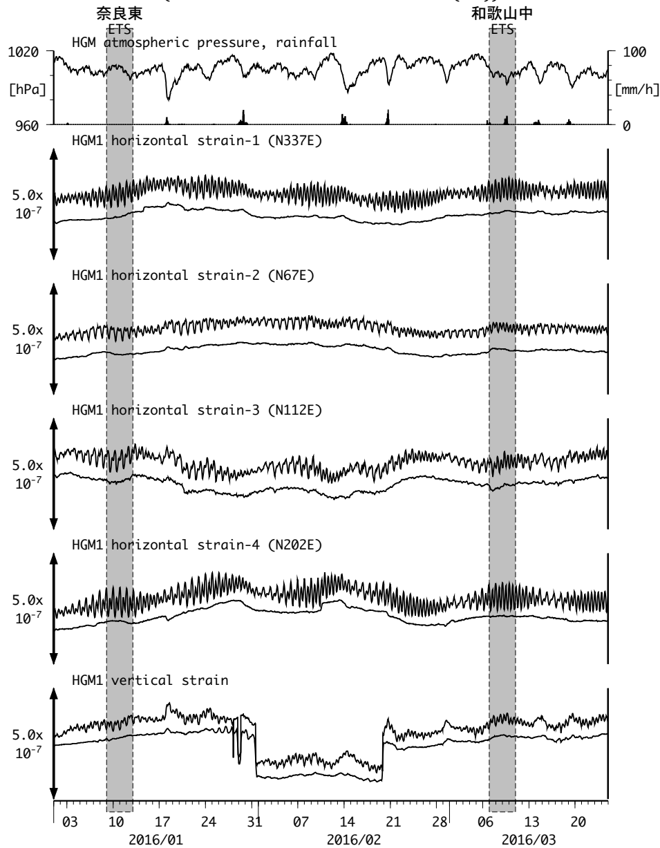
図17: Crustal strains changes at HGM 田辺本宮 (時間値) (2016/01/01 00:00 - 2016/03/25 00:00 (JST))
