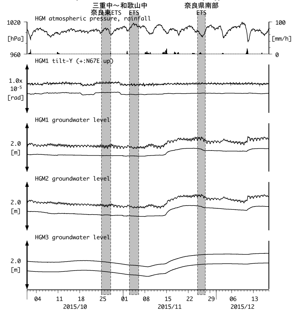
図18: Tilt and groundwater level changes at HGM 田辺本宮 (時間値)
