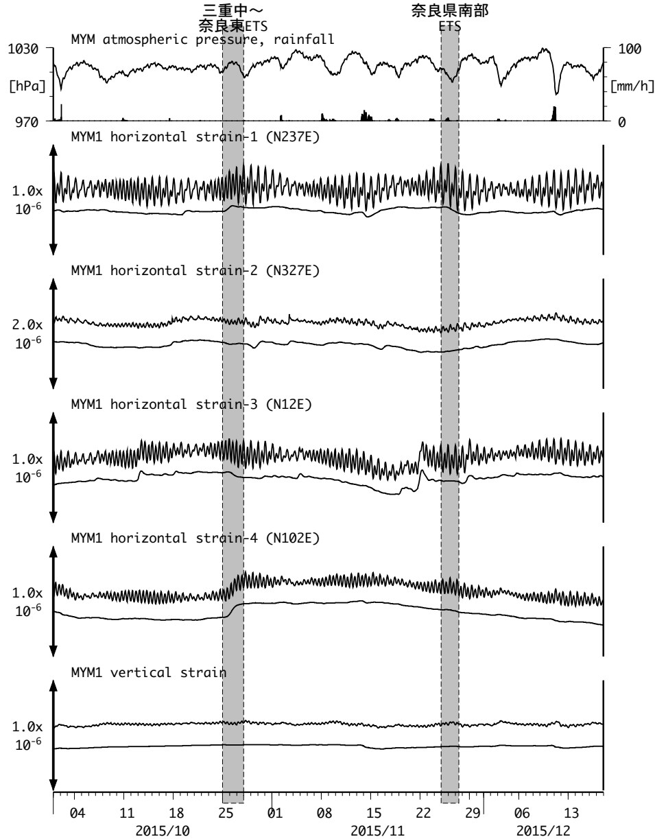
図13 : Crustal strain changes at MYM 紀北海山 (時間値)
