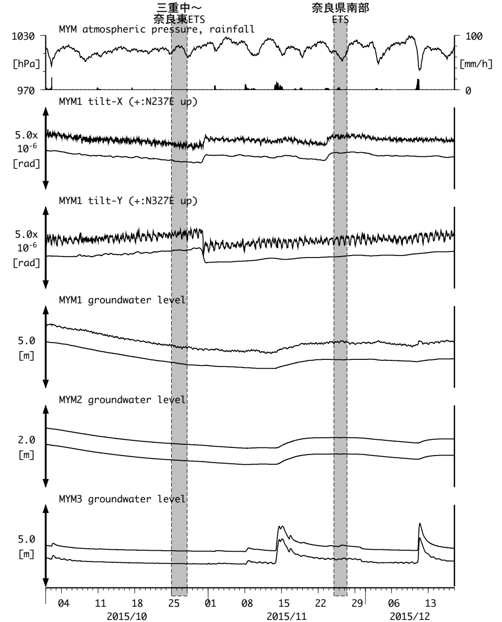
図14 : Tilt and groundwater level changes at MYM 紀北海山 (時間値)
