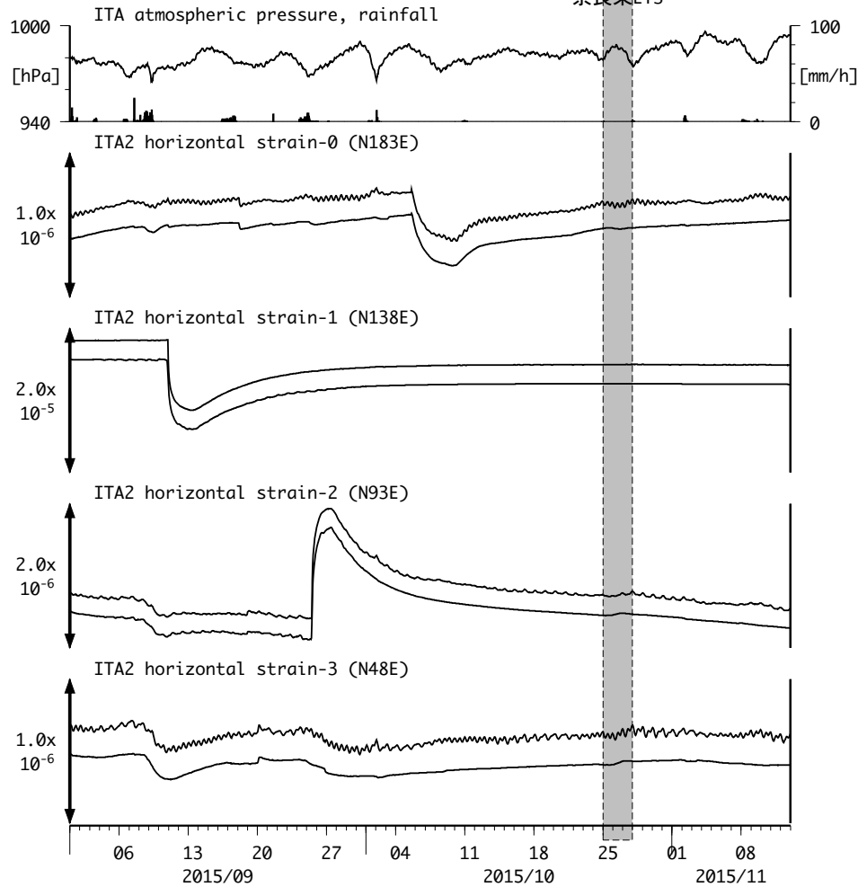
図11: Crustal strain changes at ITA 松阪飯高 (時間値) (2015/09/01 00:00 - 2015/11/13 00:00 (JST))
