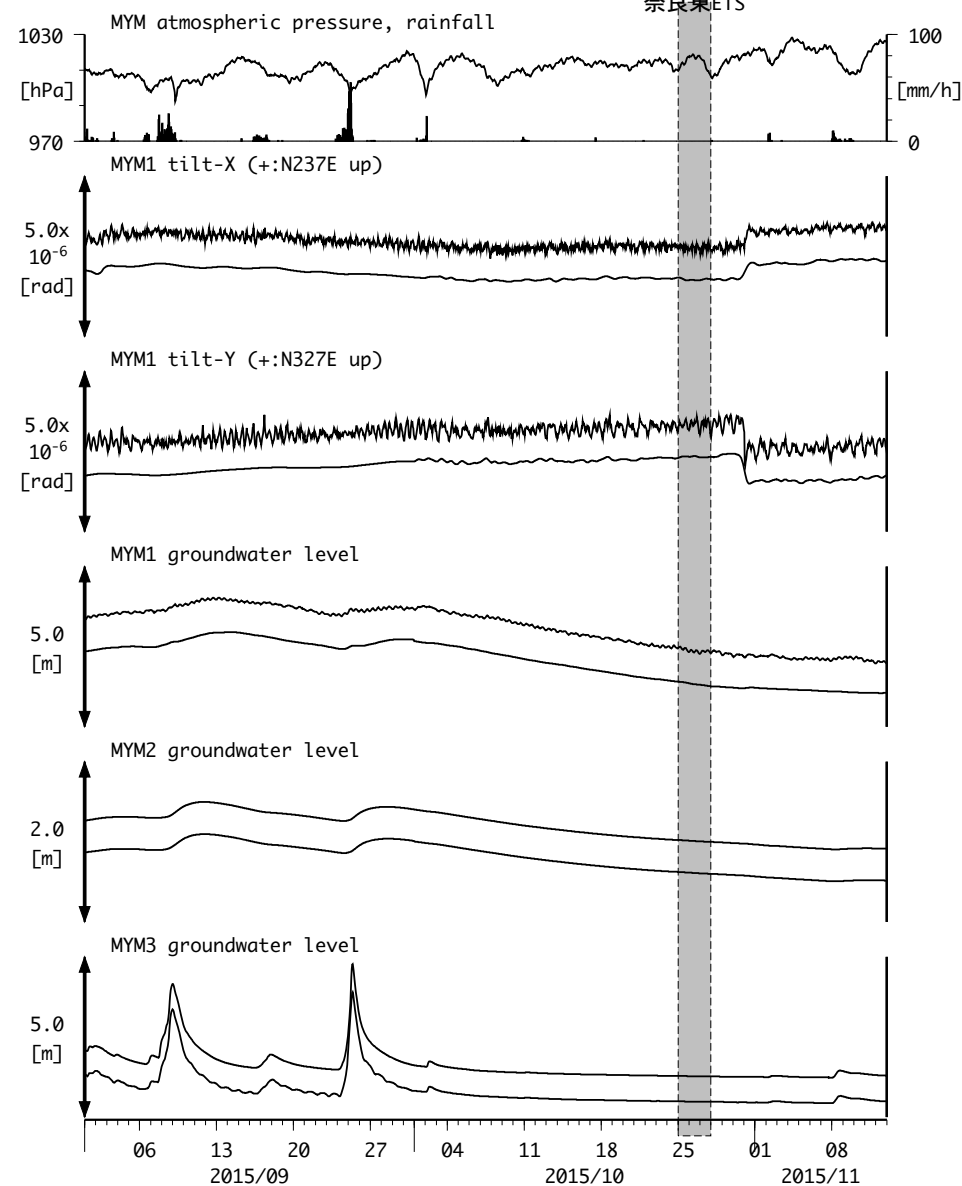
図14 : Tilt and groundwater level changes at MYM 紀北海山 (時間値) (2015/09/01 00:00 - 2015/11/13 00:00 (JST))
