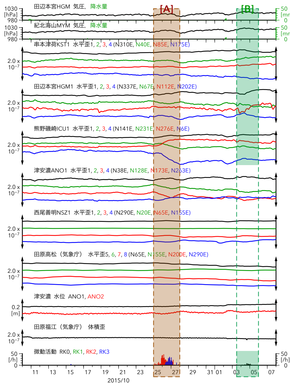
図25：紀伊半島・東海地方における歪・地下水・傾斜観測結果 (2015/10/10 00:00 - 2015/11/8 00:00 (JST))
