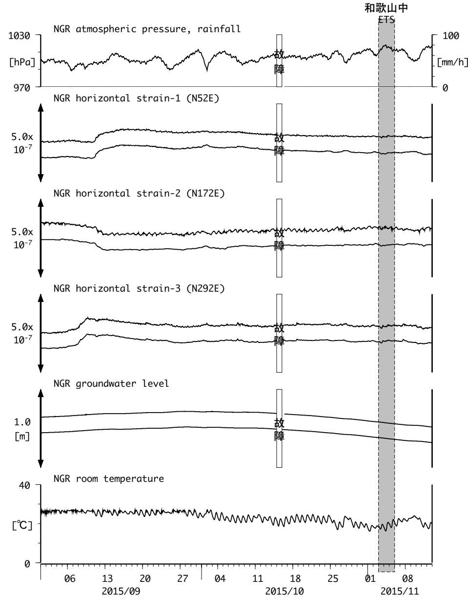
図21: Crustal strain and groundwater level changes at 岩出東坂本（時間値） (2015/09/01 00:00 - 2015/11/13 00:00 (JST))
