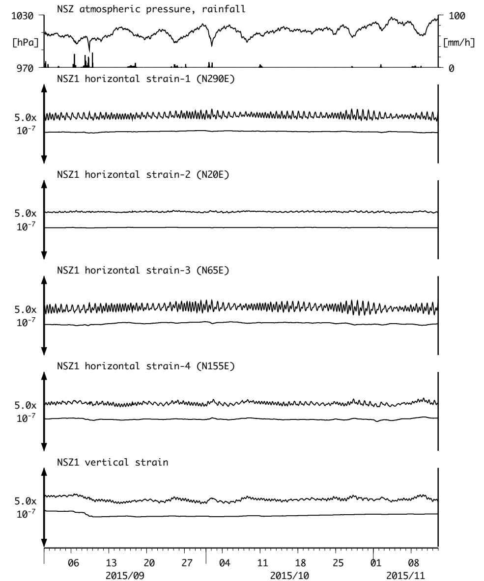
図4: Crustal strains changes at NSZ 西尾善明 (時間値) (2015/09/01 00:00 - 2015/11/13 00:00 (JST))
