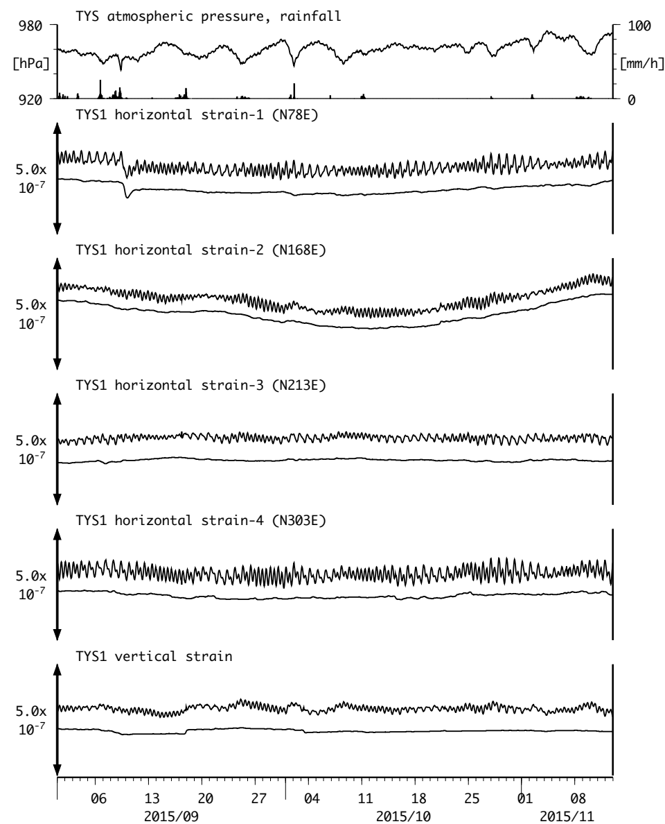
図2: Crustal strains changes at TYS 豊田神殿 (時間値) (2015/09/01 00:00 - 2015/11/13 00:00 (JST))
