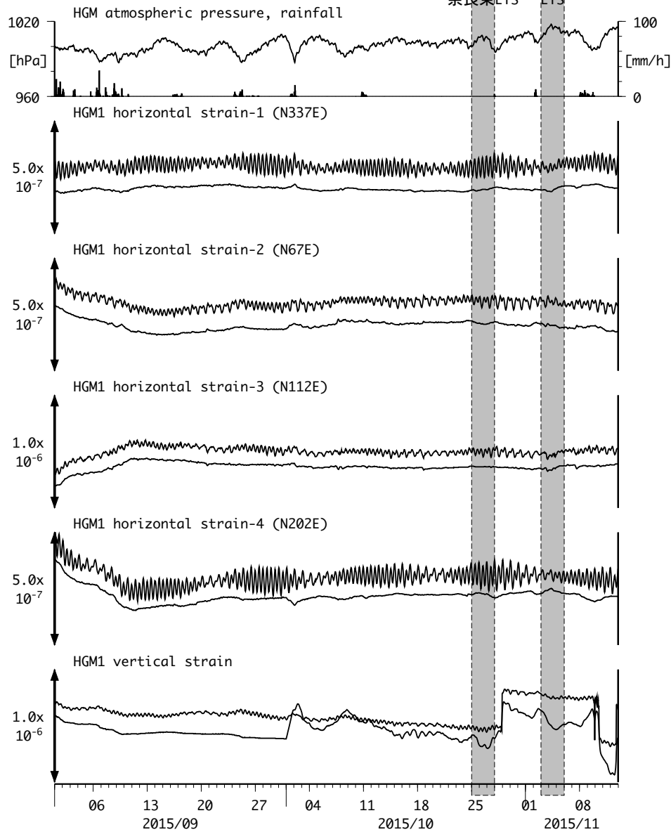
図17: Crustal strains changes at HGM 田辺本宮 (時間値) (2015/09/01 00:00 - 2015/11/13 00:00 (JST))
