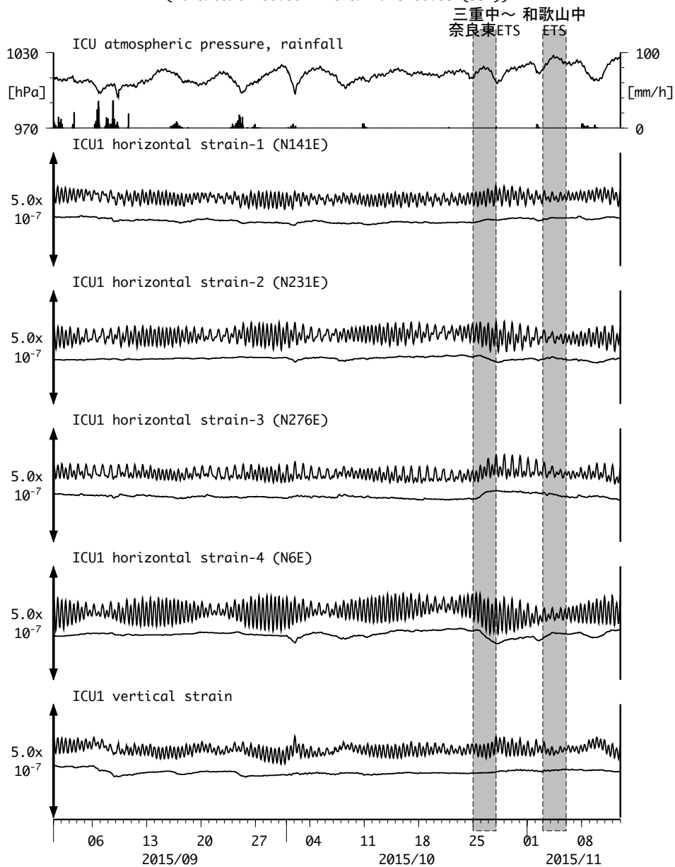
図15 : Crustal strain changes at ICU 熊野磯崎 (時間値) (2015/09/01 00:00 - 2015/11/13 00:00 (JST))
