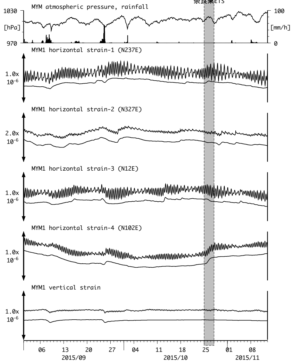
図13 : Crustal strain changes at MYM 紀北海山 (時間値) (2015/09/01 00:00 - 2015/11/13 00:00 (JST))
