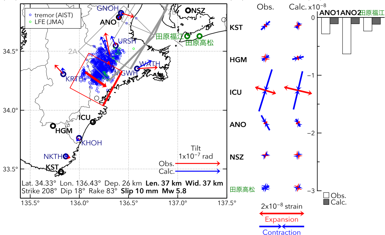
図26：2015/10/25-27の歪・傾斜・地下水変化（図25赤色[A]）を説明する断層モデル。
