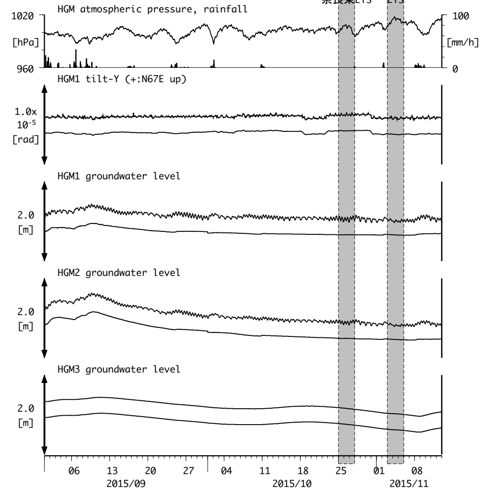
図18: Tilt and groundwater level changes at HGM 田辺本宮 (時間値) (2015/09/01 00:00 - 2015/11/13 00:00 (JST))
