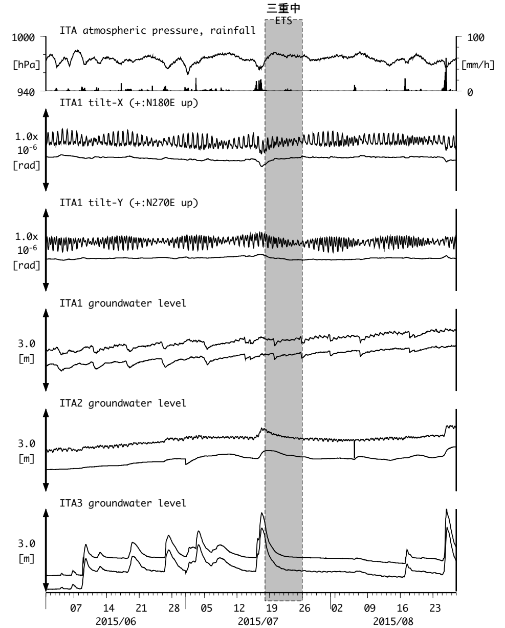
図12: Tilt and groundwater level changes at ITA 松阪飯高 (時間値) (2015/06/01 00:00 - 2015/08/28 00:00 (JST))
