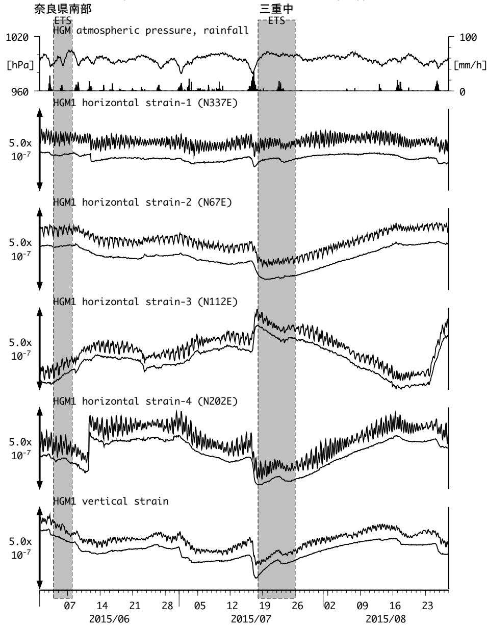
図17: Crustal strains changes at HGM 田辺本宮 (時間値) (2015/06/01 00:00 - 2015/08/28 00:00 (JST))
