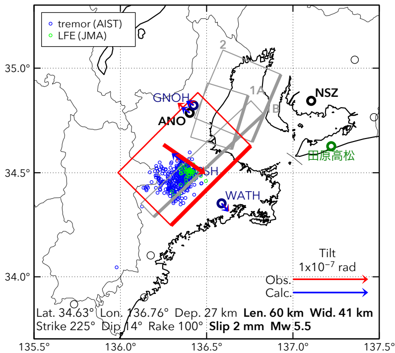
図26：2015/7/18-19の歪・傾斜変化（図25網掛[A1]）を説明する断層モデル。
