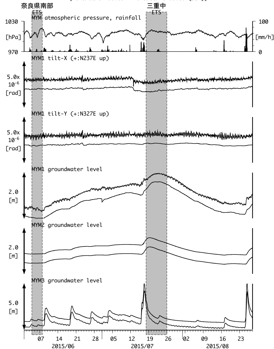
図14 : Tilt and groundwater level changes at MYM 紀北海山 (時間値) (2015/06/01 00:00 - 2015/08/28 00:00 (JST))
