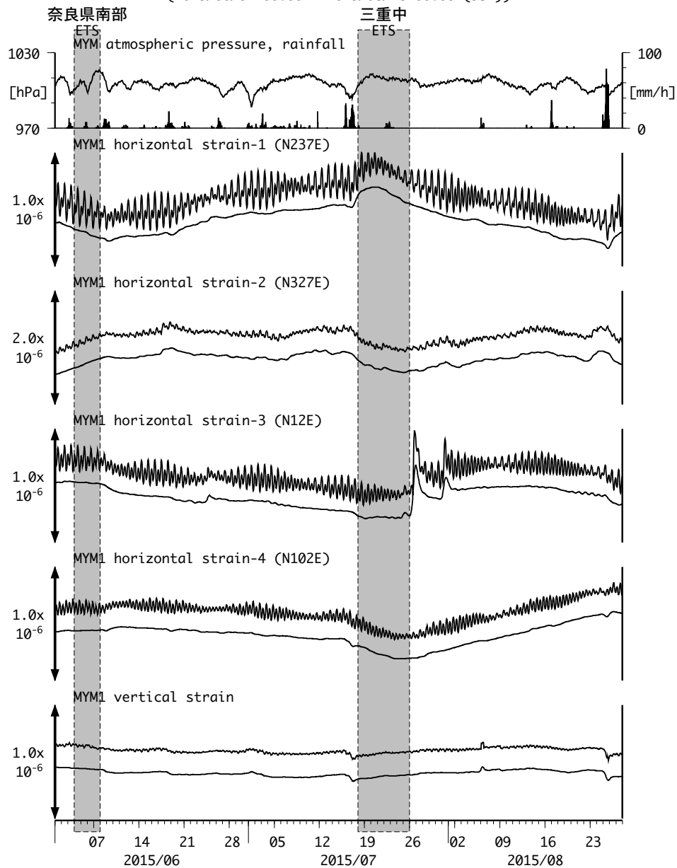
図13 : Crustal strain changes at MYM 紀北海山 (時間値) (2015/06/01 00:00 - 2015/08/28 00:00 (JST))
