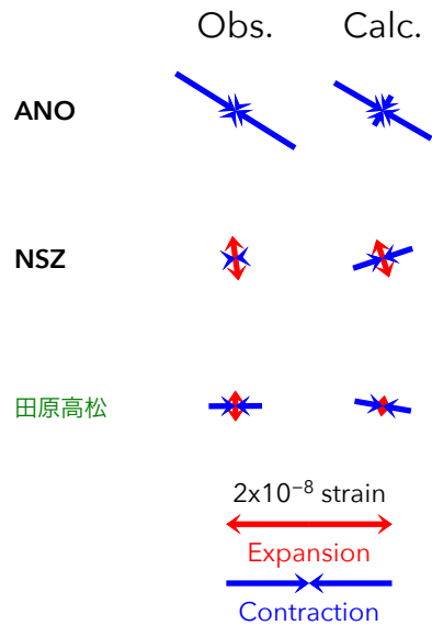
(b2) 主歪の比較
