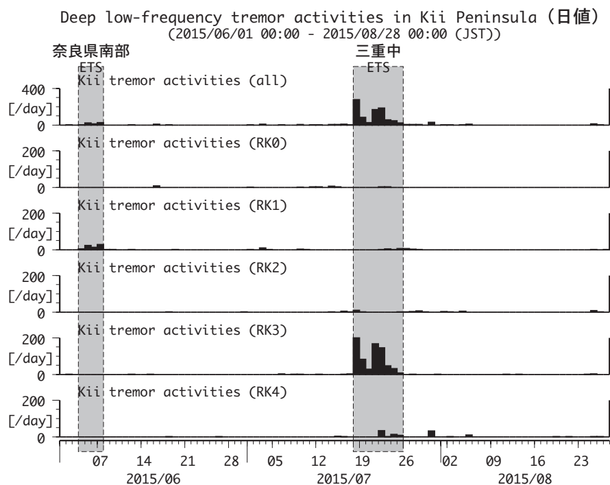
図23 (上段) 紀伊半島における深部低周波微動の時空間分布、(下段) 各領域における発生頻度(日値)。
