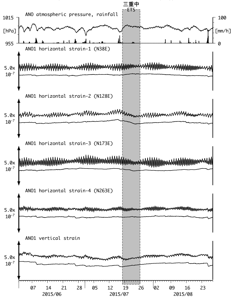
図9 : Crustal strains changes at ANO 津安濃 (時間値) (2015/06/01 00:00 - 2015/08/28 00:00 (JST))
