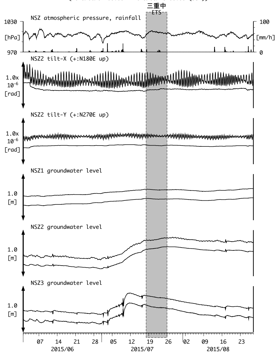
図5: Tilt and groundwater level changes at NSZ 西尾善明 (時間値) (2015/06/01 00:00 - 2015/08/28 00:00 (JST))
