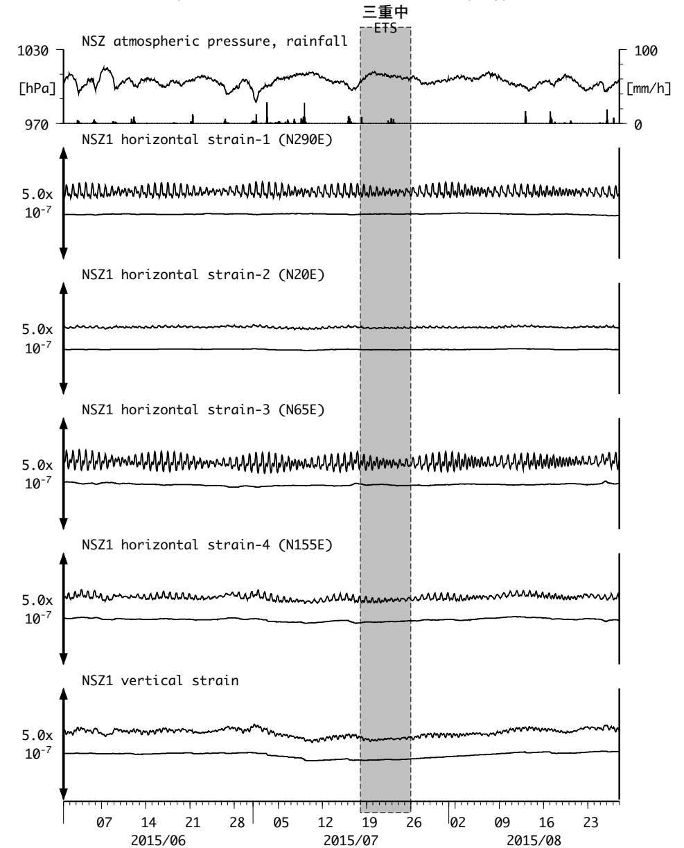
図4: Crustal strains changes at NSZ 西尾善明 (時間値) (2015/06/01 00:00 - 2015/08/28 00:00 (JST))
