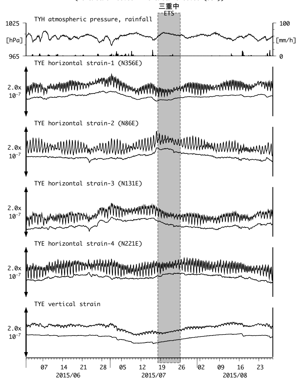
図6: Crustal strain changes at TYE 豊橋多米 (時間値) (2015/06/01 00:00 - 2015/08/28 00:00 (JST))
