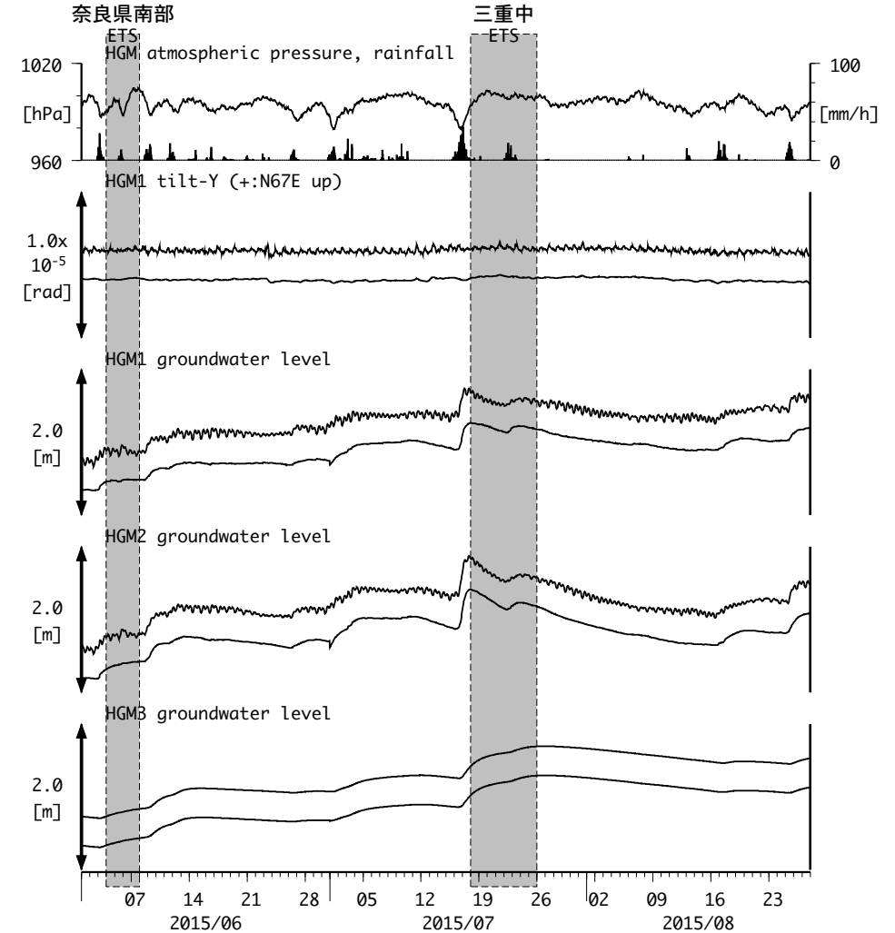
図18: Tilt and groundwater level changes at HGM 田辺本宮 (時間値) (2015/06/01 00:00 - 2015/08/28 00:00 (JST))
