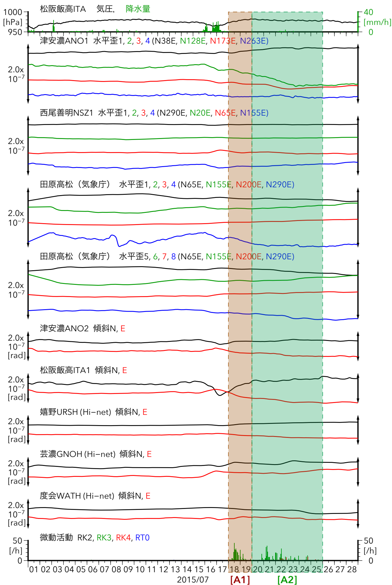
図25：紀伊半島・東海地方における歪・傾斜観測結果 (2015/7/1 00:00 - 2015/7/29 00:00 (JST))
