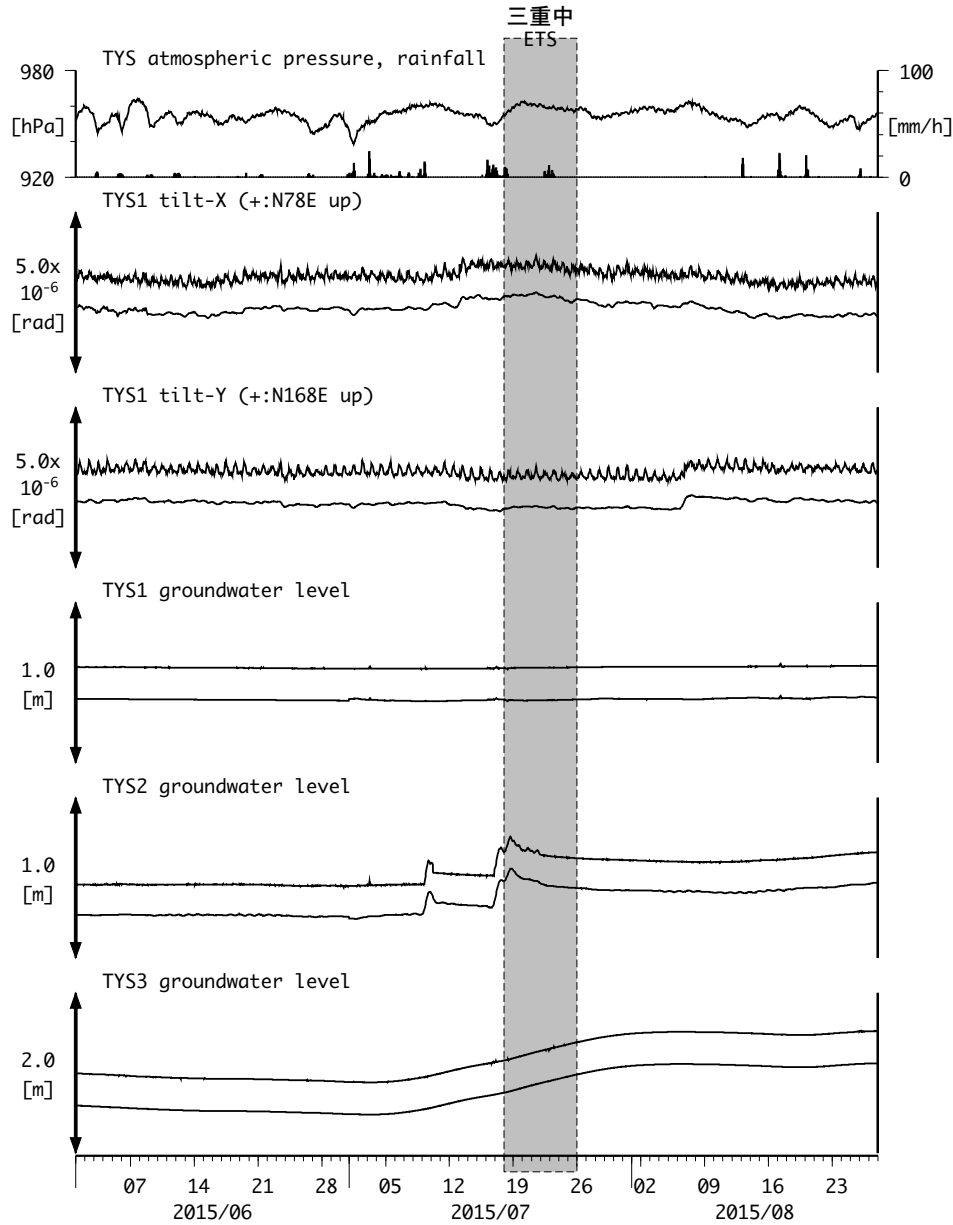
図3: Tilt and groundwater level changes at TYS 豊田神殿 (時間値) (2015/06/01 00:00 - 2015/08/28 00:00 (JST))
