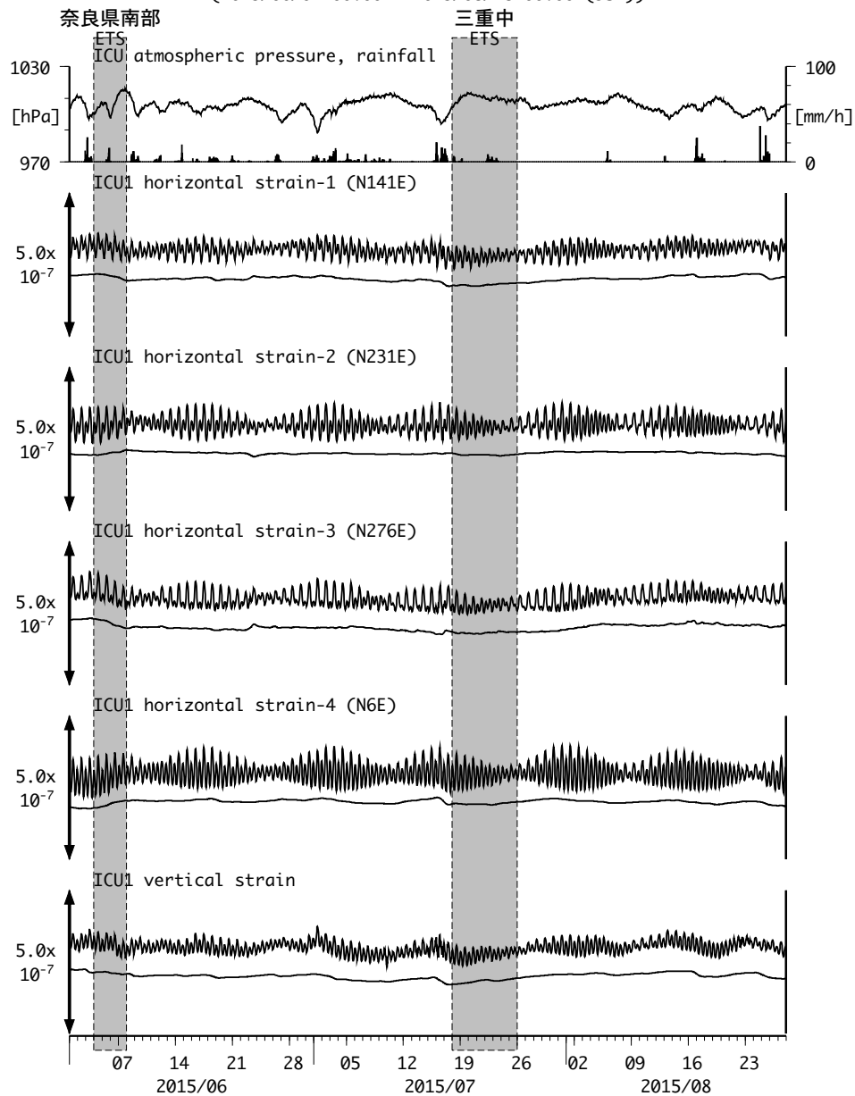
図15 : Crustal strain changes at ICU 熊野磯崎 (時間値) (2015/06/01 00:00 - 2015/08/28 00:00 (JST))
