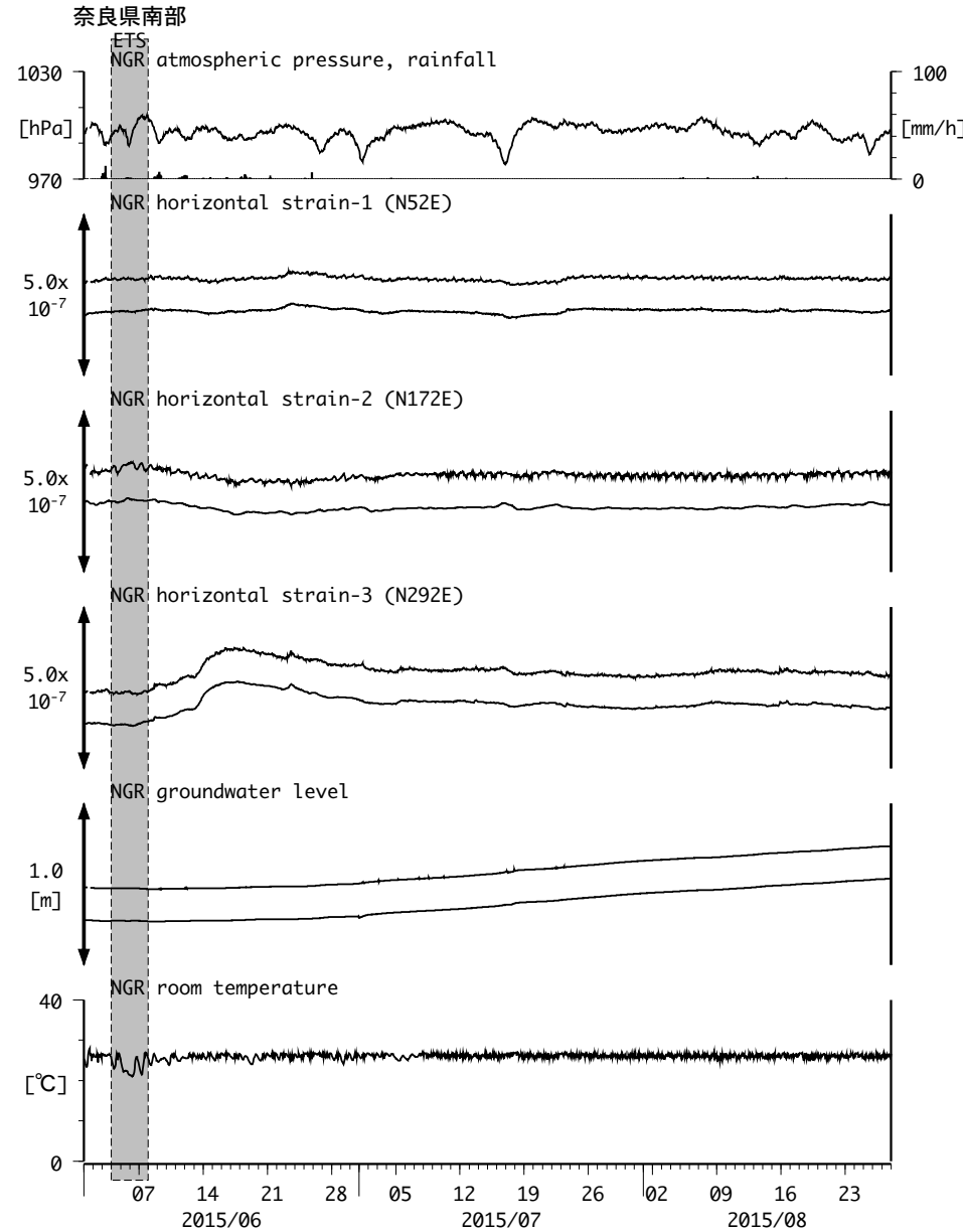
図21: Crustal strain and groundwater level changes at 岩出東坂本（時間値） (2015/06/01 00:00 - 2015/08/28 00:00 (JST))
