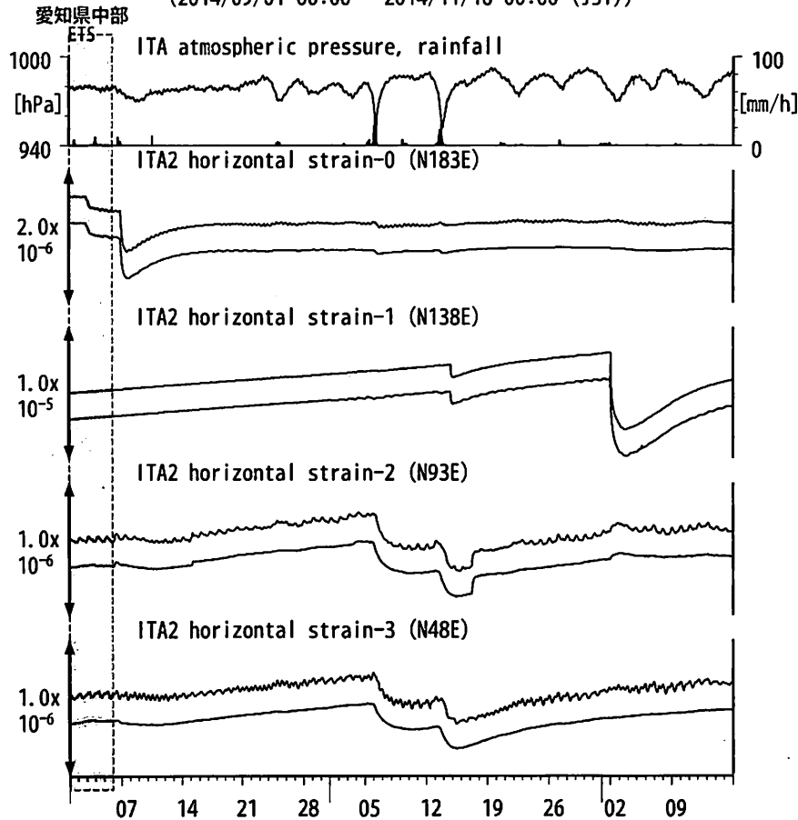
図11: Crustal strain changes at ITA 松阪飯高 (時間値) (2014/09/01 00:00 - 2014/11/16 00:00 (JST))
