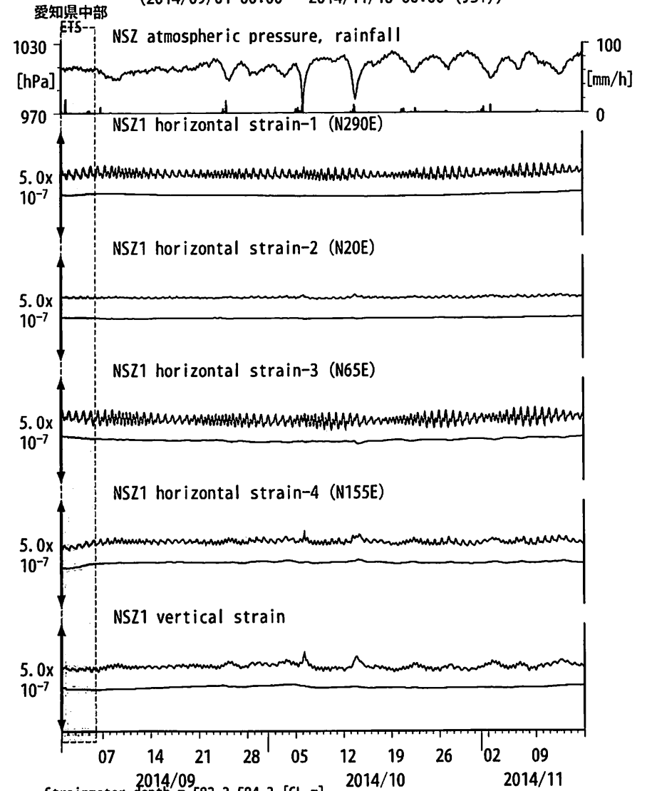
図4: Crustal strains changes at NSZ 西尾善明 (時間値) (2014/09/01 00:00 - 2014/11/16 00:00 (JST))
