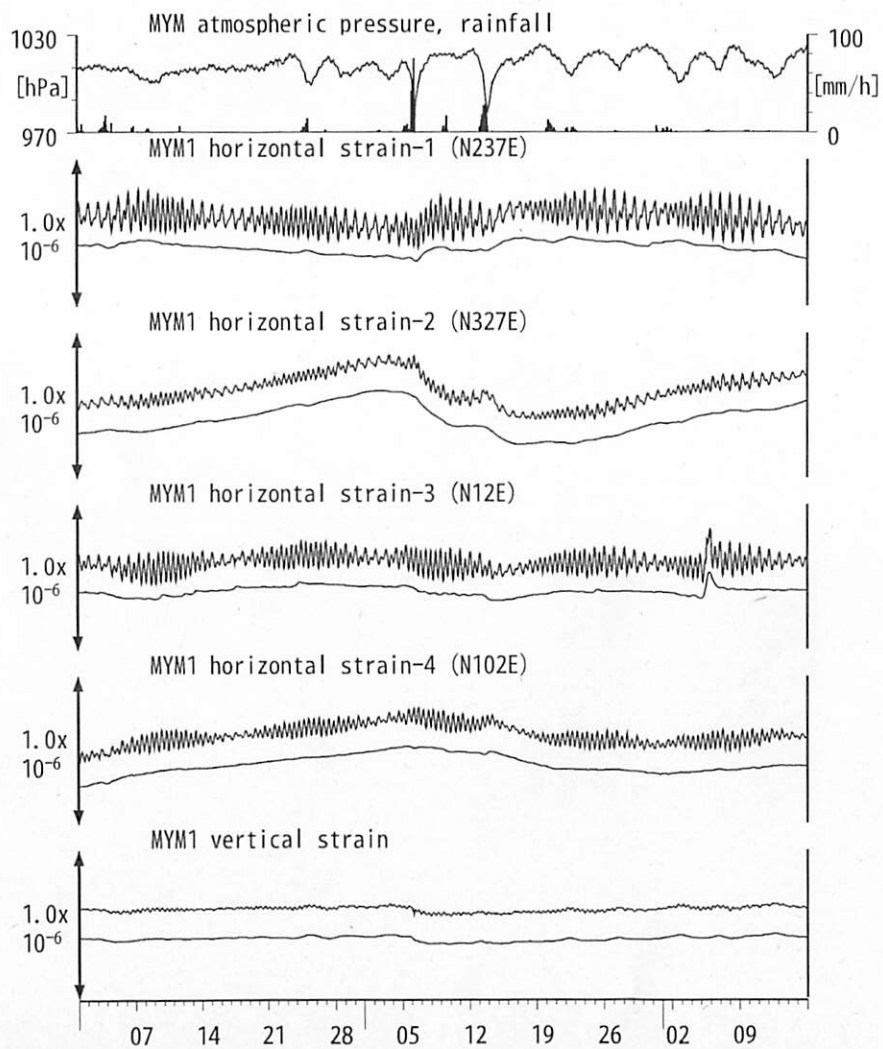
図13: Crustal strain changes at MYM 紀北海山 (時間値) (2014/09/01 00:00 - 2014/11/16 00:00 (JST))
