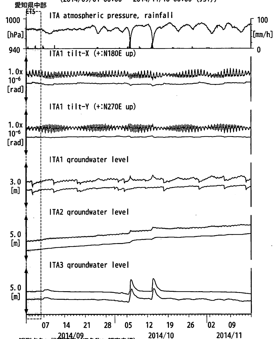
図12: Tilt and groundwater level changes at ITA 松阪飯高 (時間値) (2014/09/01 00:00 - 2014/11/16 00:00 (JST))
