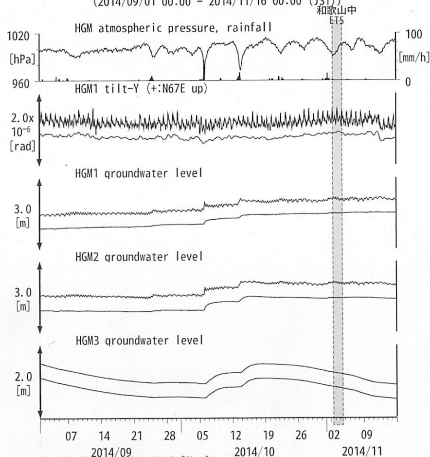
図18: Tilt and groundwater level changes at HGM 田辺本宮 (時間値) (2014/09/01 00:00 - 2014/11/16 00:00 (JST))
