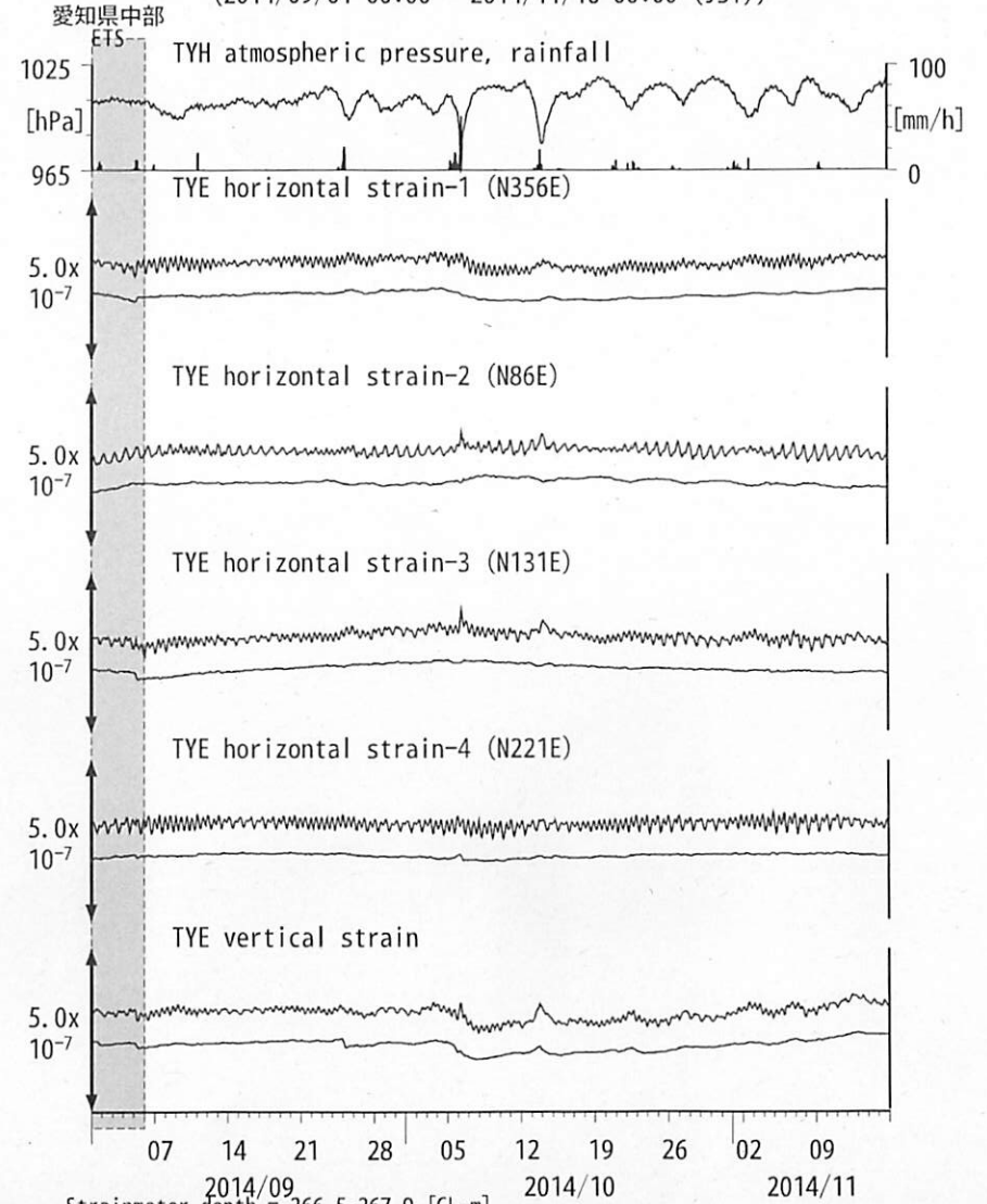
図6: Crustal strain changes at TYE 豊橋多米 (時間値) (2014/09/01 00:00 - 2014/11/16 00:00 (JST))
