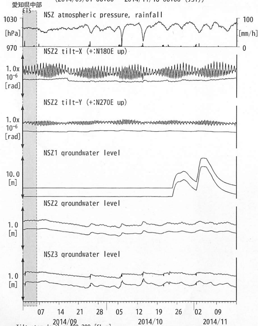
図5: Tilt and groundwater level changes at NSZ 西尾善明 (時間値) (2014/09/01 00:00 - 2014/11/16 00:00 (JST))
