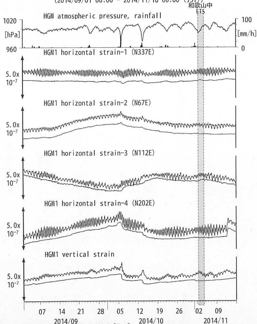
図17: Crustal strains changes at HGM 田辺本宮 (時間値) (2014/09/01 00:00 - 2014/11/16 00:00 (JST))
