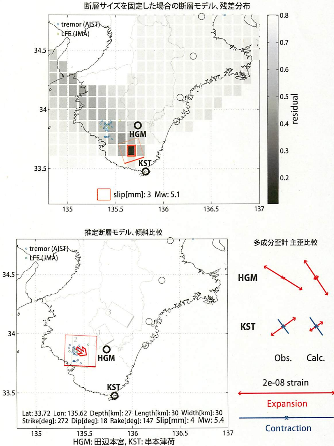
図26: (上段)プレート境界面上のパッチ(断層面)をすべらせた際の、歪・傾斜の観測値と計算値の残差分布図。断層面サイズは固定(20x20km)。赤色矩形は最小残差の断層面を表す。このパッチのすべり量、Mwを下部に示している。
