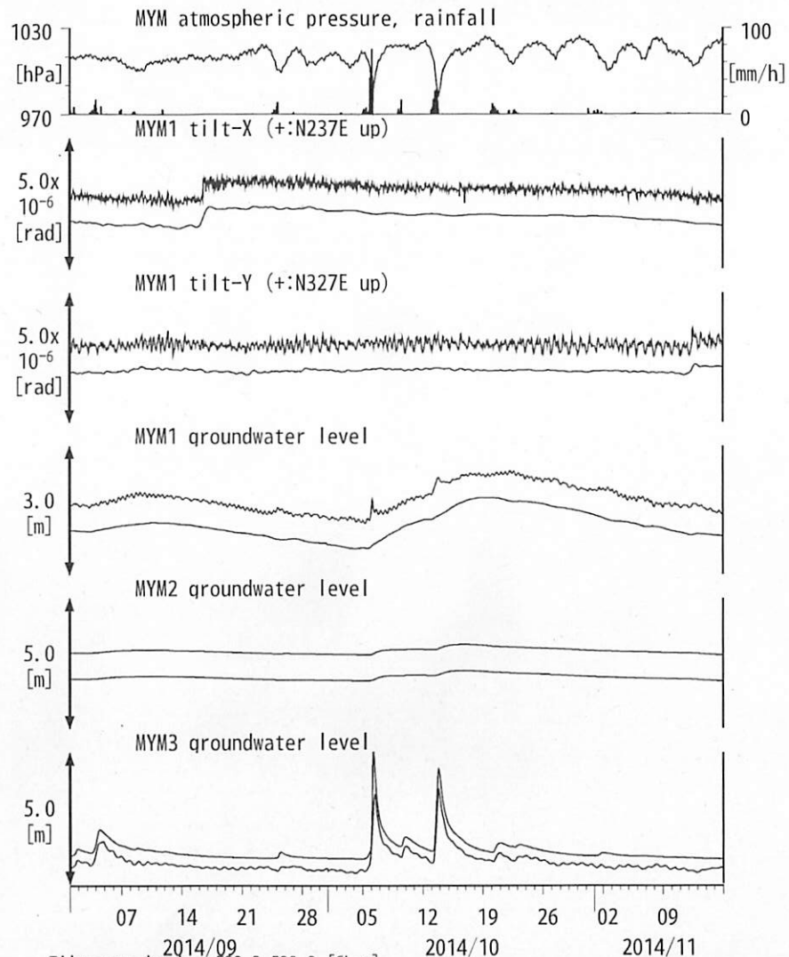
図14: Tilt and groundwater level changes at MYM 紀北海山 (時間値) (2014/09/01 00:00 - 2014/11/16 00:00 (JST))
