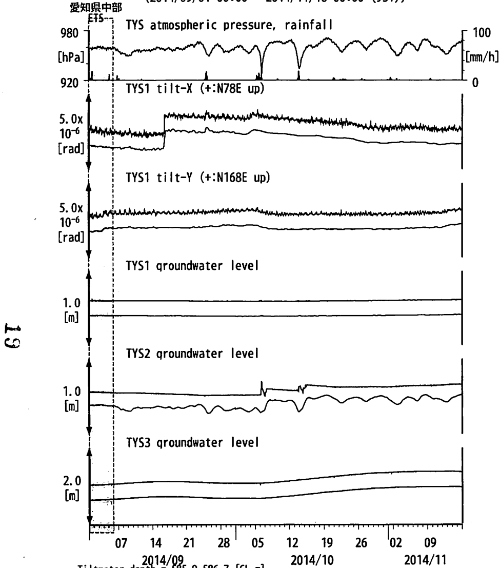
図3: Tilt and groundwater level changes at TYS 豊田神殿 (時間値) (2014/09/01 00:00 - 2014/11/16 00:00 (JST))
