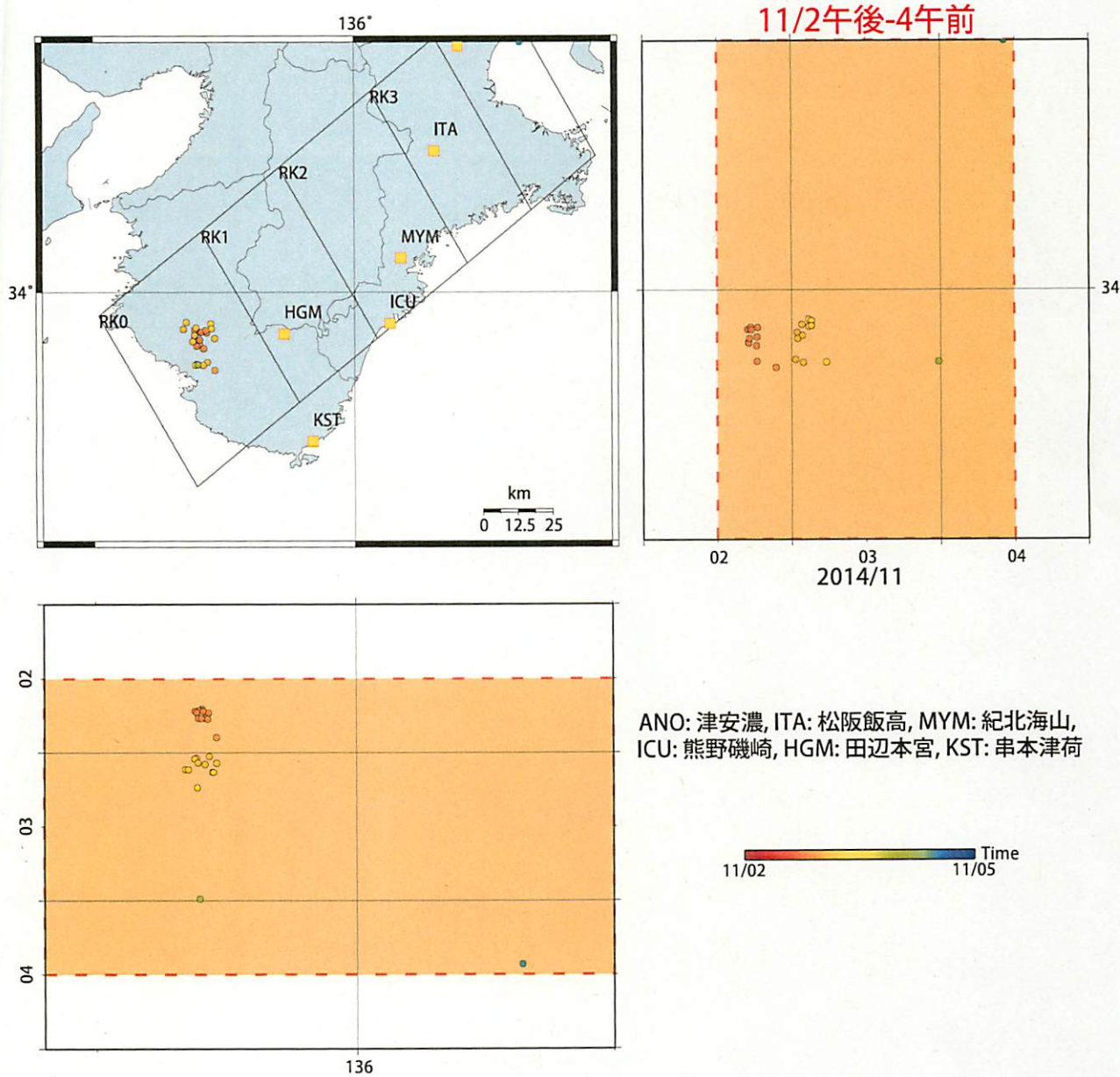
図24: 2014/11/2 0:00 - 11/5 0:00 における紀伊半島周辺の深部低周波微動の時空間分布図。 エンベロープ相関法により決定。
