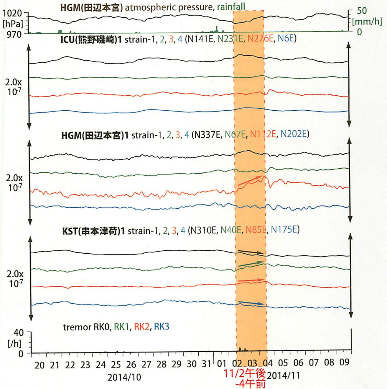
図25: 紀伊半島における歪観測結果 (2014/10/20 00:00 - 2014/11/10 00:00 (JST))
