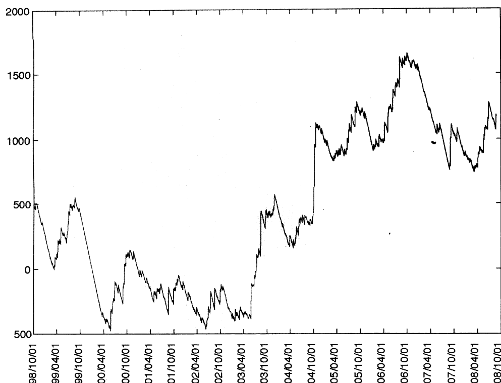
榛原観測井 降雨量の積算からトレンド除去後のグラフ (mm) (1998. 10. 1-2008. 08. 28)
