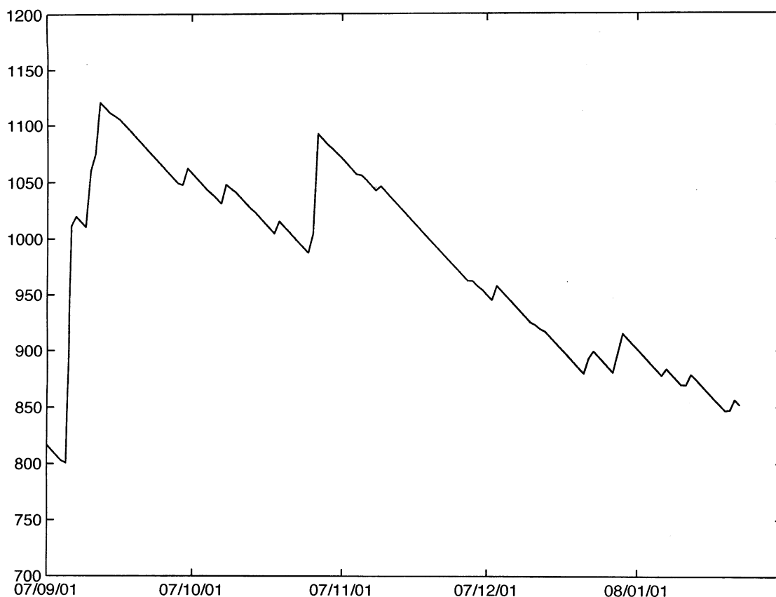
榛原観測井 降雨量の積算からトレンド除去後のグラフ (mm) (2007. 9. 1-2008. 1. 22)
