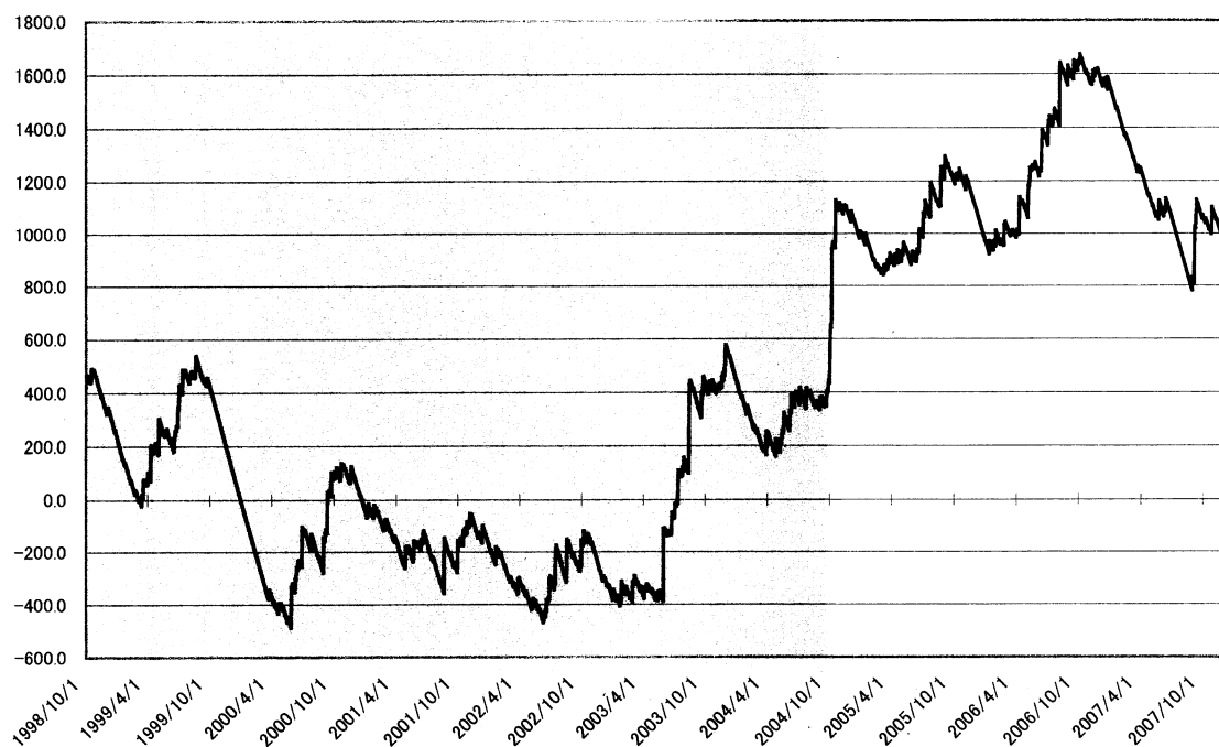
榛原観測井 降雨量の積算からトレンド除去後のグラフ (mm) (1998. 10. 1-2007. 12. 19)
