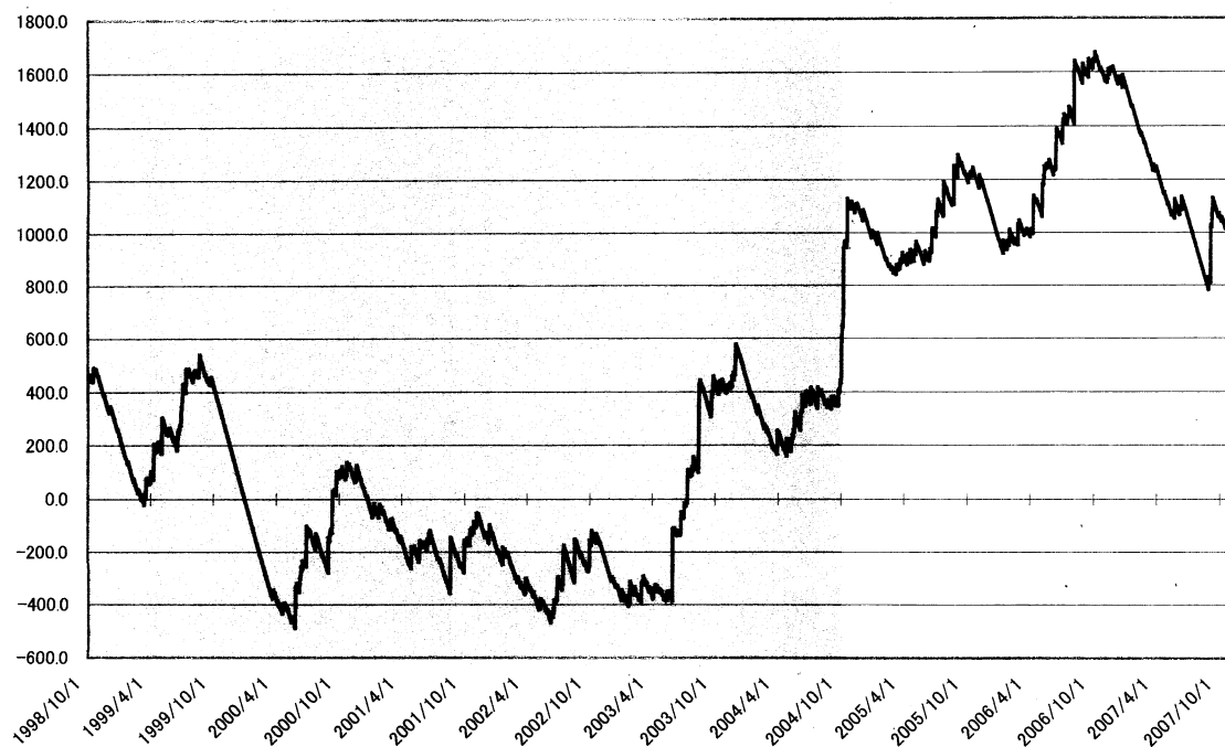
榛原観測井 降雨量の積算からトレンド除去後のグラフ (mm) (1998. 10. 1~2007. 11. 20)
