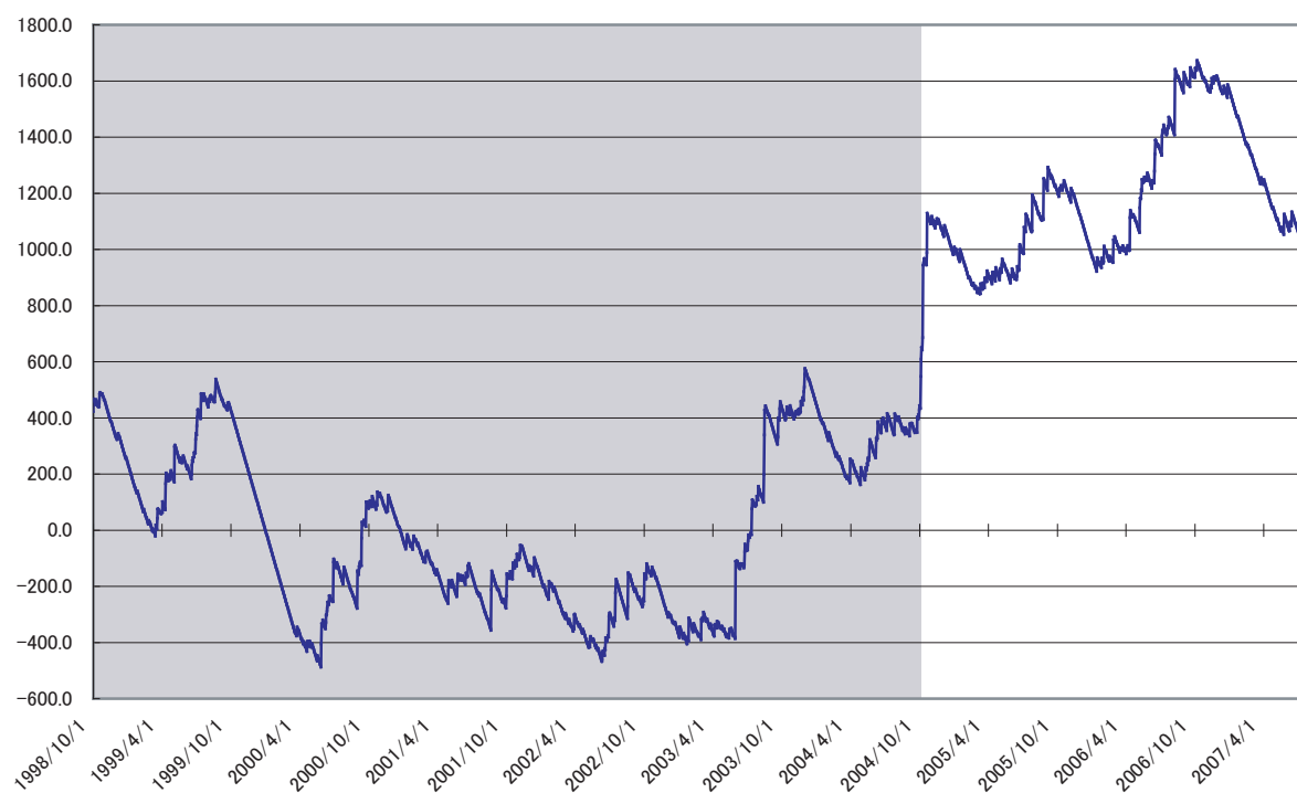
榛原観測井 降雨量の積算からトレンド除去後のグラフ (mm) (1998. 10. 1-2007. 7. 25)
