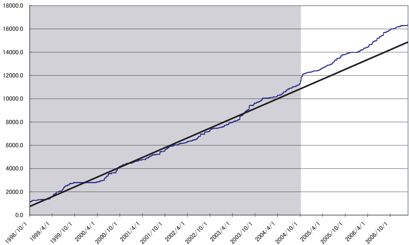
榛原の降雨量の積算グラフ (1998. 10. 1-2007. 2. 21) (mm)
