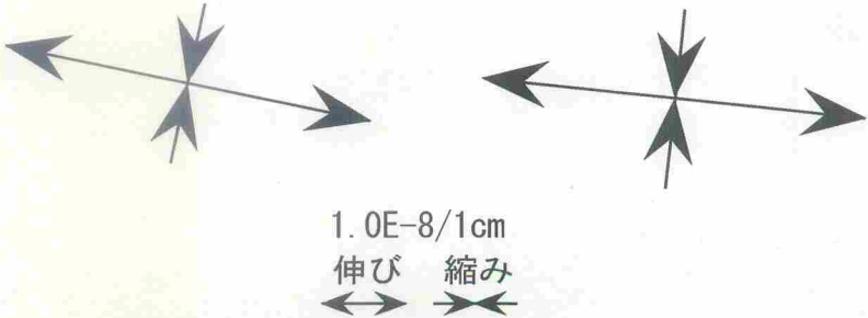
豊橋東観測点の 歪N356E, N131E, N221E から推定した主歪場
