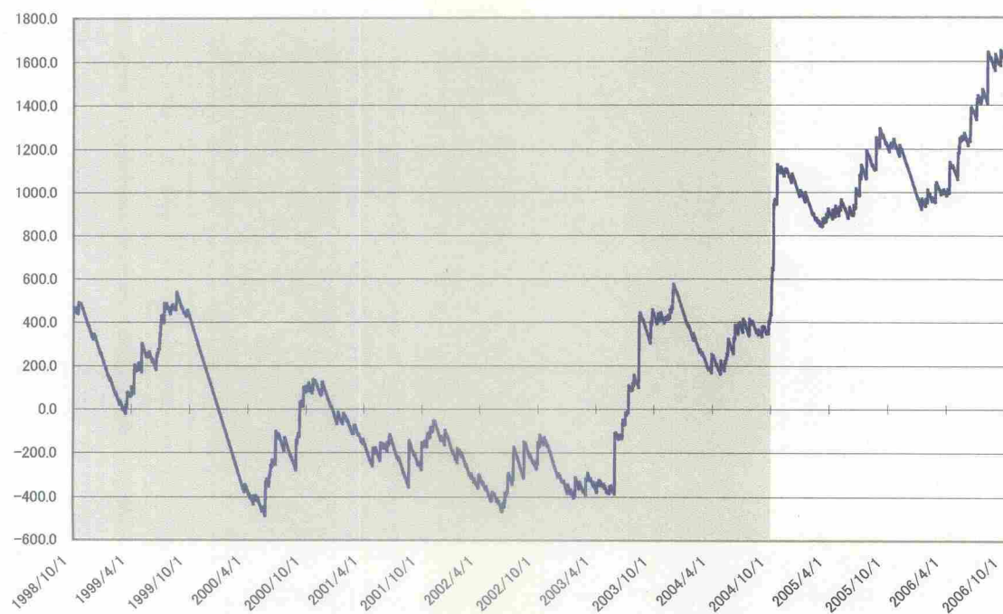
榛原観測井 降雨量の積算からトレンド除去後のグラフ (mm) (1998. 10. 1-2006. 10. 25)
