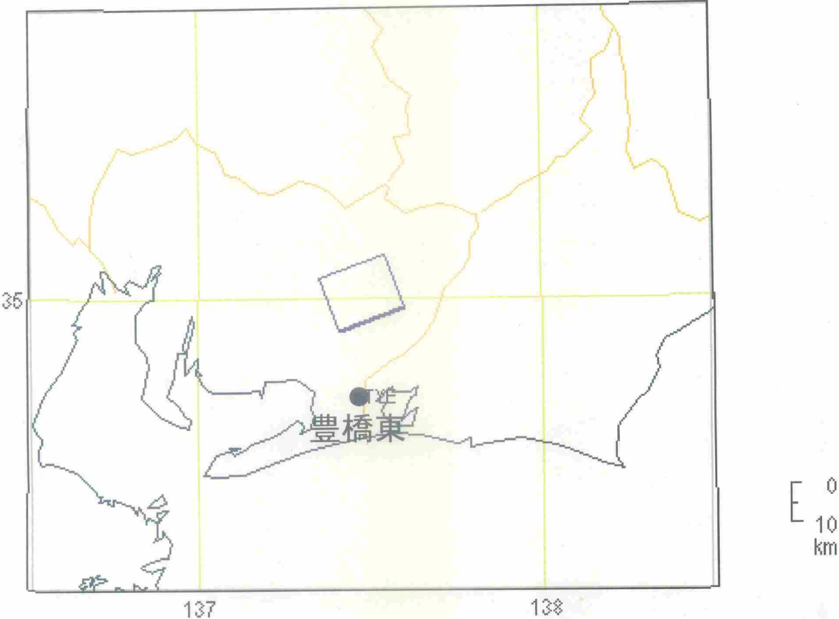
短期的スロースリップモデルと豊橋東観測点の位置
