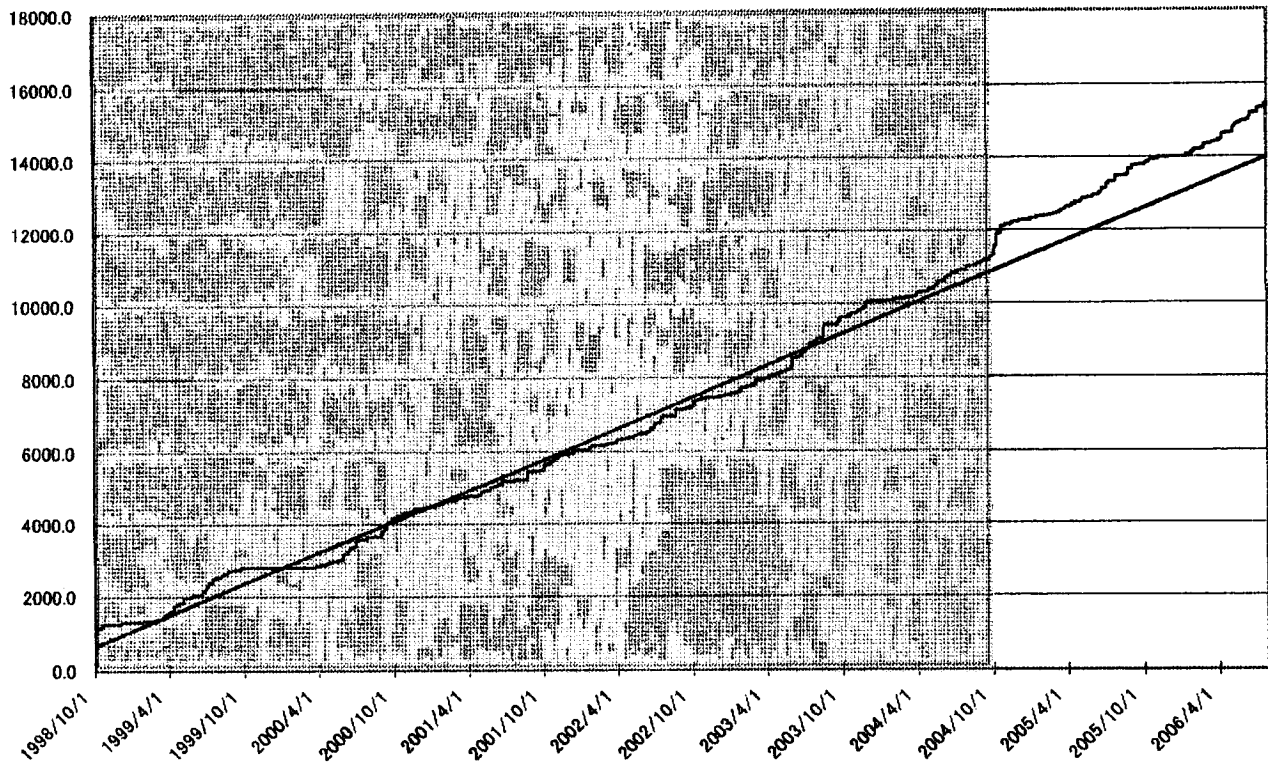
榛原の降雨量の積算グラフ (1998. 10. 1-2006. 7. 25) (mm) (線形近似区間 : 1998. 10/1-2004/9/30)
