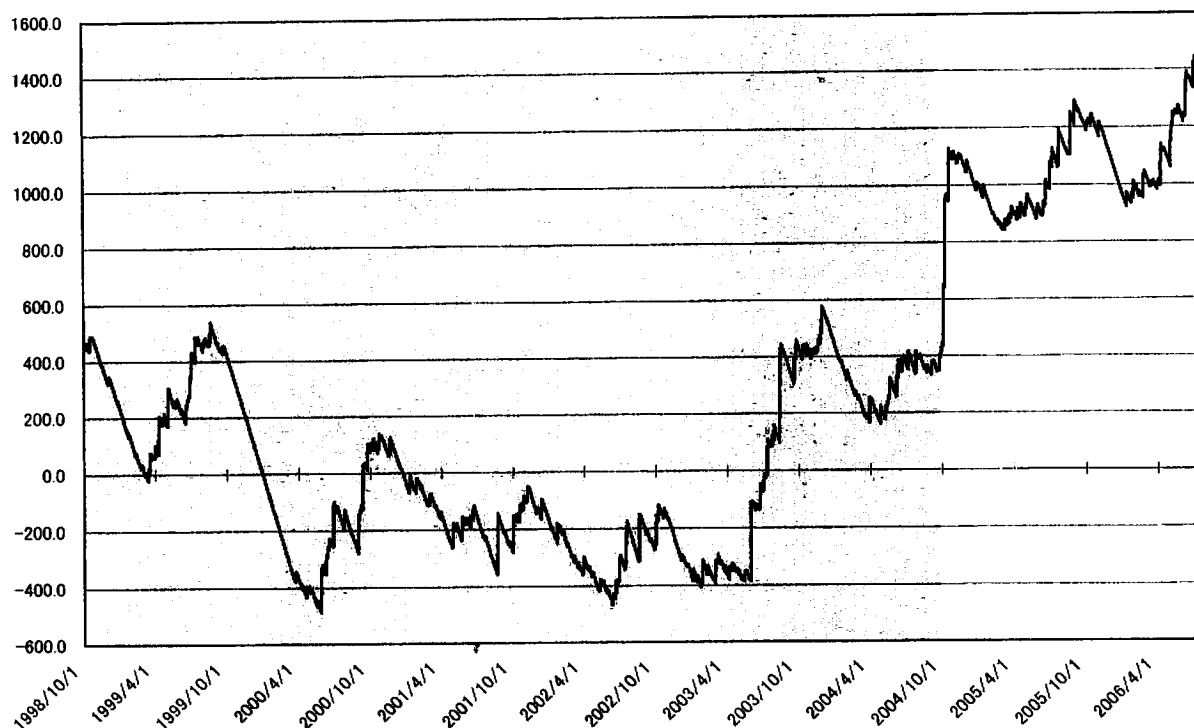
榛原観測井 降雨量の積算からトレンド除去後のグラフ (mm) (1998. 10. 1-2006. 7. 26)
