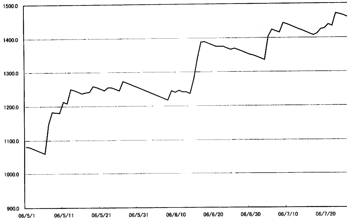
榛原観測井 降雨量の積算からトレンド除去後のグラフ (mm) (2006. 4. 1-2006. 7. 26)
