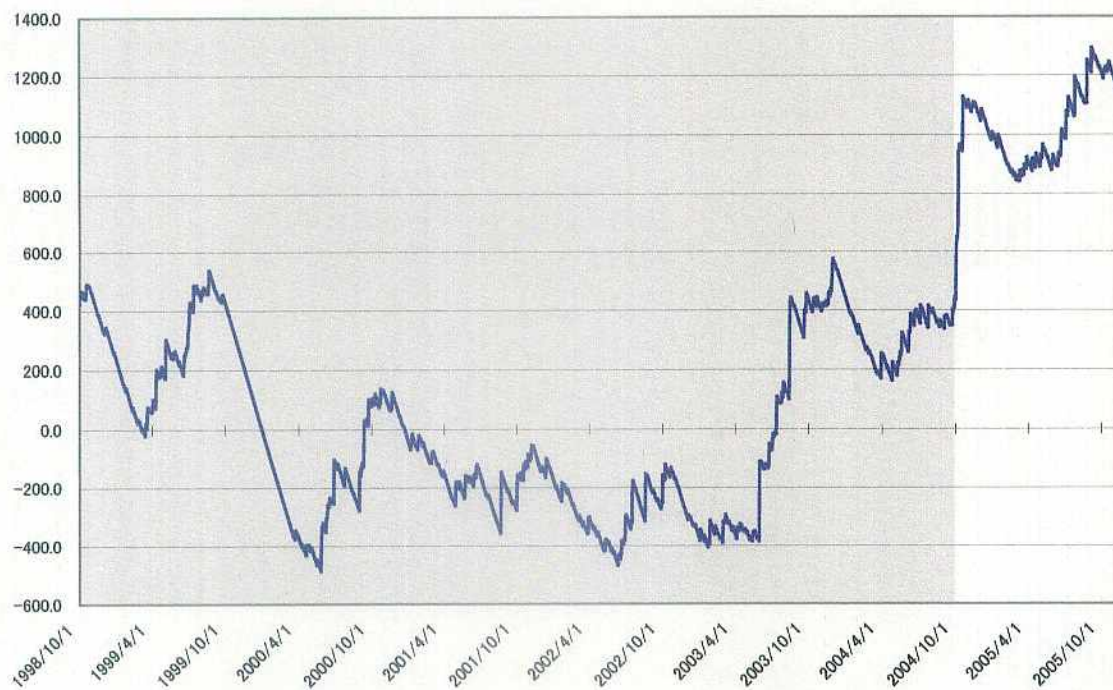
榛原観測井 降雨量の積算からトレンド除去後のグラフ (mm) (1998. 10. 1-2005. 11. 22)
