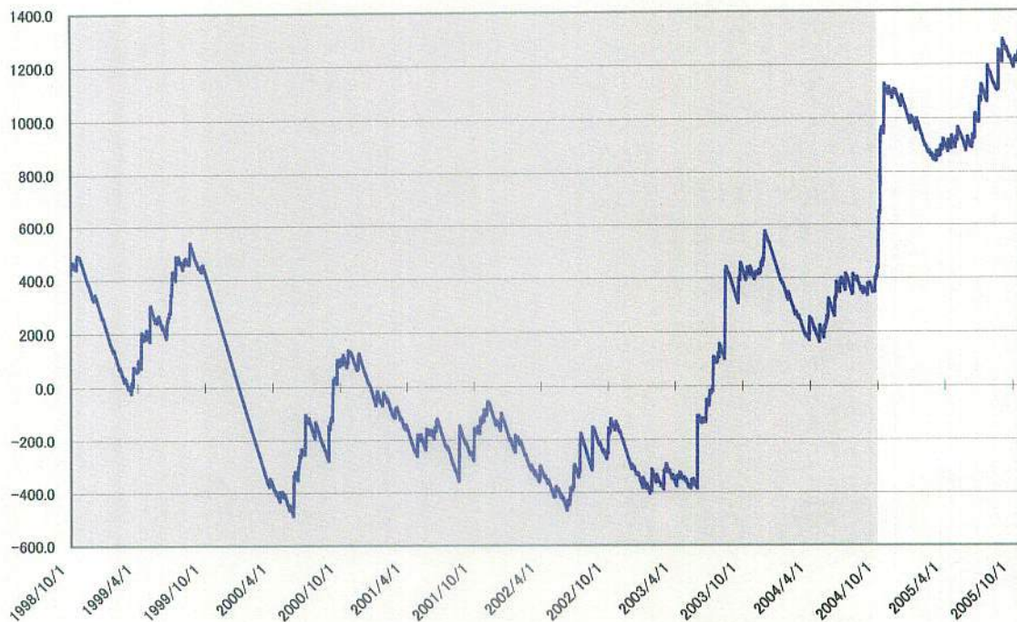
榛原観測井 降雨量の積算からトレンド除去後のグラフ (mm) (1998. 10. 1-2005. 10. 25)
