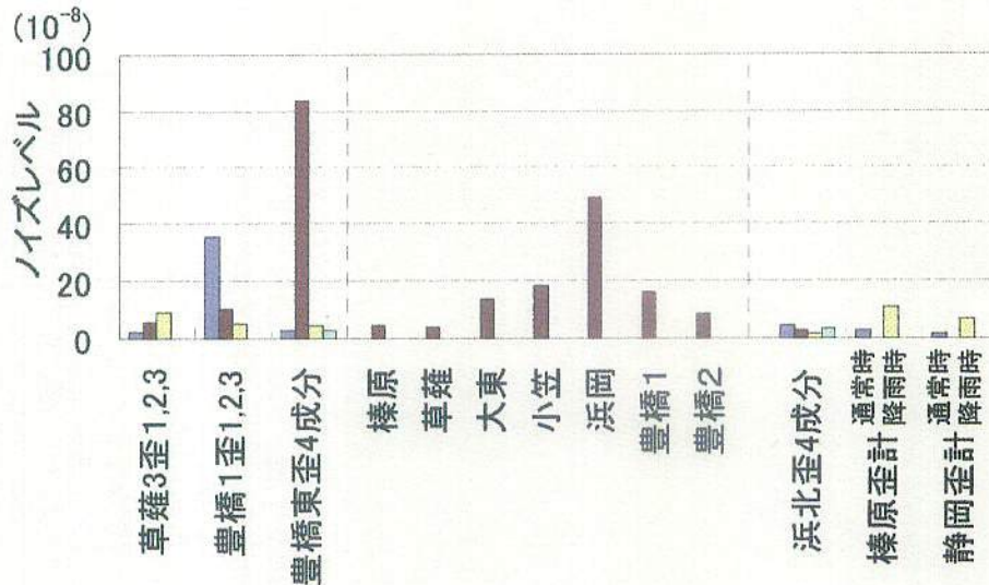
図4 草薙・豊橋1・豊橋東観測井の多成分歪計のノイズレベル(左)。真ん中は産総研地下水位ネットワークのノイズレベル。右は気象庁の多成分歪計と体積歪計のノイズレベル(小林・松森, 1999; 気象庁地震予知情報課、私信)。すべて24時間階差のノイズレベル。
