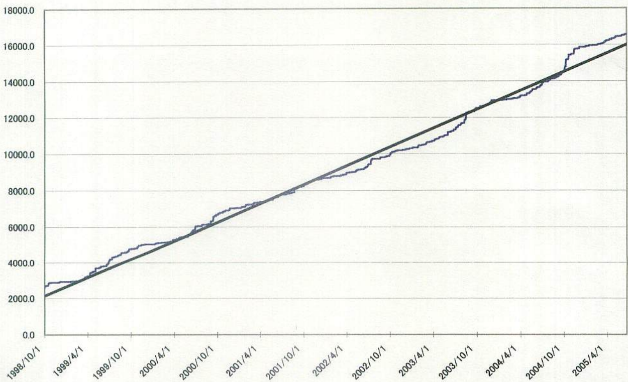
榛原の降雨量の積算グラフ (1998. 10. 1-2005. 6. 21) (mm)
