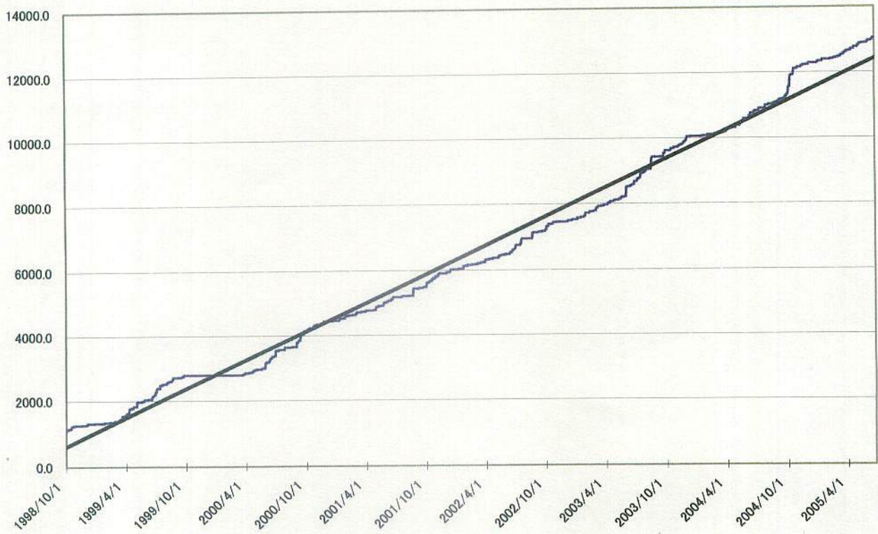
浜岡の降雨量の積算グラフ (1998. 10. 1-2005. 6. 21) (mm)
