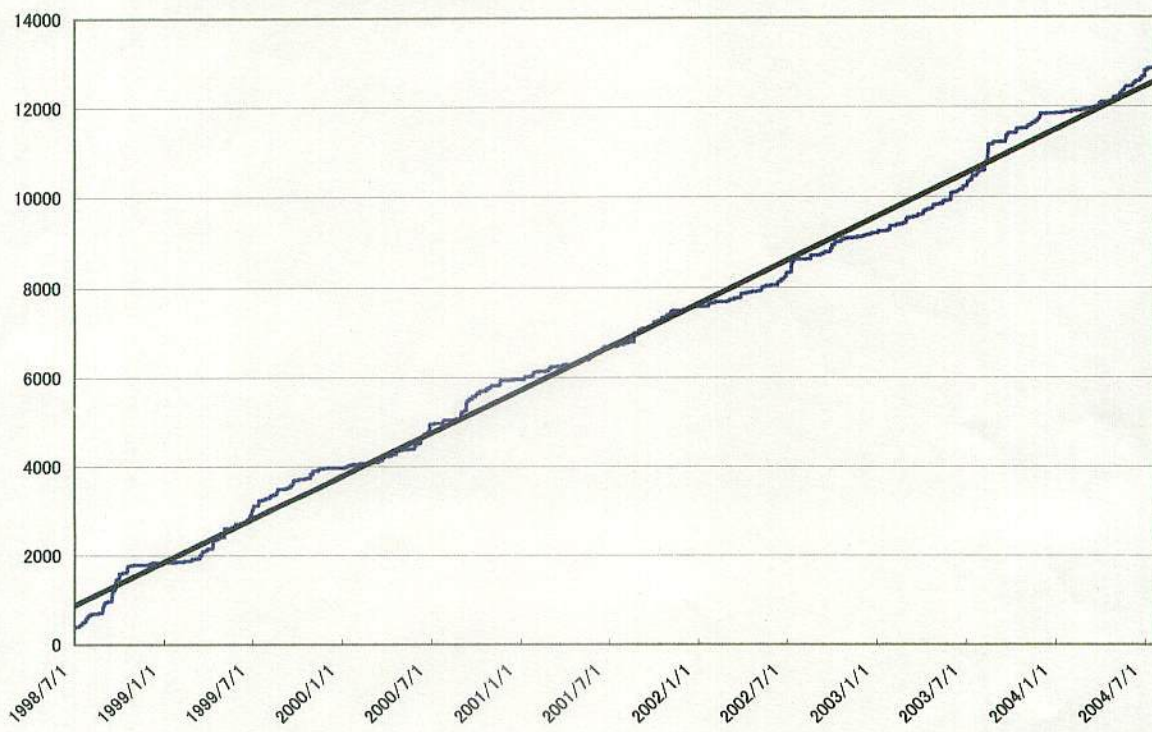
榛原の降雨量の積算グラフ (1998. 7. 1-2004. 7. 21) (mm)
