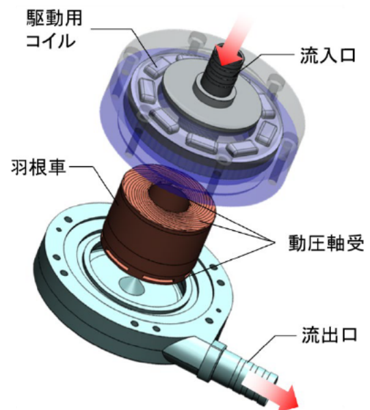
図2 動圧浮上遠心血液ポンプの内部構造
