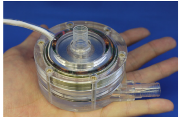
図1 開発した動圧浮上遠心血液ポンプ
