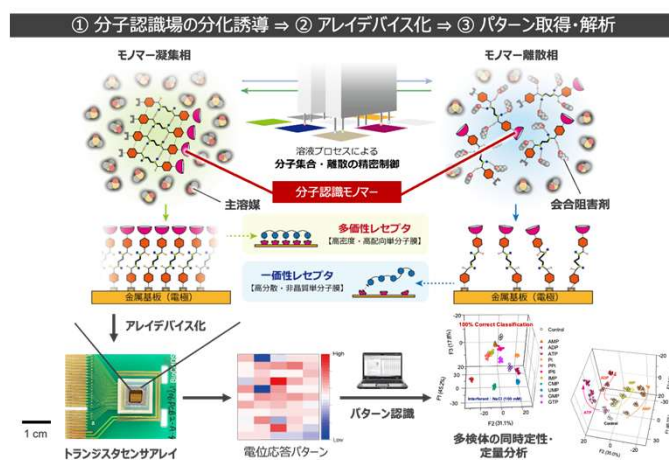
図. 化学センサデバイスの概要
