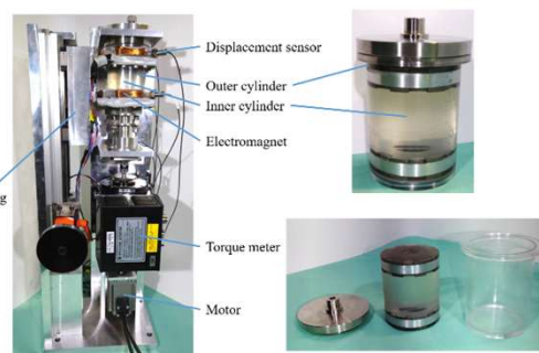
図2 血流を模擬したせん断負荷装置 (東京科学大学との共同研究)
