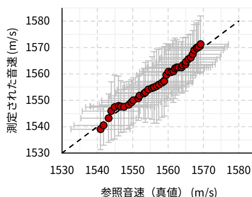
図2 肝臓（摘出）の音速測定結果
