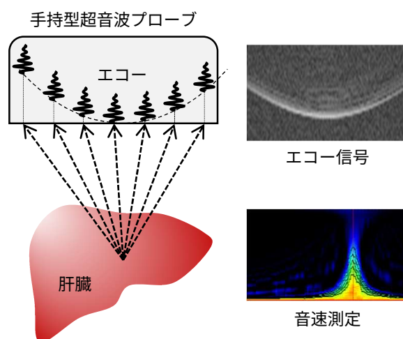
図1 肝臓を対象とした音速測定
