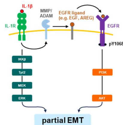
図2 pEMT誘導に関わる新規シグナル経路
