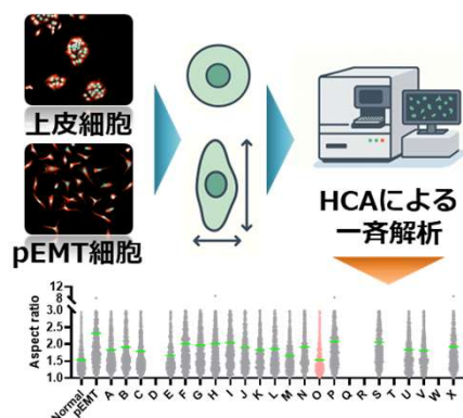
図1 形態変化を指標としたスクリーニング法
