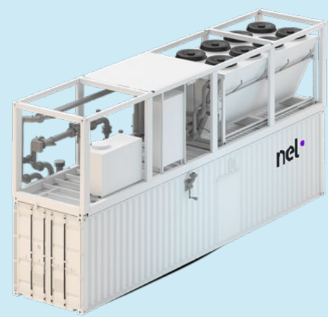
Nel社製水電解装置（PEM型）
