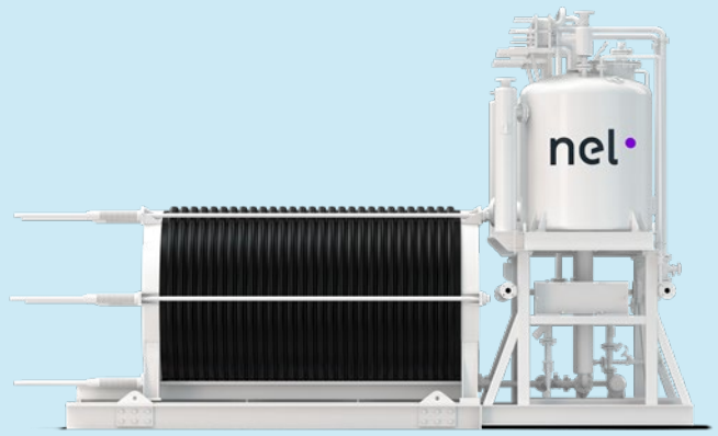
Nel社製水電解装置（アルカリ型）
