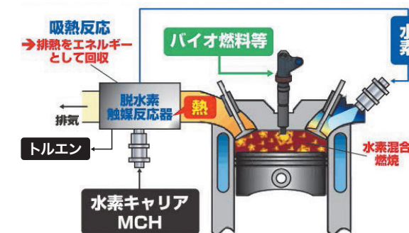
エンジン排熱回収型脱水素反応システム
