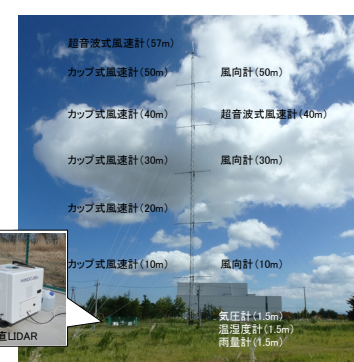
ライダー風況アセスメントの実証試験
