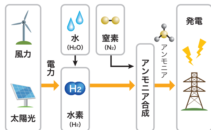
アンモニア発電のしくみ
