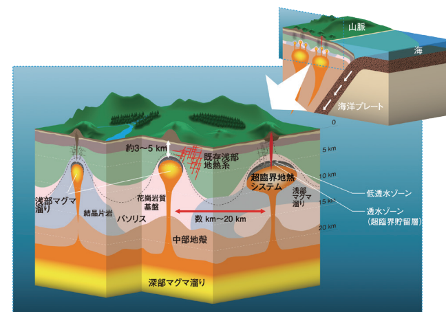
超臨界地熱システムの概念
