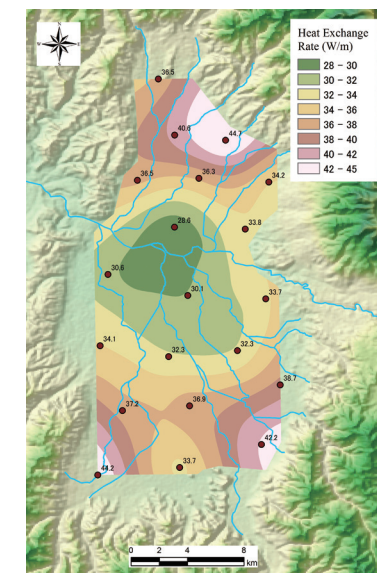
会津盆地における地中熱ポテンシャルマップ
