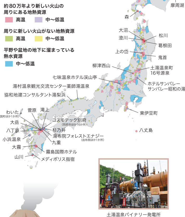
土湯温泉バイナリー発電所
