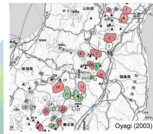
東北地方で50以上の古火山・カルデラが存在します。 古いカルデラの分布 (Oyagi, 2003)
