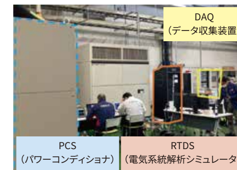
DAQ (データ収集装置) PCS (パワーコンディショナ) RTDS (電気系統解析シミュレータ)
