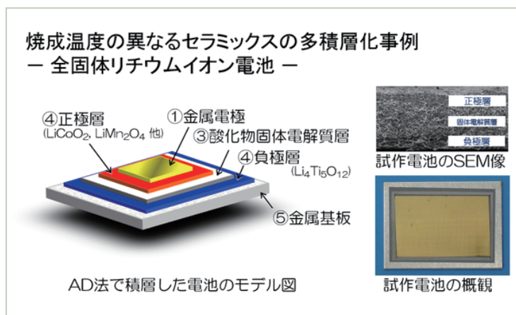
全固体リチウム電池試作例
