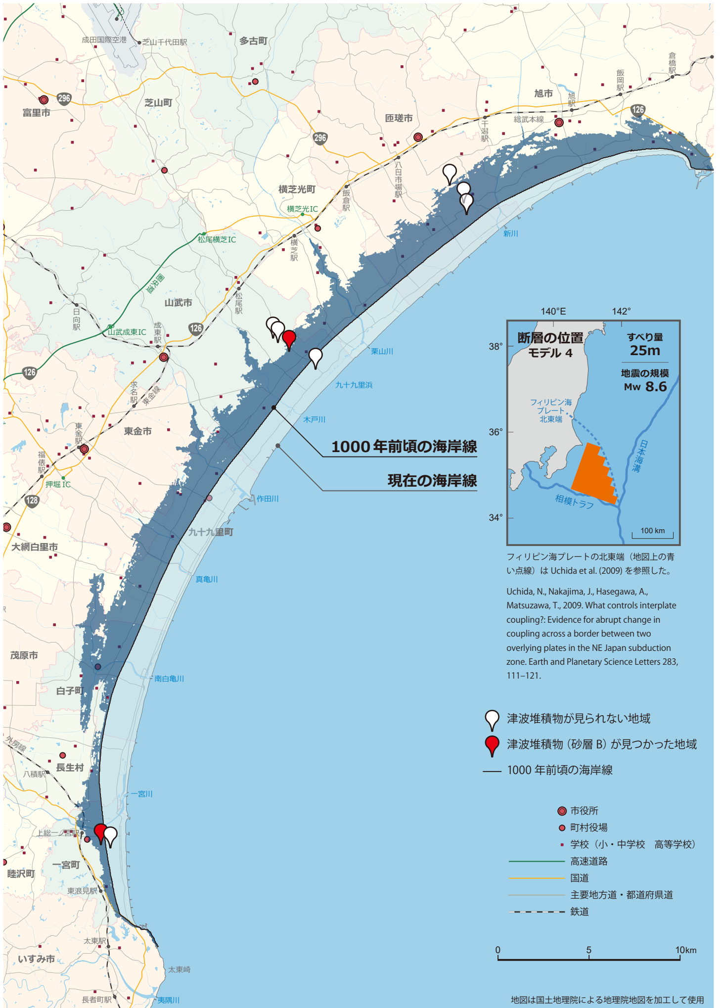
房総半島東方沖で約1000年前に発生した巨大津波の浸水域 (モデル 4)
