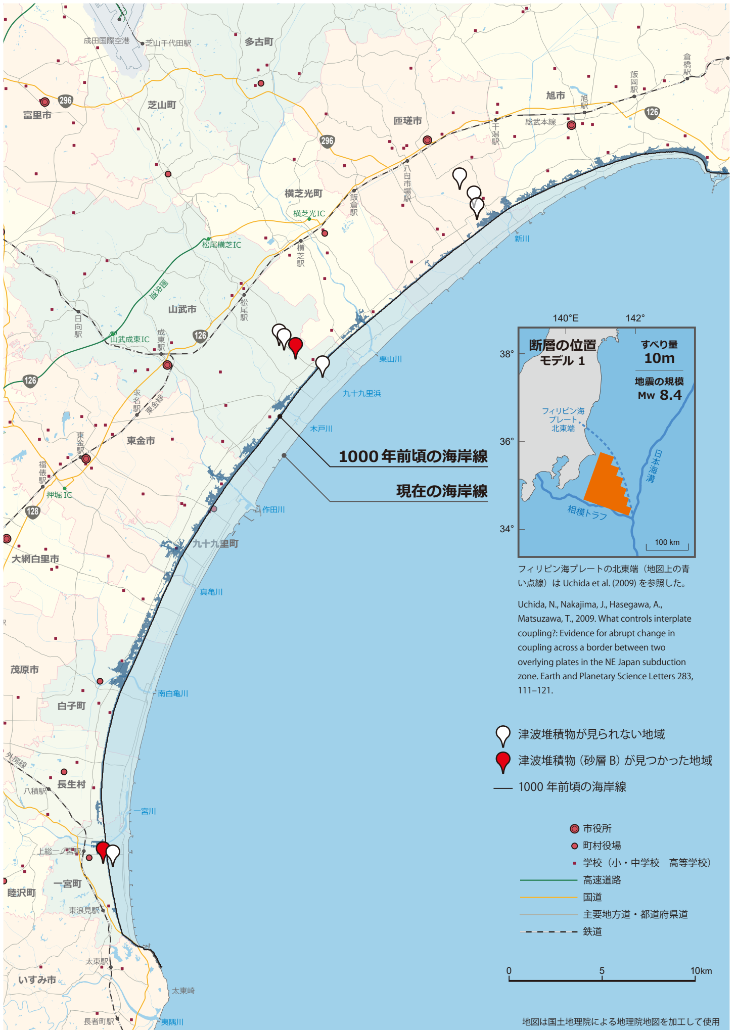
房総半島東方沖で約1000年前に発生した巨大津波の浸水域 (モデル 1)
